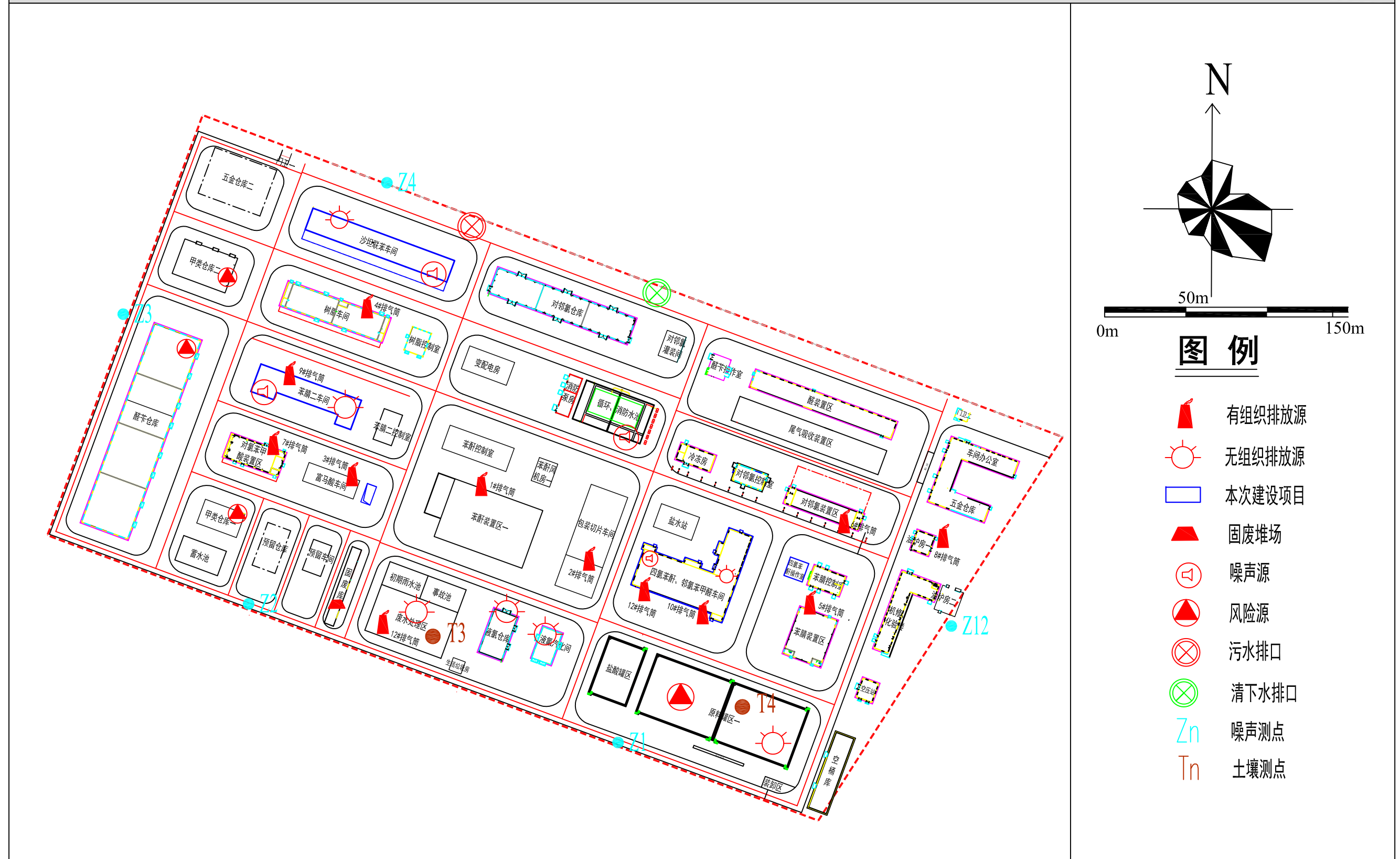
附图二 项目平面布置图
