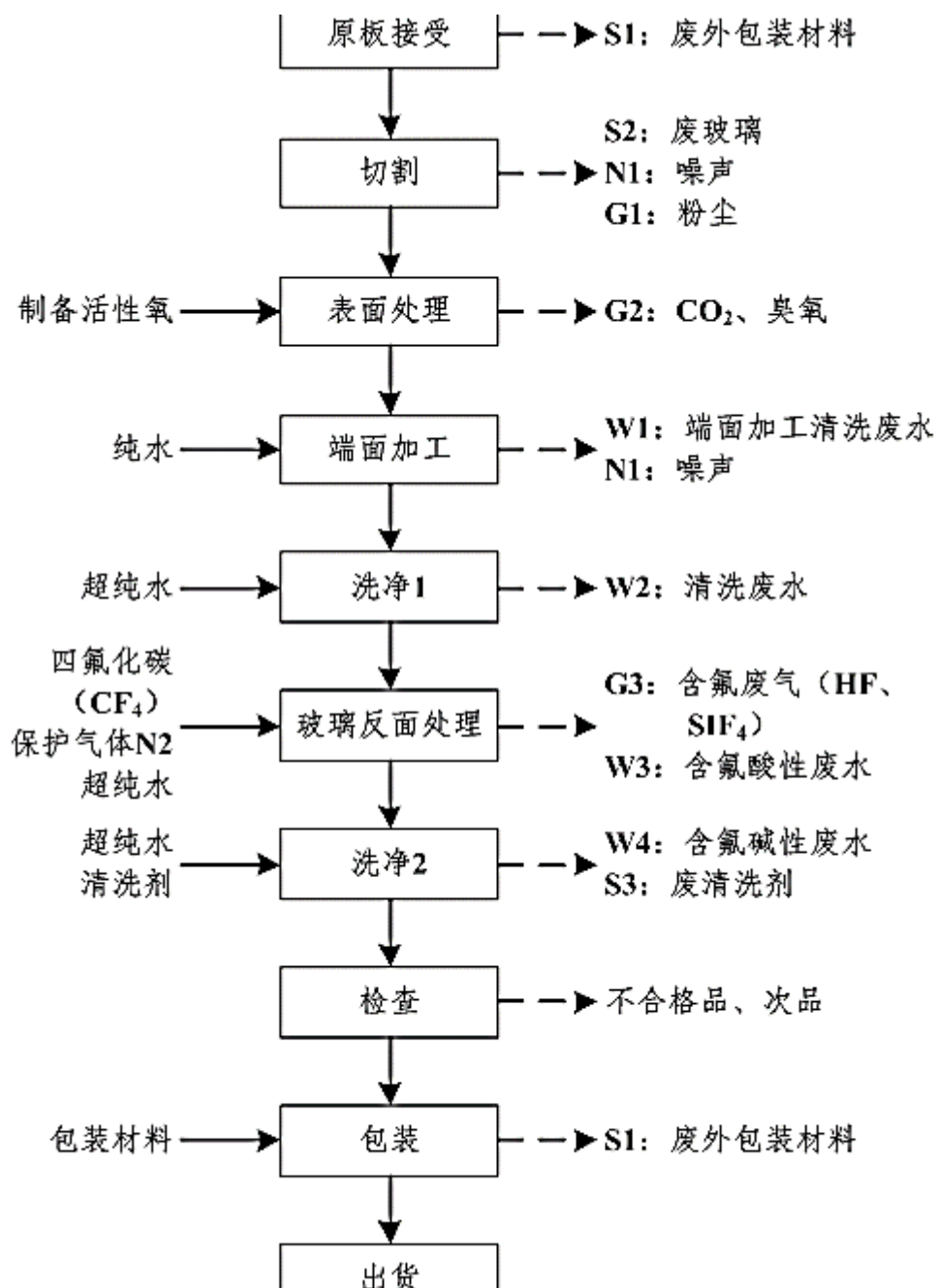
图 3-5 生产工艺及产污流程图
