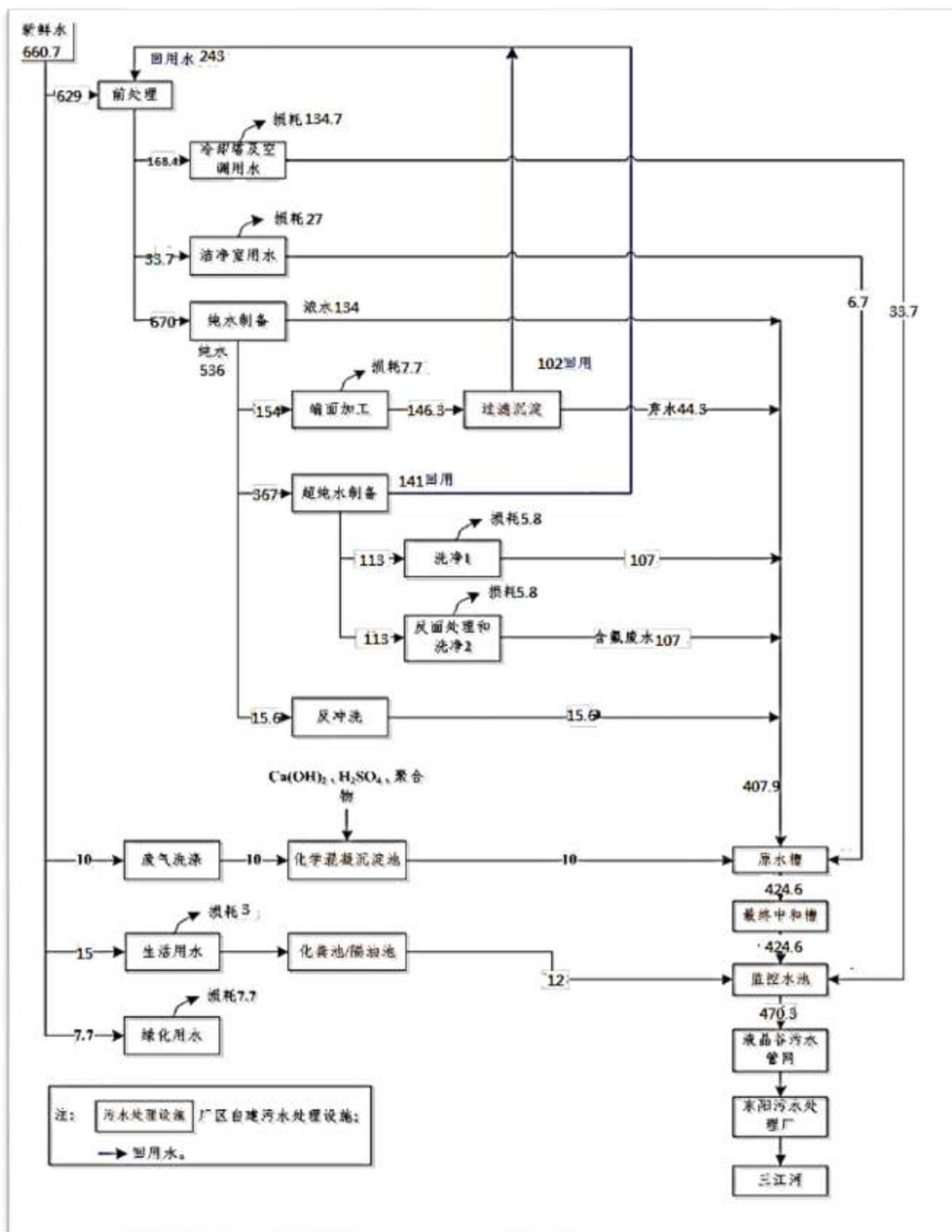
图 3-4 全厂实际水平衡图 (m³/d)
