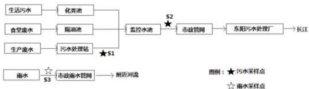
图 4-3 全厂废水及雨水流向图
