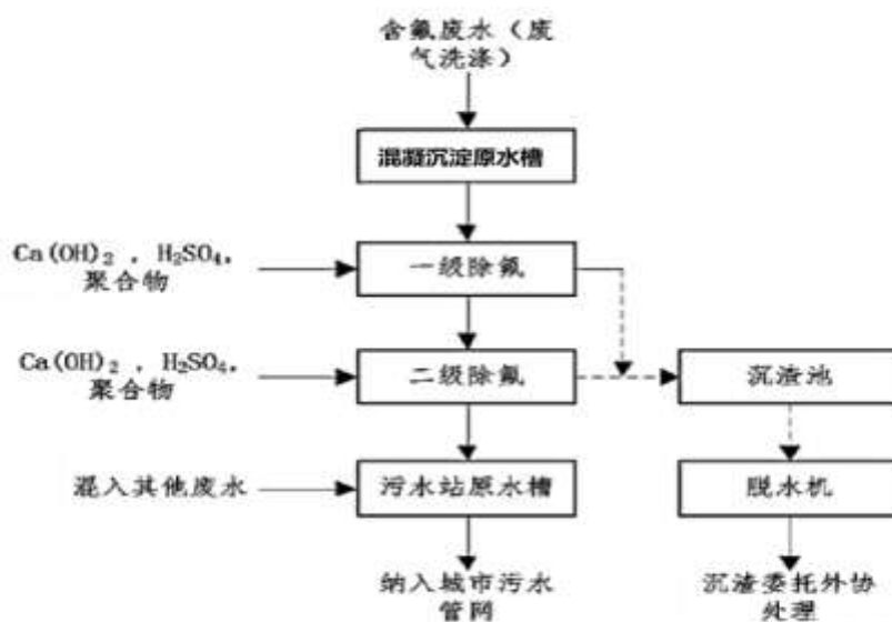
图 4-1 污水处理工艺流程图
