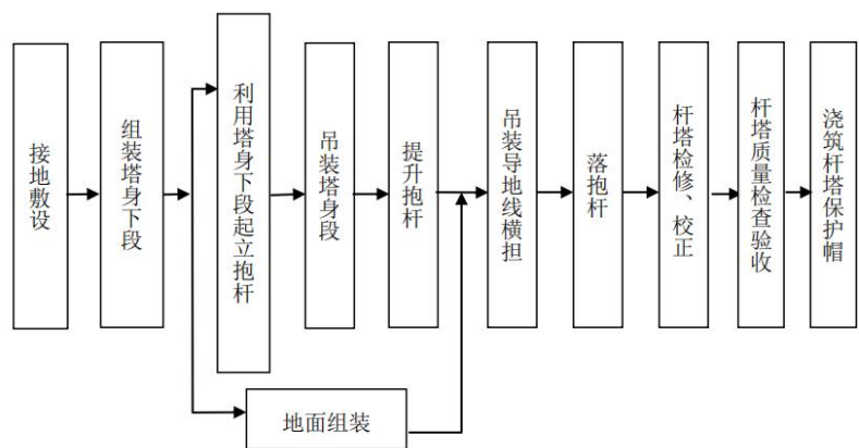
图 3.1 铁塔组立及接地工程施工流程图
