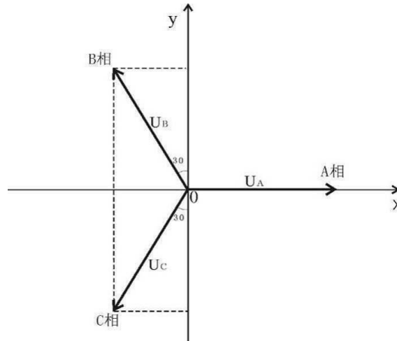
图 6.1 对地电压计算图
