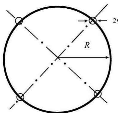
图 6.3 等效半径计算图
