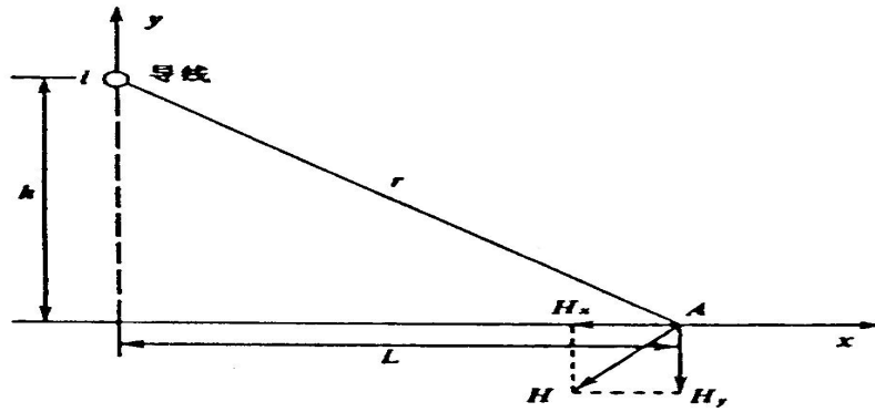
图6.4 磁场向量图
