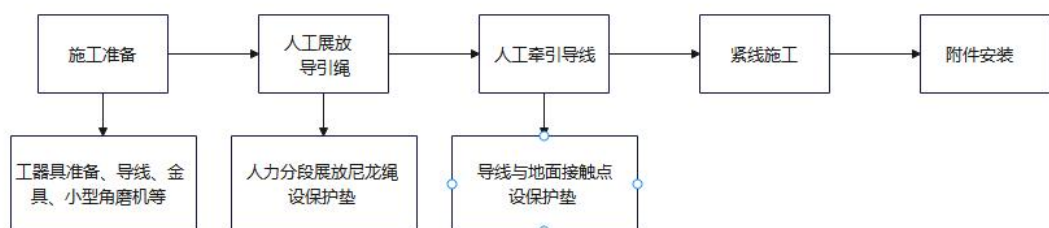
图 3.2 架线施工流程图
