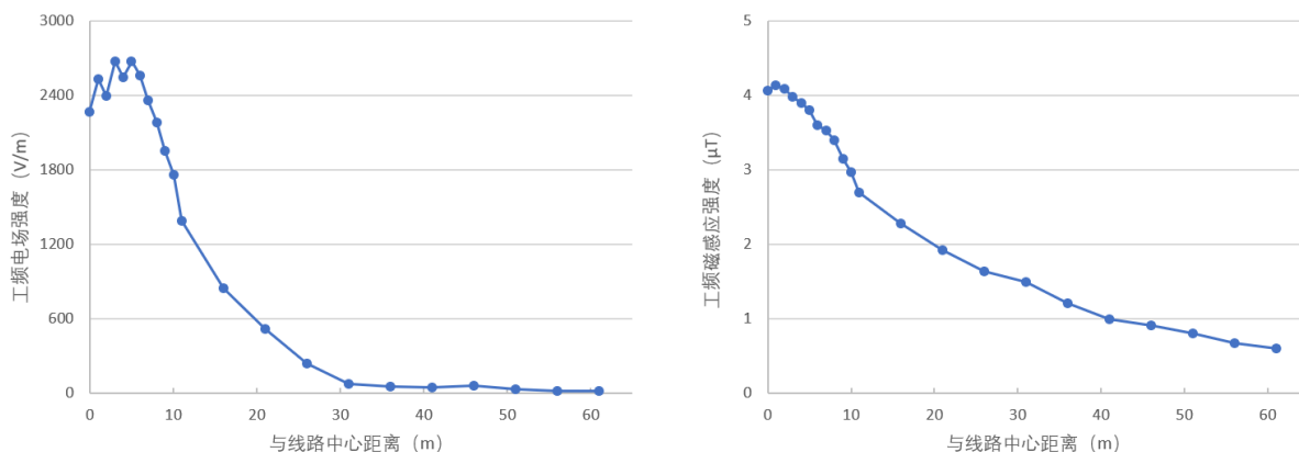
图 6-2 类比监测线路工频电场、工频磁场分布示意图
