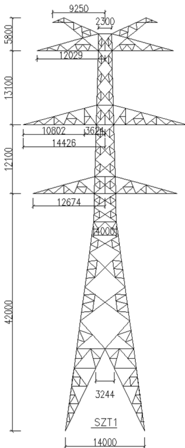
图 6-5 本项目同塔双回线路模式计算典型杆塔
