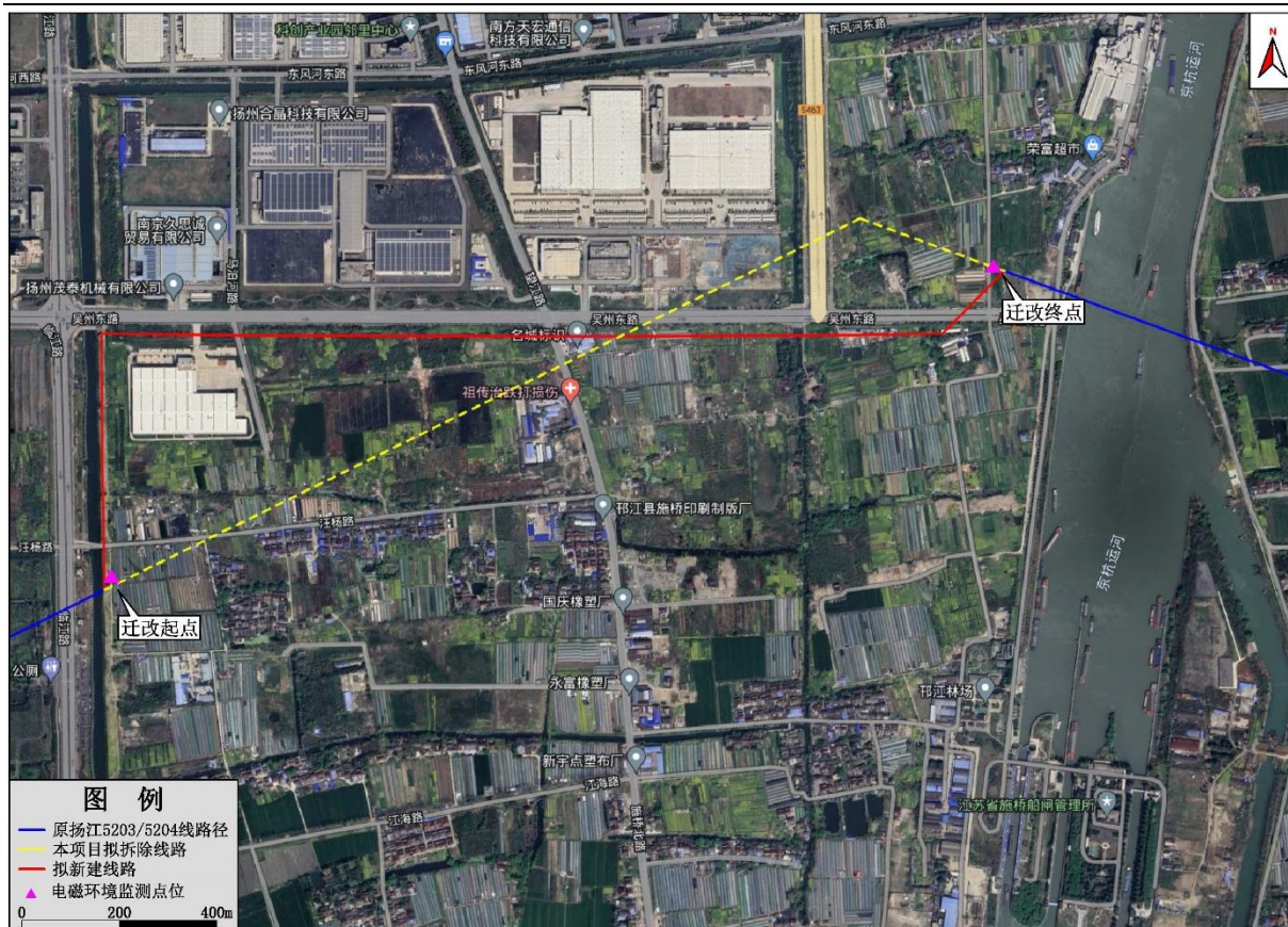
图 4-1 迁改线路起点、终点处监测点位示意图
