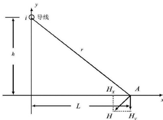
图 6-3 磁场向量图
