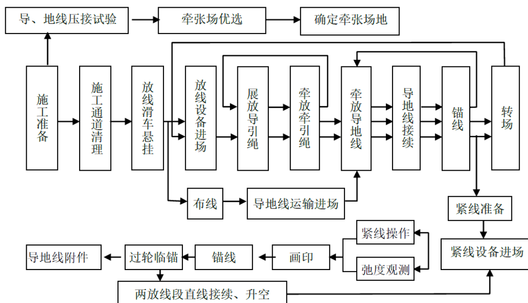
图 3-2 架线施工流程图
