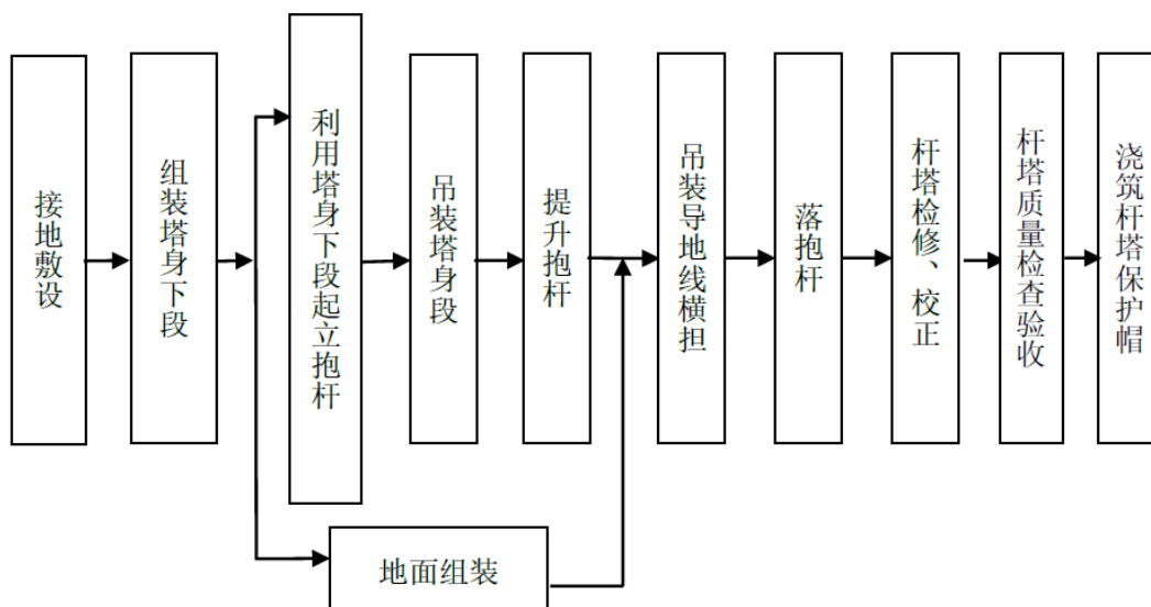
图 3-1 杆塔组立及接地工程施工流程图
