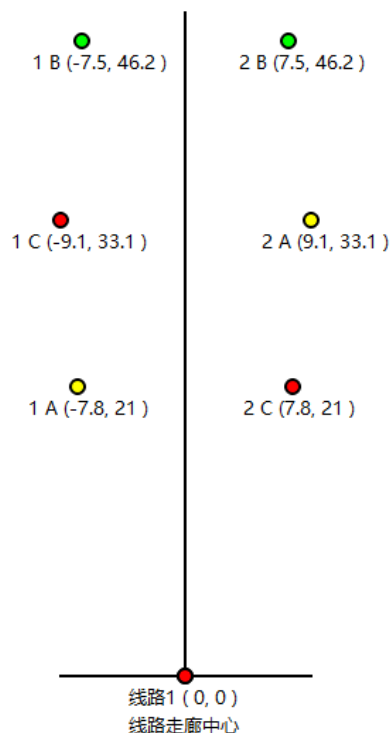
图 6-4 计算模型示意图
