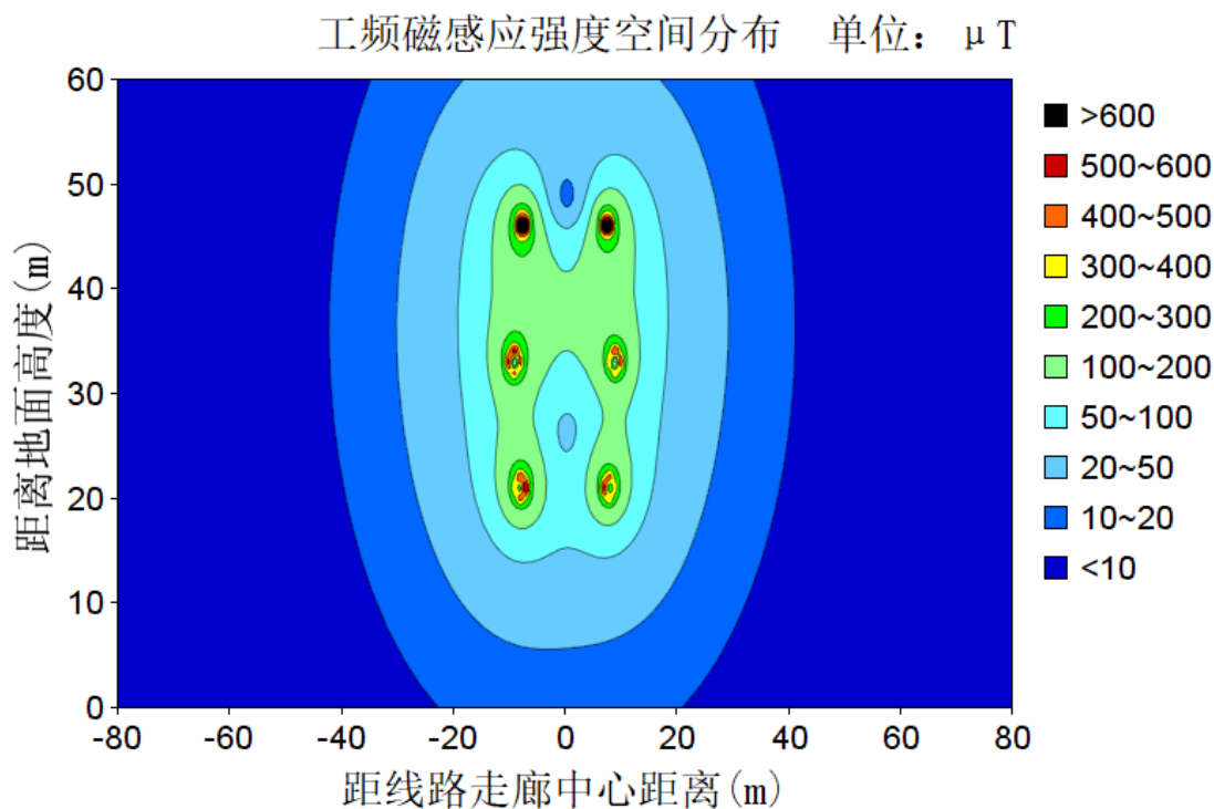
图 6-9 500kV 同塔双回线路工频磁感应强度等值线图 (导线高度 21m)
