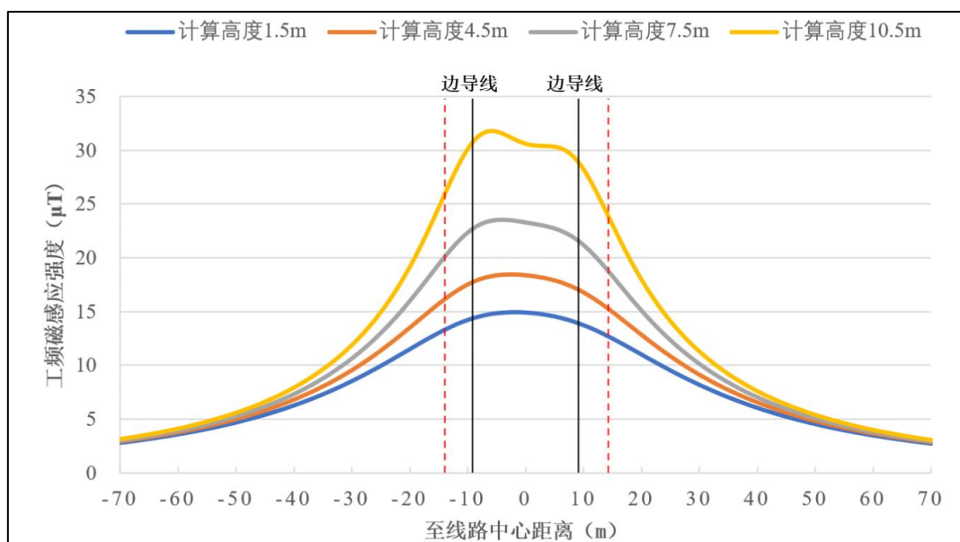
图 6-8 500kV 同塔双回线路不同计算高度工频磁感应强度预测结果 (线高 21m)
