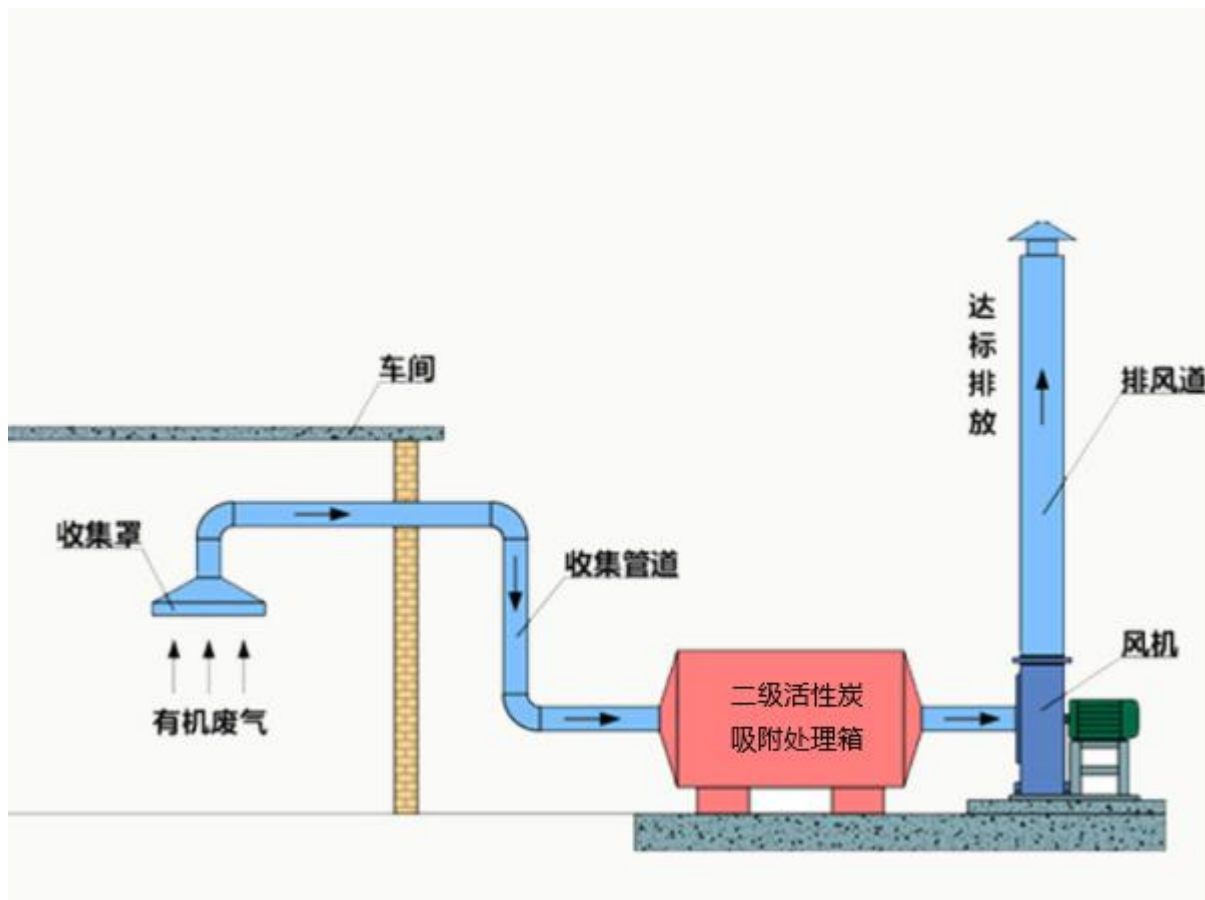
图4-1 二级活性炭吸附装置工艺流程图
