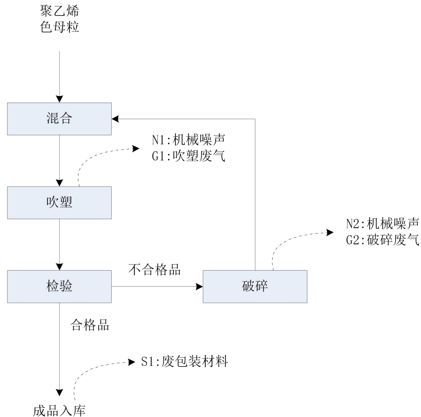
图2-2 塑料瓶生产工艺流程图及产污环节图
