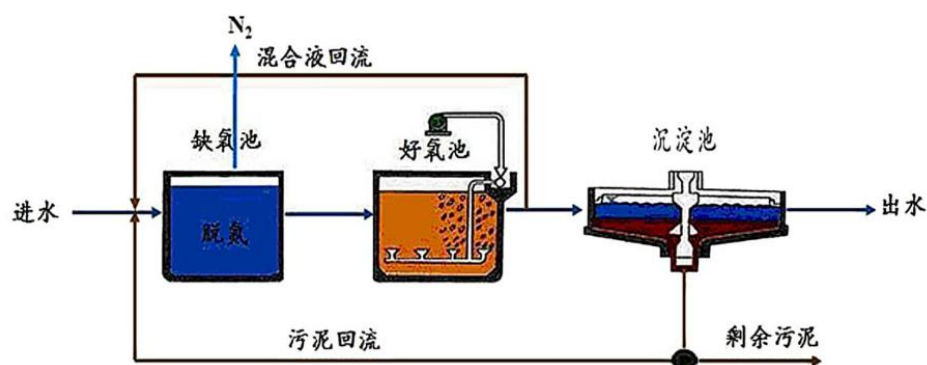
图4-4 红山污水处理厂污水处理工艺流程
