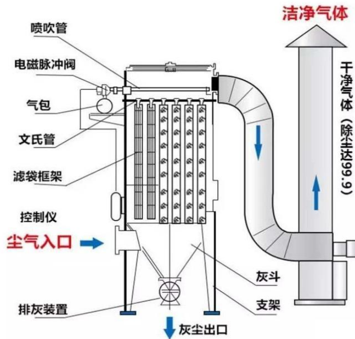
图4-3 布袋除尘器工艺流程图
