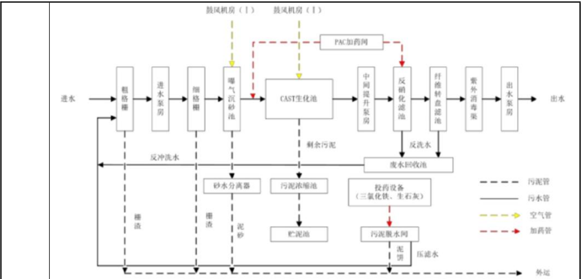
图 4-1 六合区污水处理厂工艺流程图
