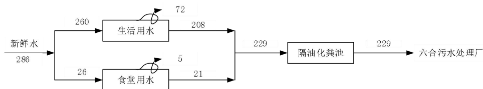
图 2-1 建设项目实施后全厂水平衡图 单位：t/a
