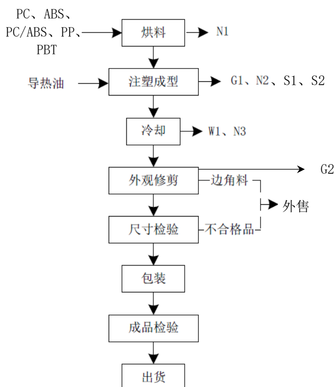
图 5-1 工艺流程图
