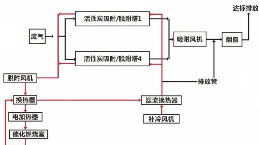
图 7-1 催化燃烧装置原理图
