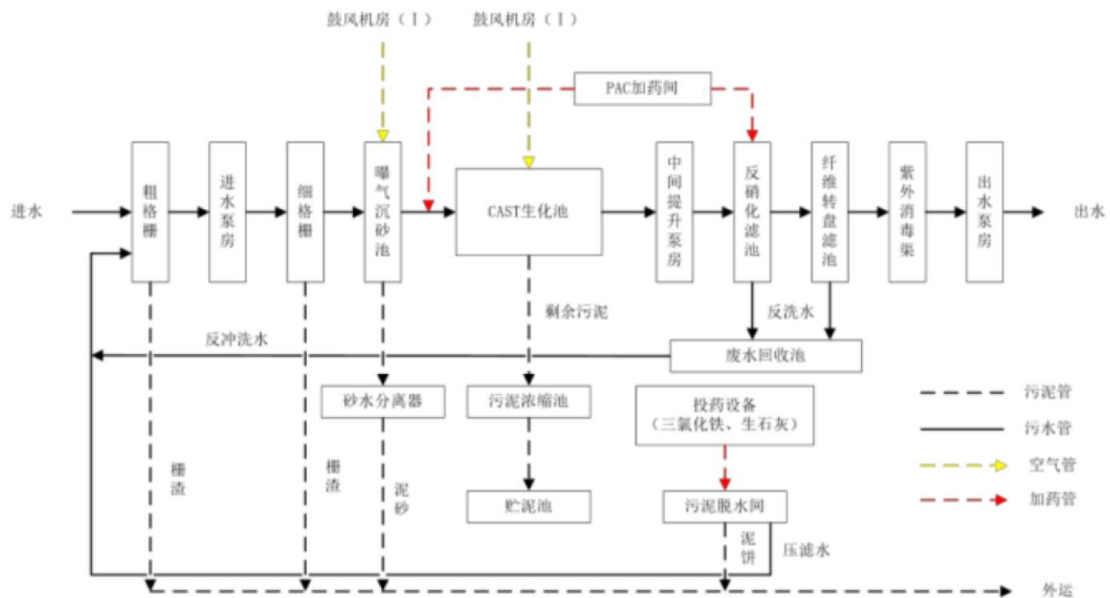
图7-2 六合区污水厂工艺流程图
