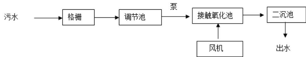
图 6.3-4 锡张高速沿线地埋式污水处理装置工艺流程图
