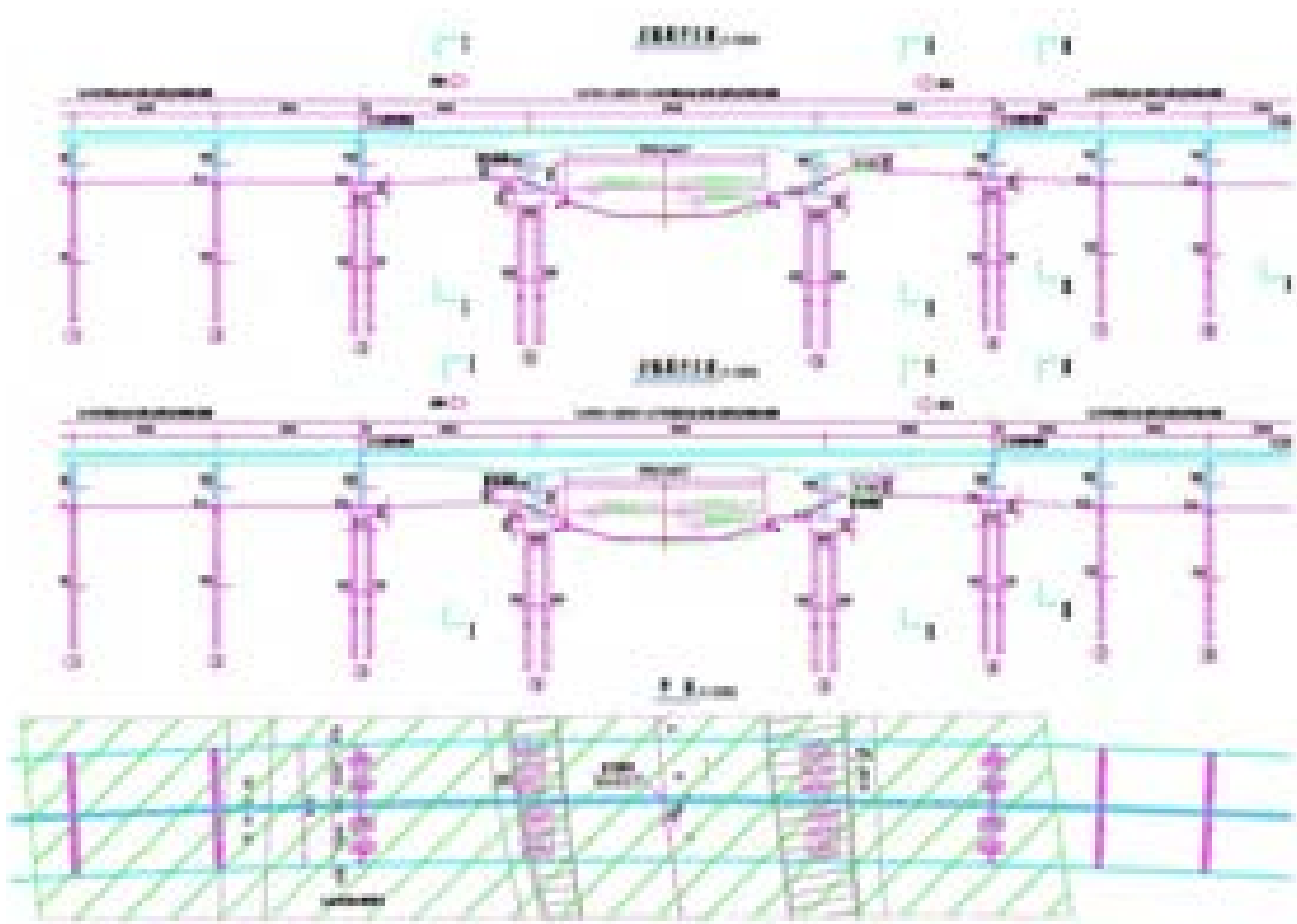
图 2.3-2 九曲河桥型布置图
