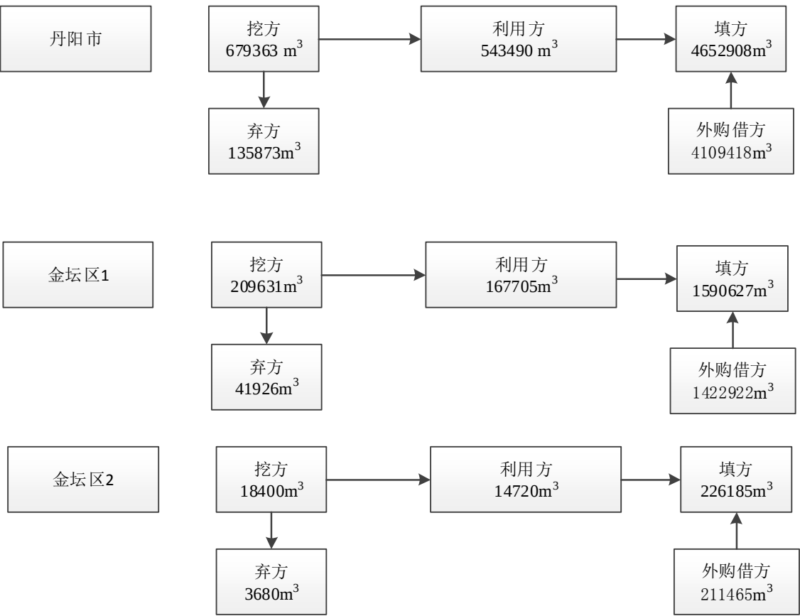
图 2.3-5 土石方平衡图
