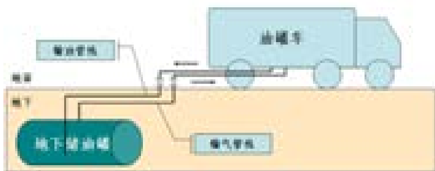
图 6.3-1 卸油油气回收系统示意图
