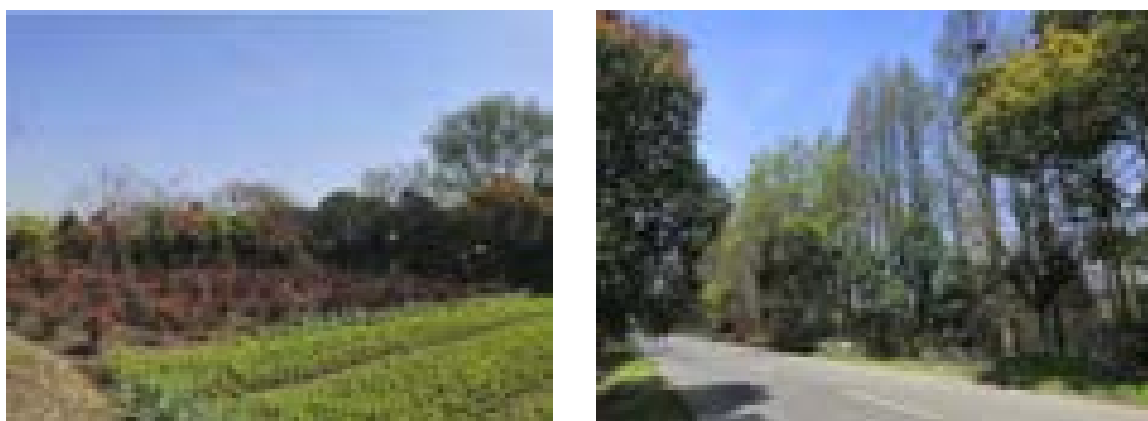
图 3.2-5 现状自然生态系统 (a)
