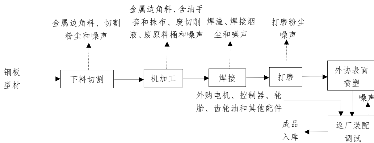
图 6.1 项目生产工艺流程及产污环节图
