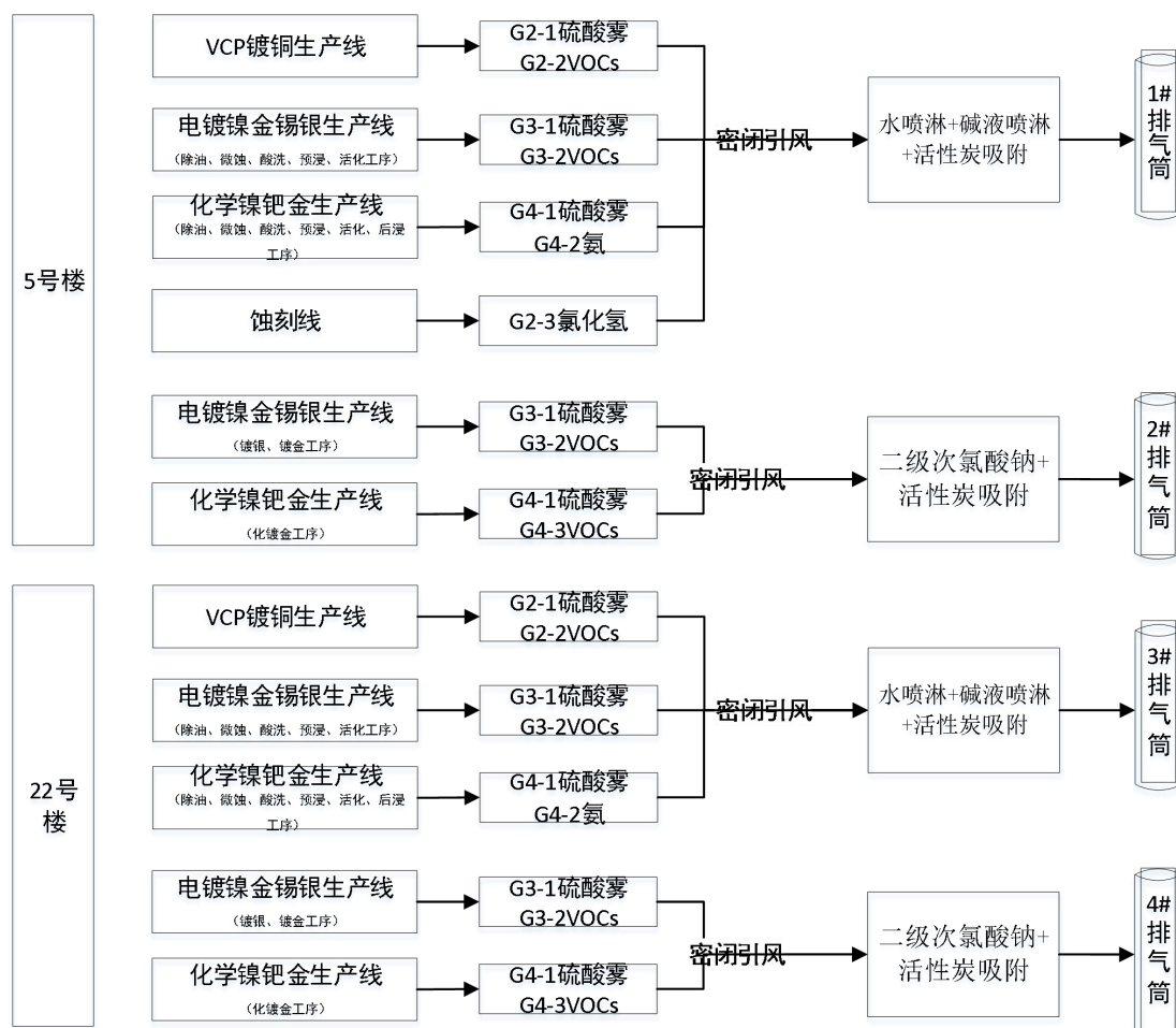
图 6.1.1-1 废气收集系统示意图
