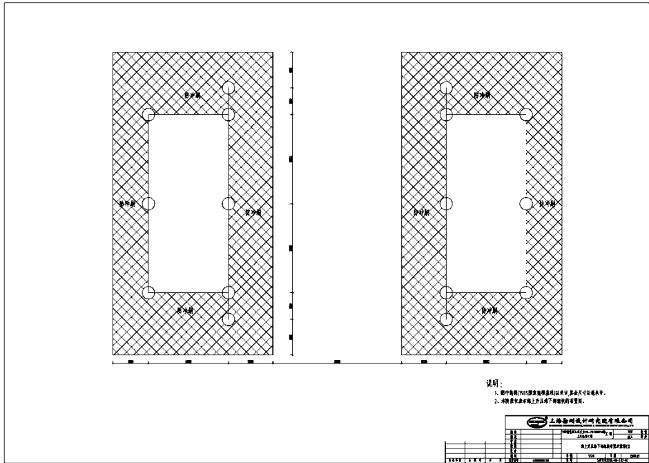
图 3.3-10 海上换流站基础防冲刷保护
