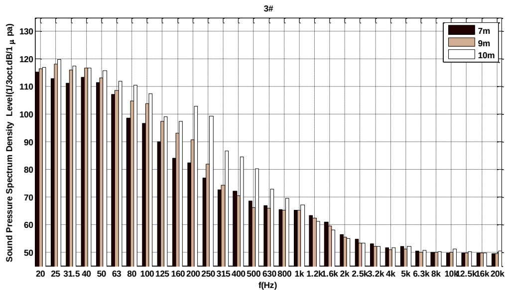
图 6.8-8 3#测点不同水深声压功率密度谱比较（1/3oct. 声压谱级）
