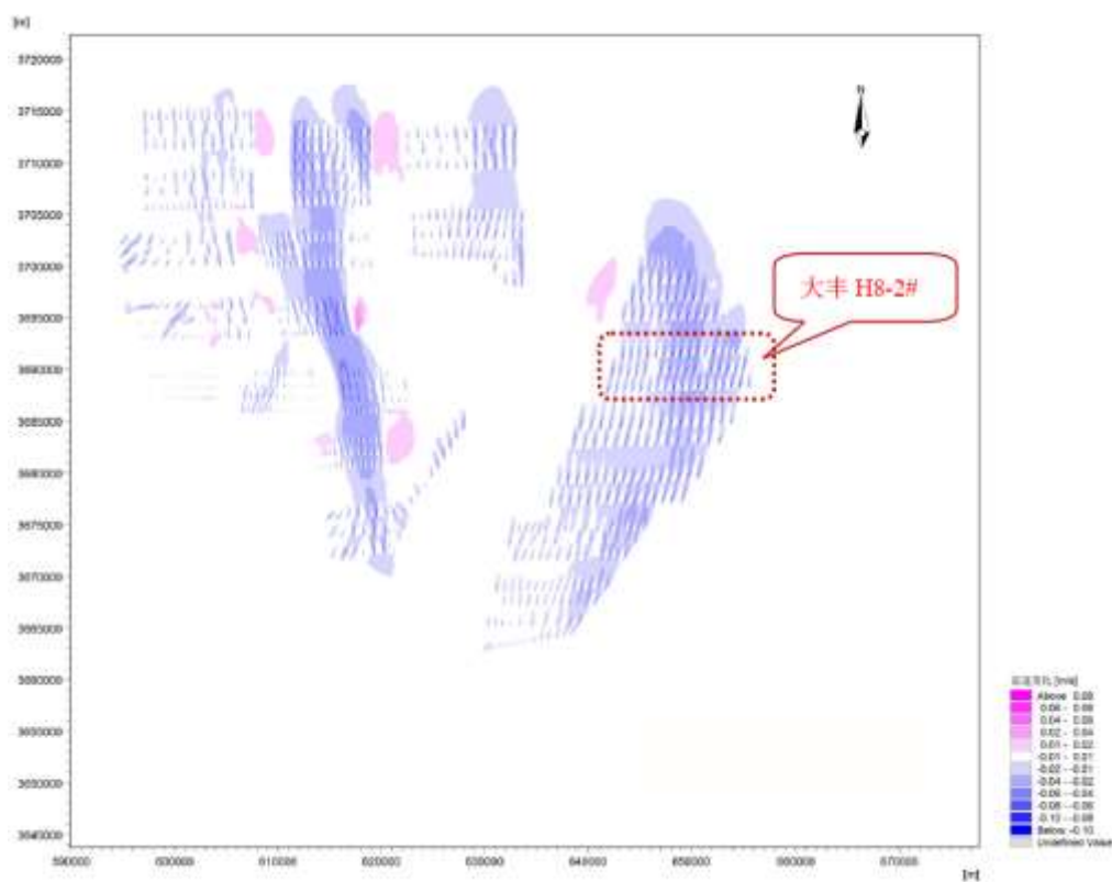
图 7.1-21 工程建设前后大潮落急时刻流速变化图
