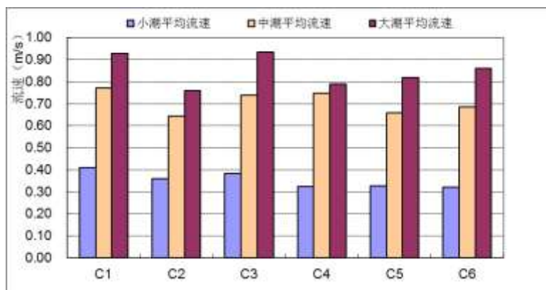
图 6.1-4 夏季测验期间各测站流速对比
