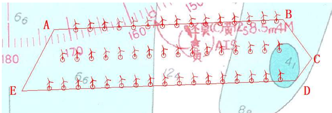
图 12.5-3 方案三风机布置图
