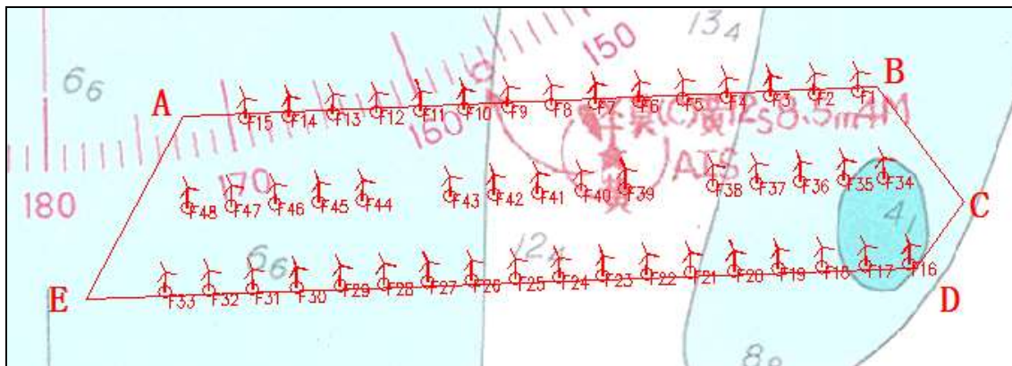
图 12.5-4 江苏大丰 H8-2 海上风电场最终风机布置图
