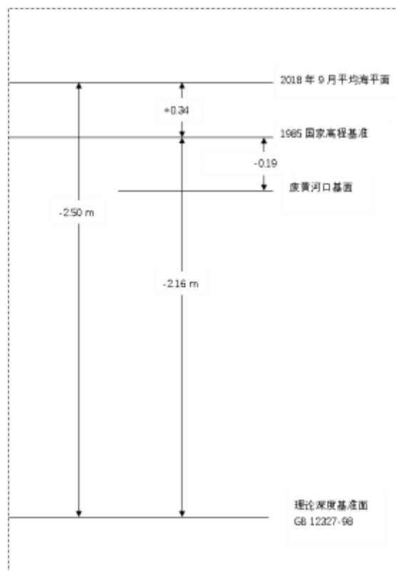
图 6.1-3 风电场区水域基准面关系
