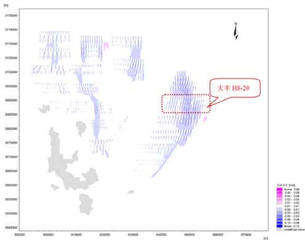
图 7.1-20 工程建设前后大潮涨急时刻流速变化图
