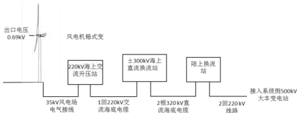
图 3.3-1 风电场工艺流程图
