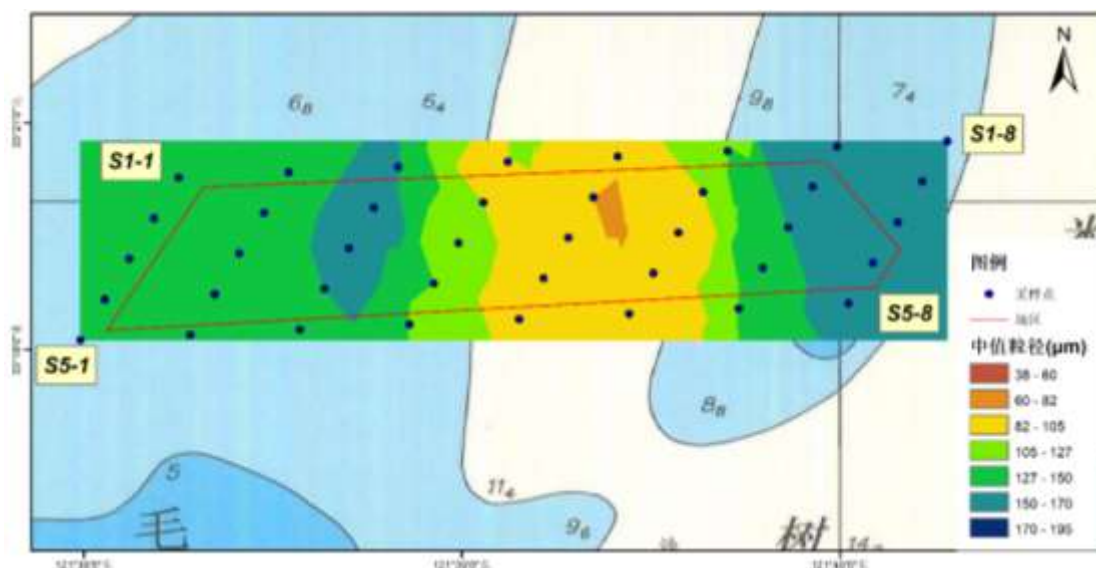
图 6.1-10 表层沉积物中值粒径分布示意图
