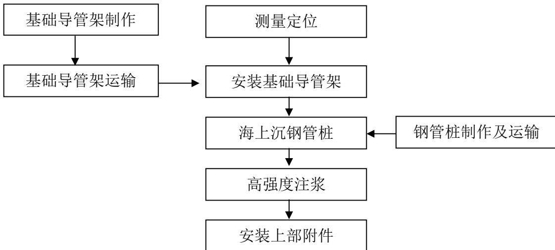
图 3.5-5 海上升压平台基础施工流程图
