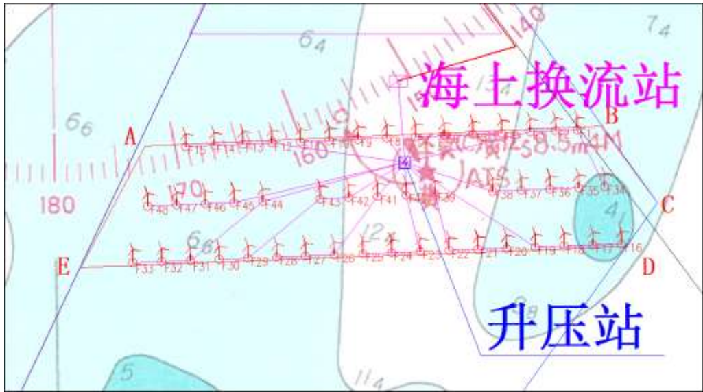
图 3.3-2 风电场风机布置示意图
