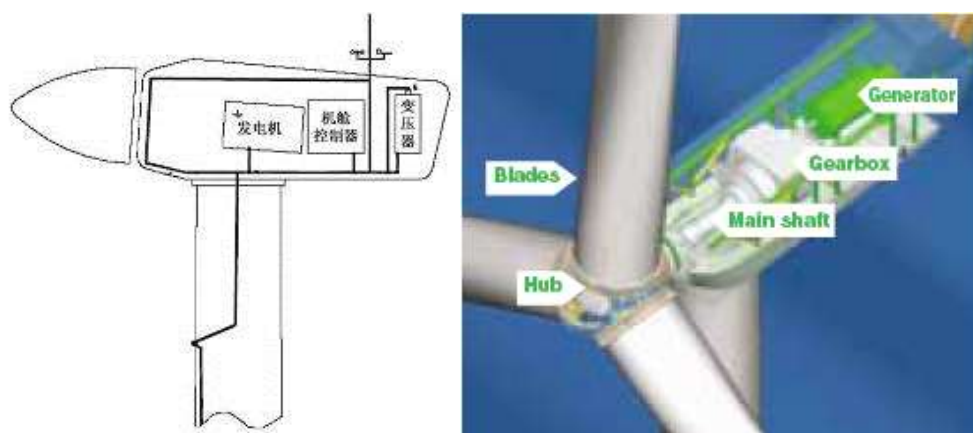
图 3.3-3 风机机舱结构示意图
