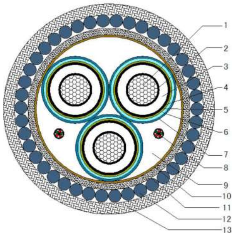
1.阻水导体 2.半导电尼龙带+导体屏蔽 3.绝缘 4.绝缘屏蔽 5. 半导电电阻带 6.铅套 7.半导电 PE 护套 8.光缆单元 9.PP 填充 10.成缆包带 11.聚丙烯绳内衬层 12. 镀锌钢丝 13. 聚丙烯绳纤维外被
