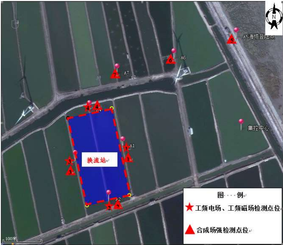
图 6.9-1 电磁环境现状检测点位示意图
