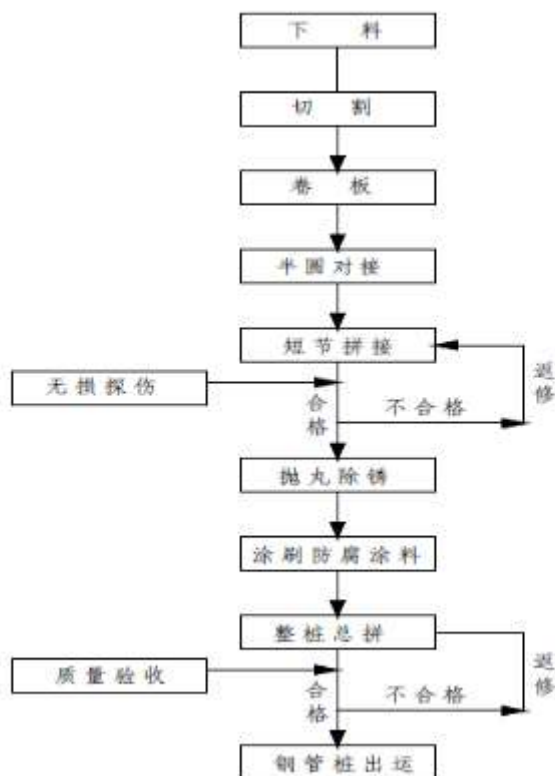
图 3.5-3 钢管桩制作工艺流程图
