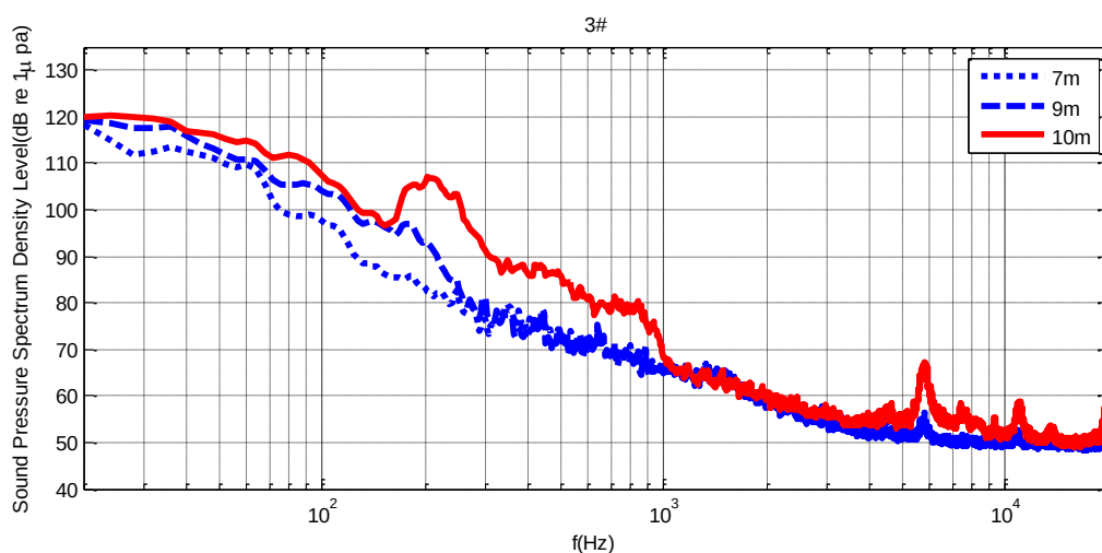
图 6.8-7 3#测点不同水深声压功率密度谱比较（窄带频率谱）
