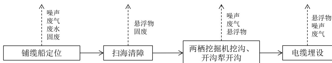
图 4.1-2 电缆主要施工工序及产污环节
