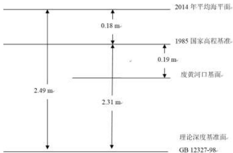
图 5.1-7 基面关系示意图
