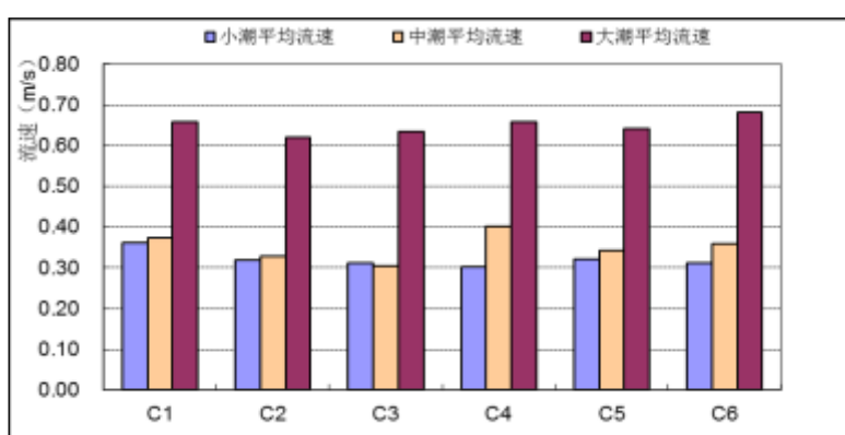
图 6.1-5 冬季测验期间各测站流速对比
