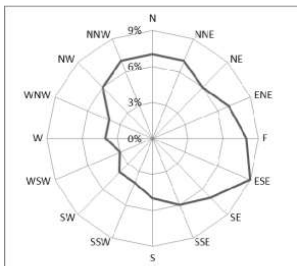
图 5.1-4 大丰气象站多年风向玫瑰图
