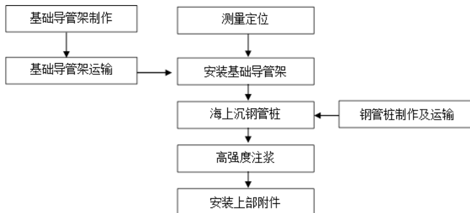
图 3.5-6 海上换流站基础施工流程图
