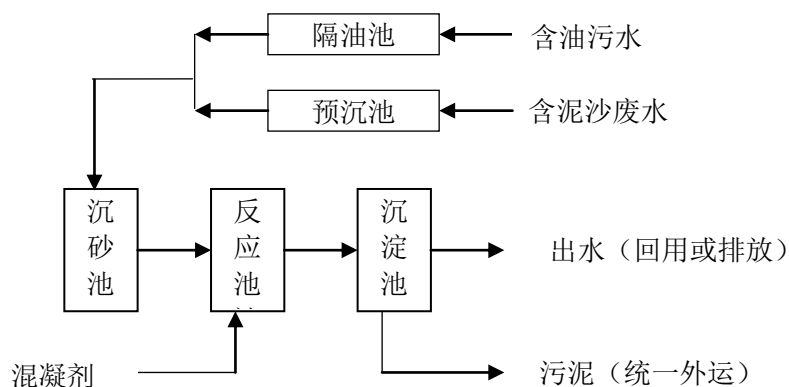
图 10.2-1 施工废水处理流程图
