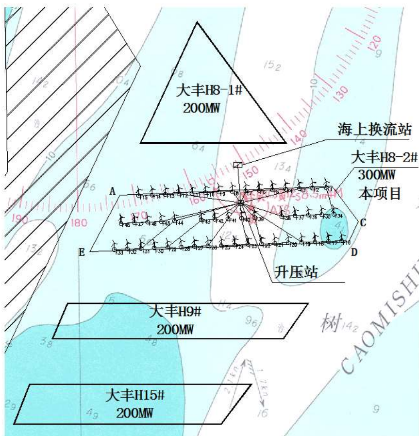
图 3.3-4 海上升压站及换流站布置方案图
