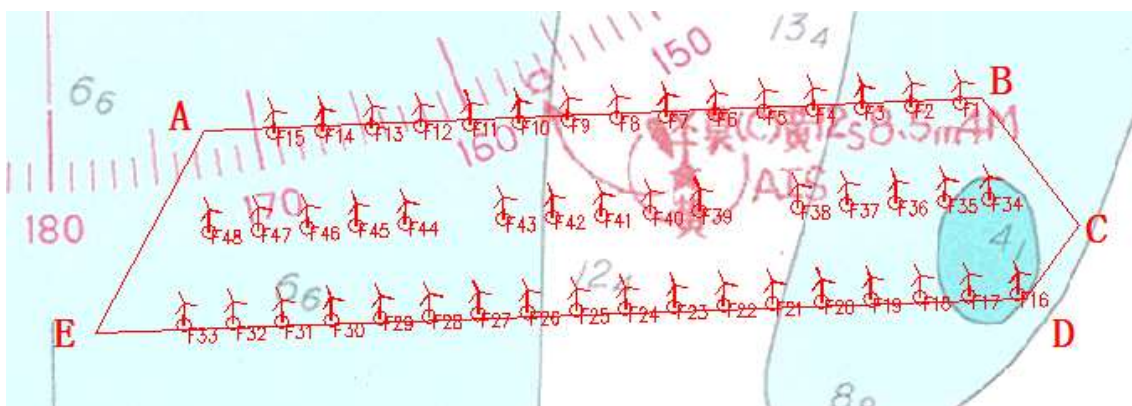
图 14.1-1 基于 WTG-4 的最优风机布置方案示意图
