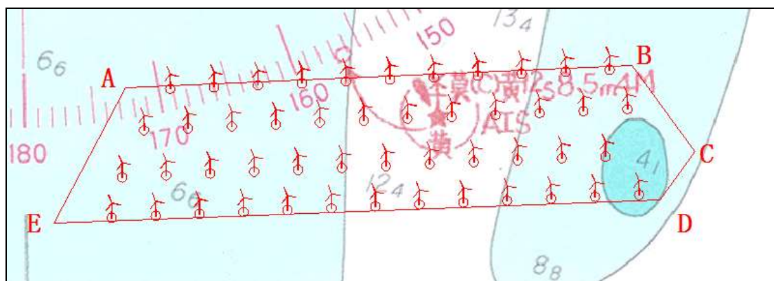
图 12.5-1 方案一风机布置图
