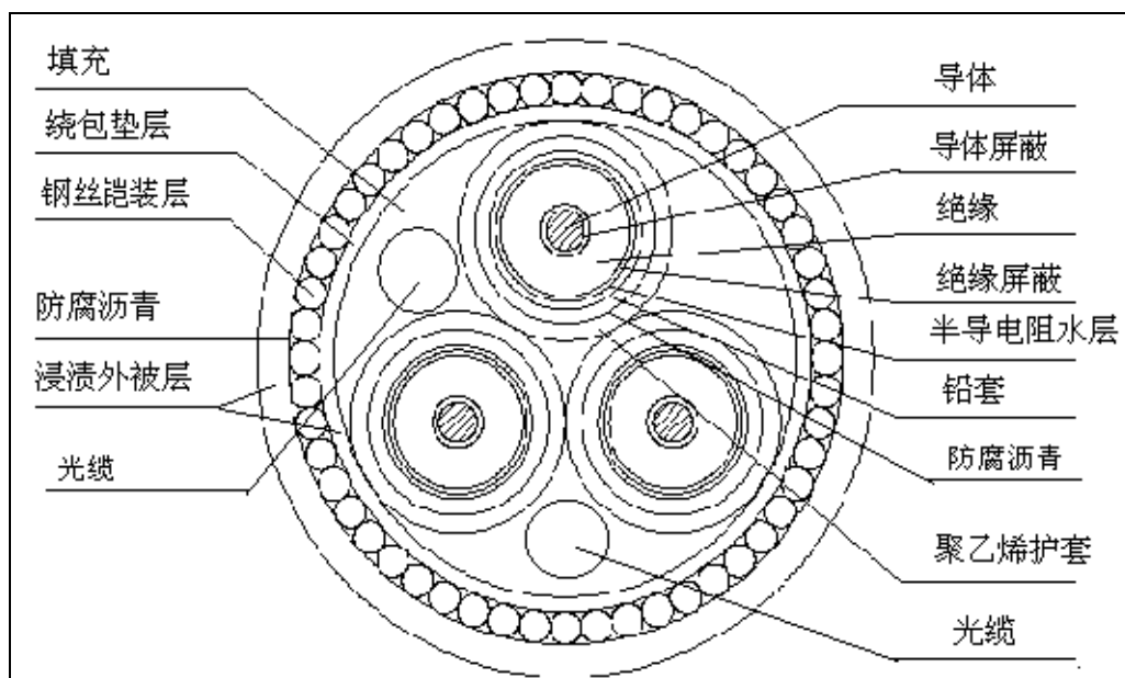
图 3.3-6 35kV 海底电缆剖面结构示意图
