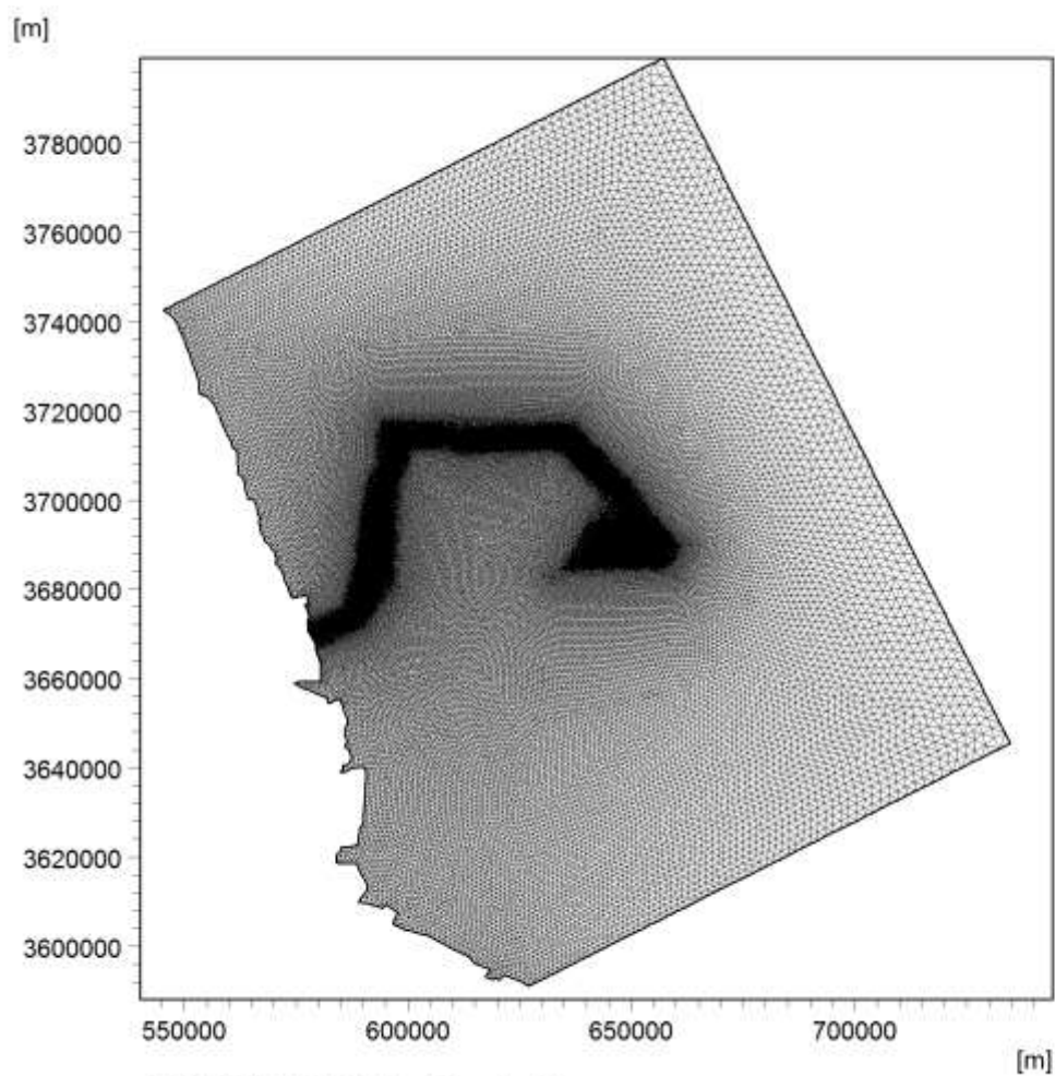
图 7.1-2 工程区域小模型网格图
