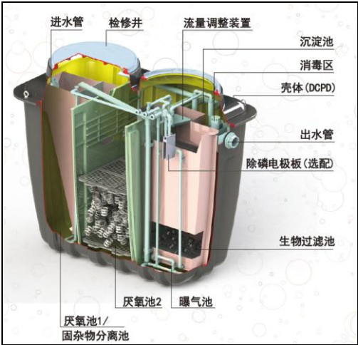
图 1 分散生活污水处理装置示意图
