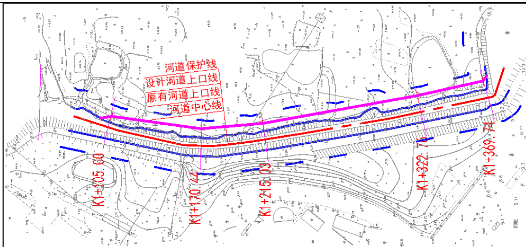
图2 堤防加高段平面图
