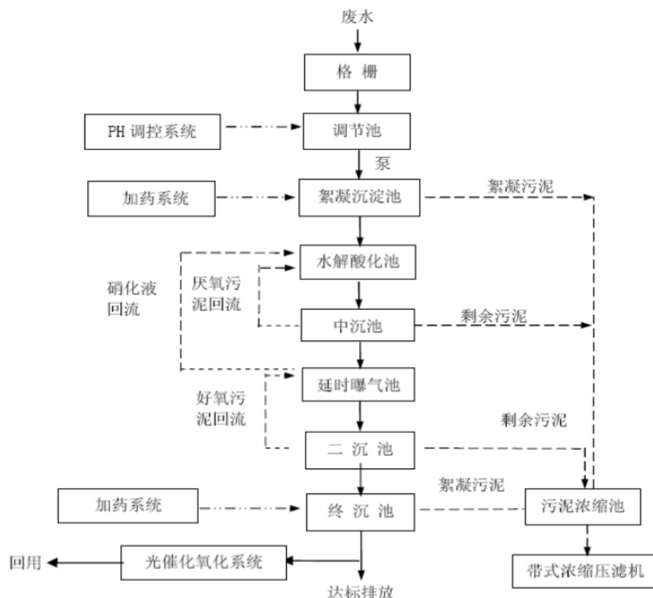
图 6.2-2 鹰泰水务（海安）有限公司处理工艺流程
