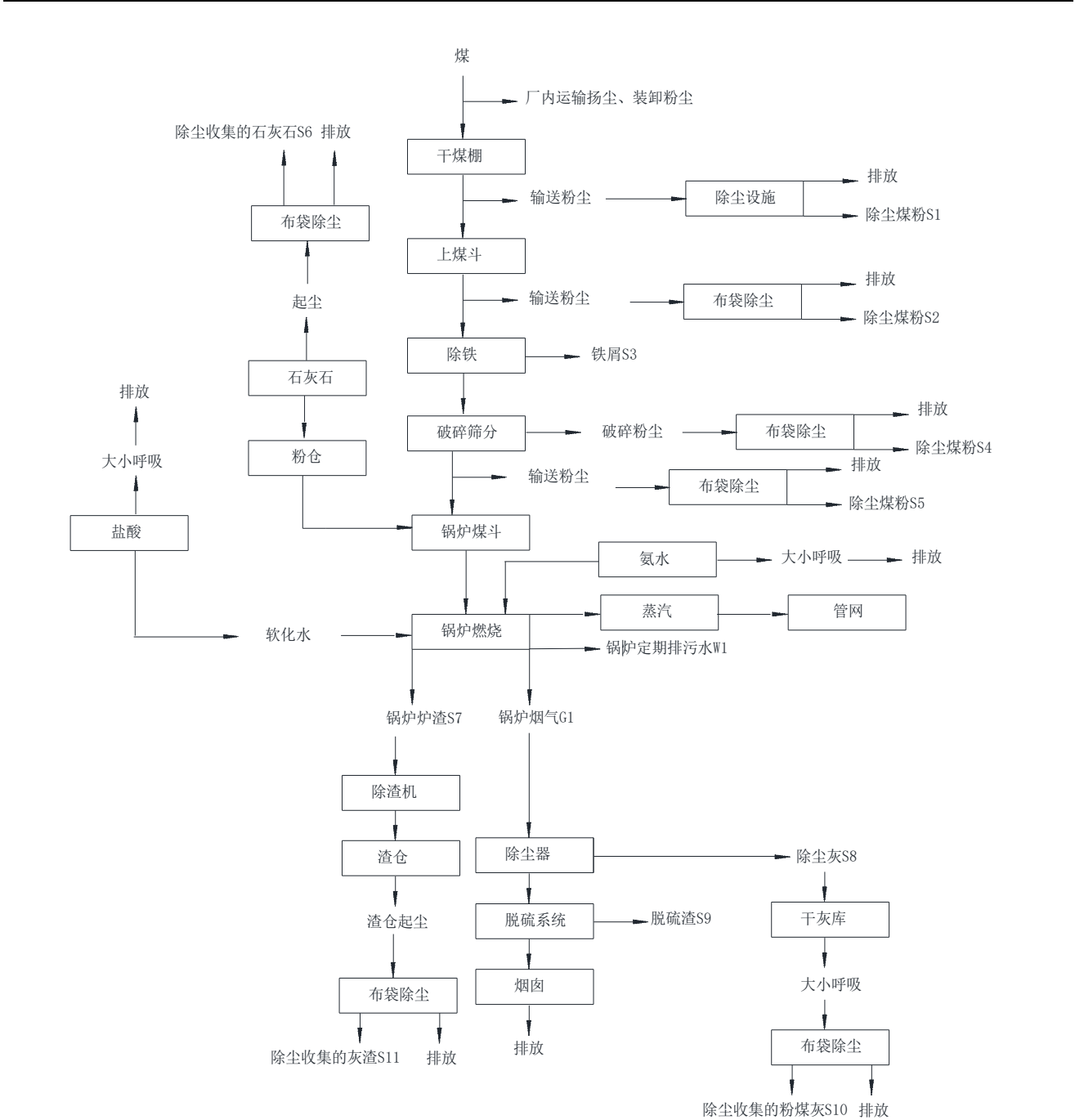
图 3.1-2 现有项目工艺流程图
