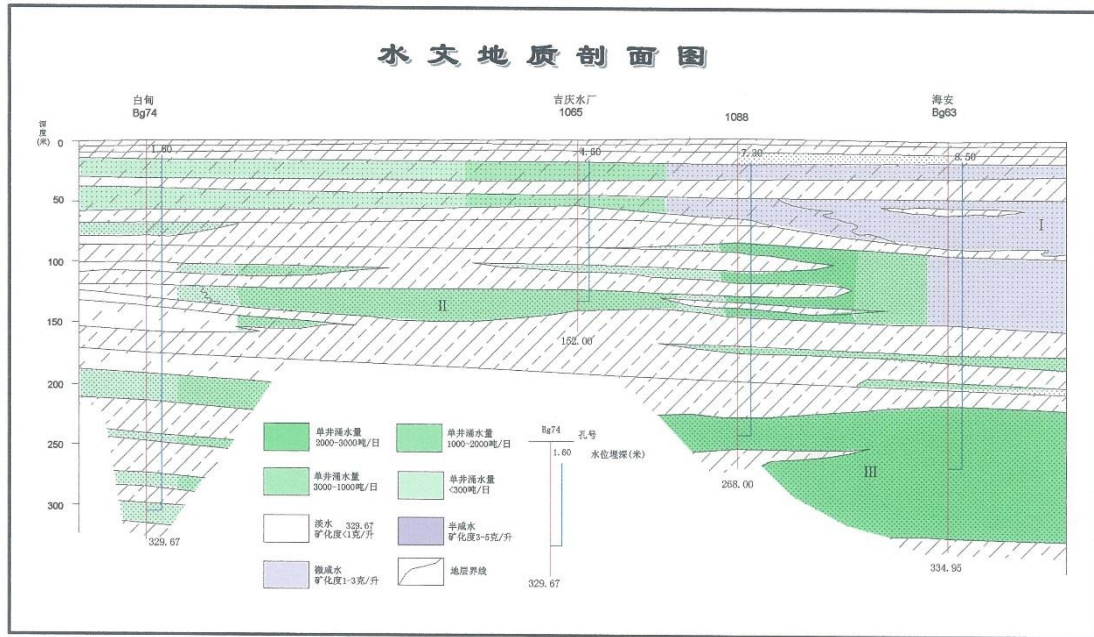
图 5.2-17 区域水文地质剖面图
