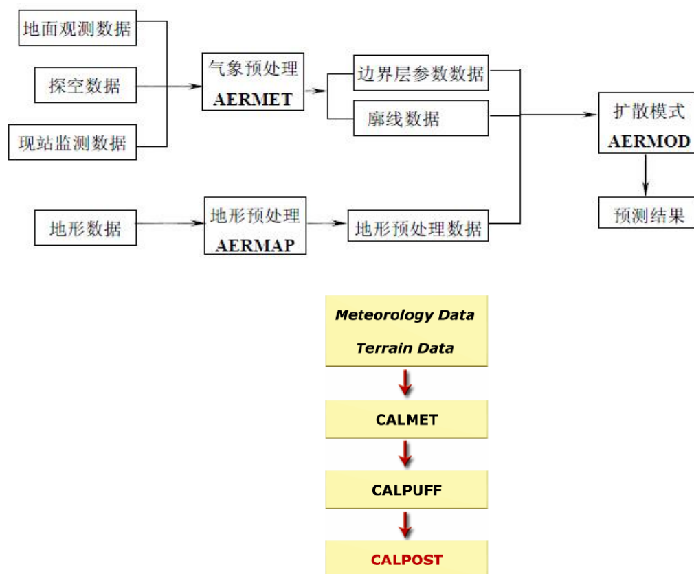
图 5.2-6 模式系统流程图
