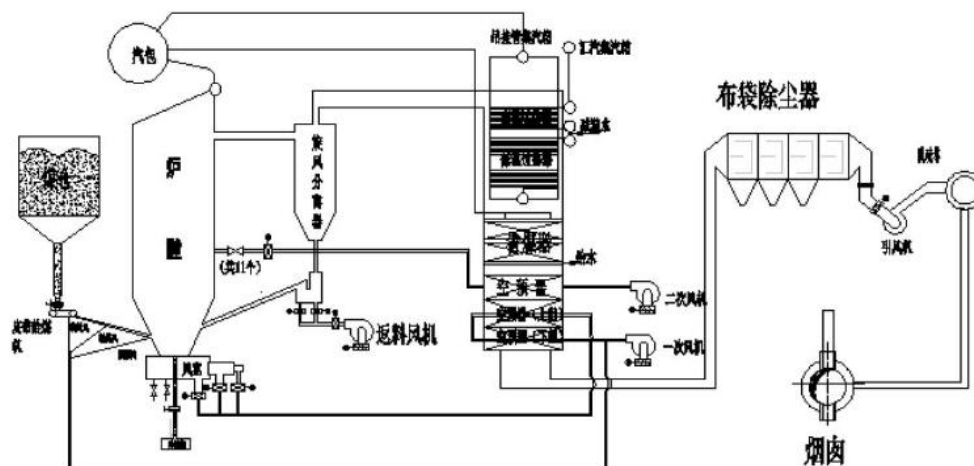
图 3.1-5 燃烧系统工艺流程示意图
