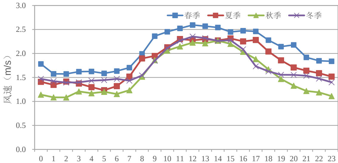
图 5.2-4 2017 年季节小时平均风速的日变化图
