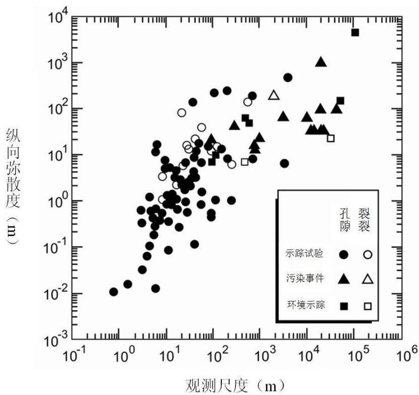
图 5.2-20 纵向弥散度与观测尺度之间的关系
