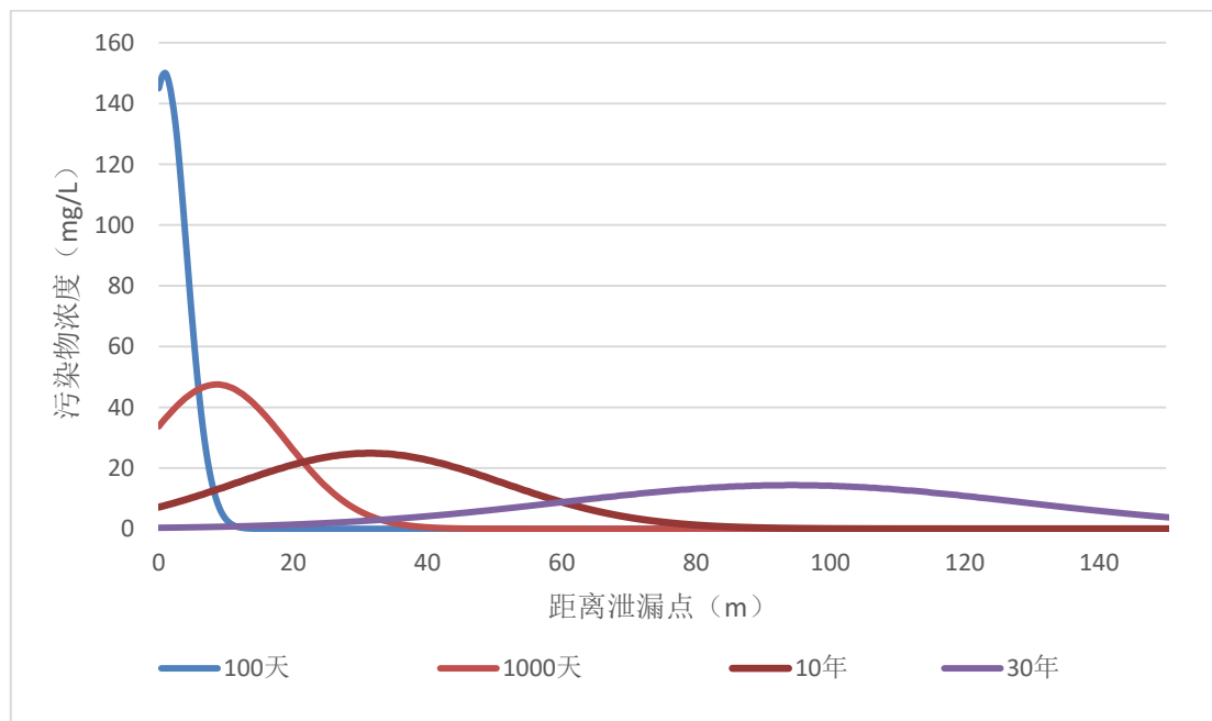
图 5.2-23 不同预测条件下石油类浓度变化图
