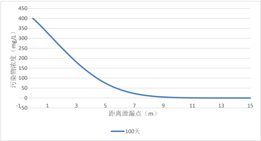
图 5.2-21 100 天预测条件下高锰酸盐指数浓度变化图
