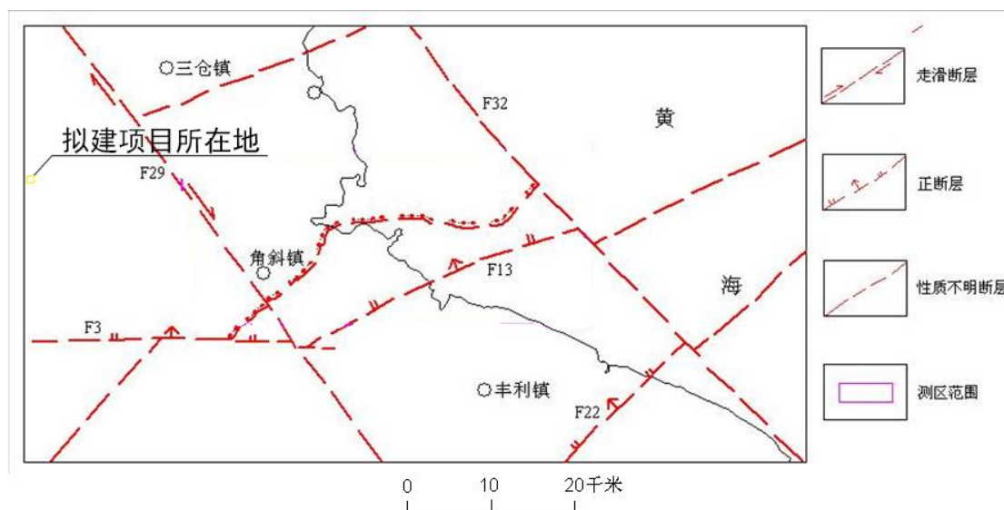
图 5.2-16 研究区及邻区主要地质构造
