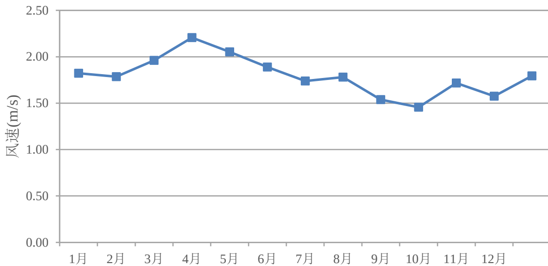
图 5.2-3 2017 年平均风速的月变化图
