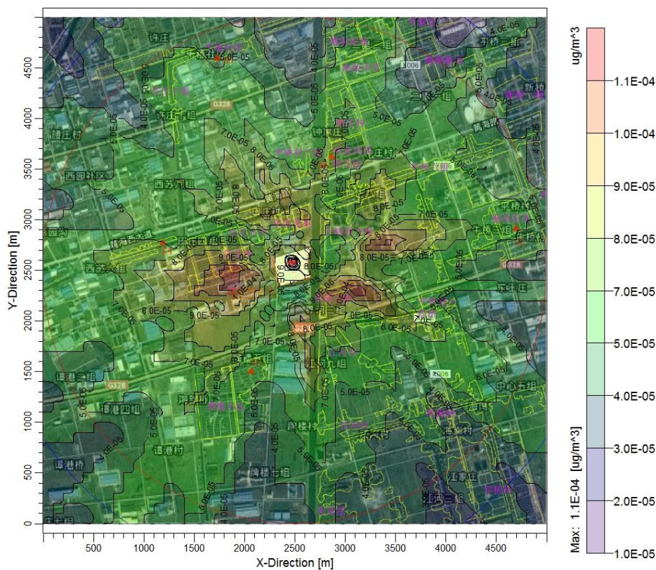
图5.2-12 评价区域Hg日均最大浓度分布图
