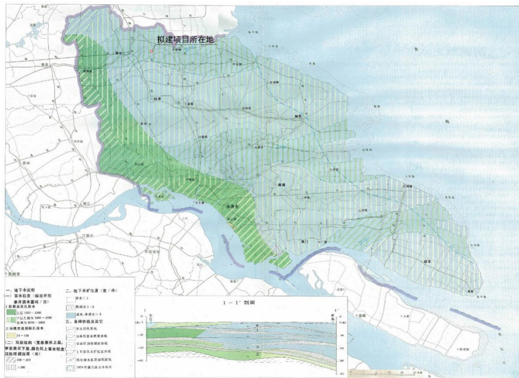
图 5.2-18 南通市水文地质图
