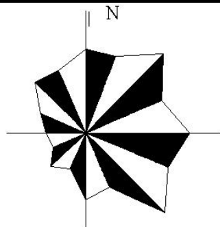
图 5.2-1 近 20 年风向玫瑰图
