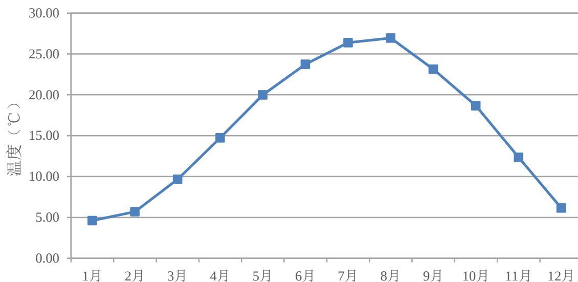
图 5.2-2 2017 年平均温度的月变化
