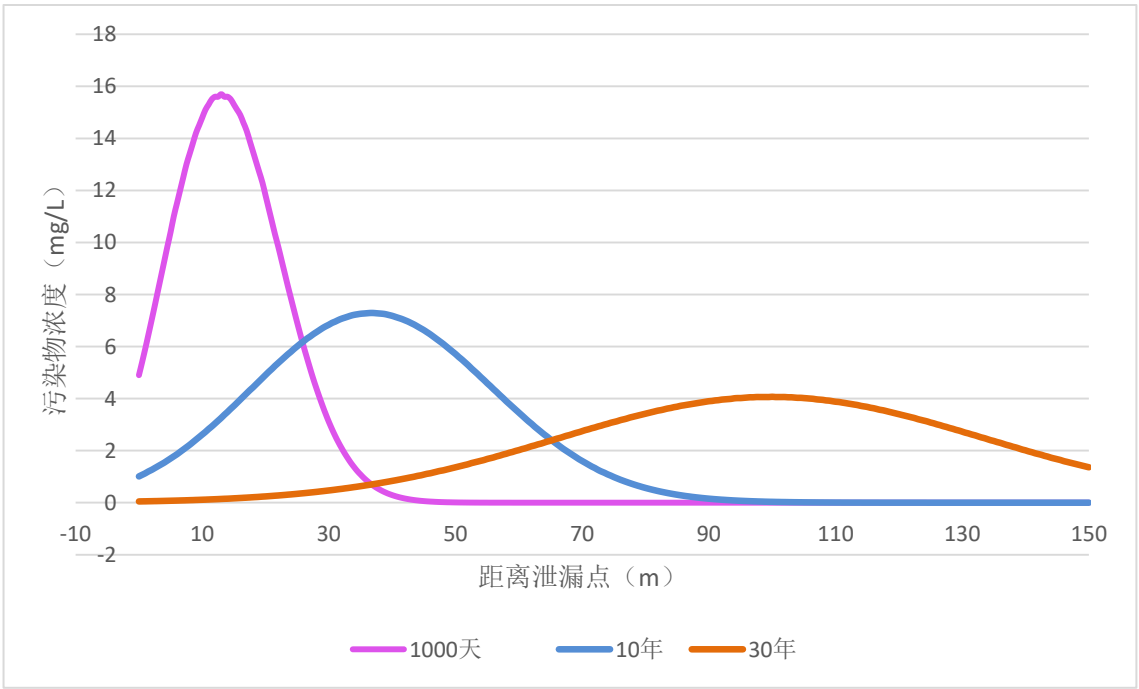
图 5.2-22 不同预测条件下高锰酸盐指数浓度变化图
