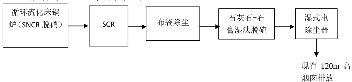
图 6.1-1 锅炉烟气处理工艺框架图
