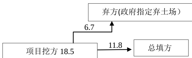
图 5-2 本项目土石方平衡图（单位：万 m 3 ）
