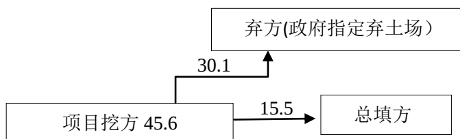
图 5-2 本项目土石方平衡图（单位：万 \text{m}^3 ）
