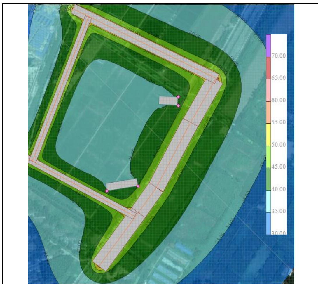
图 7-4 本项目周边规划道路夜间噪声预测等声值线图
