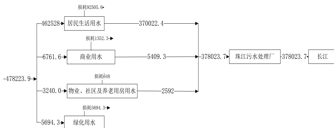
图 5-3 建设项目水平衡图 (单位: m 3 /a)
