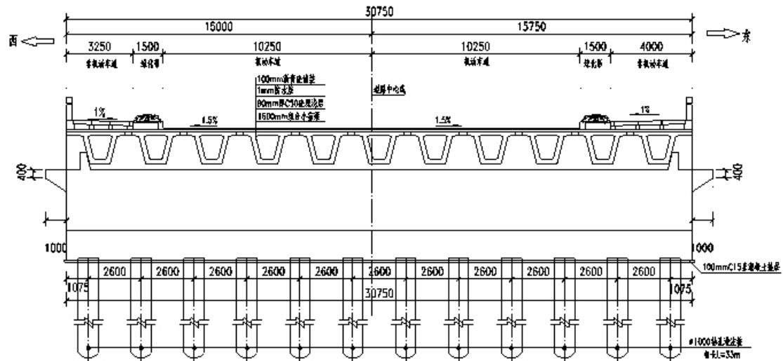
3.2-3 十二号路一号桥桥台横断面图
