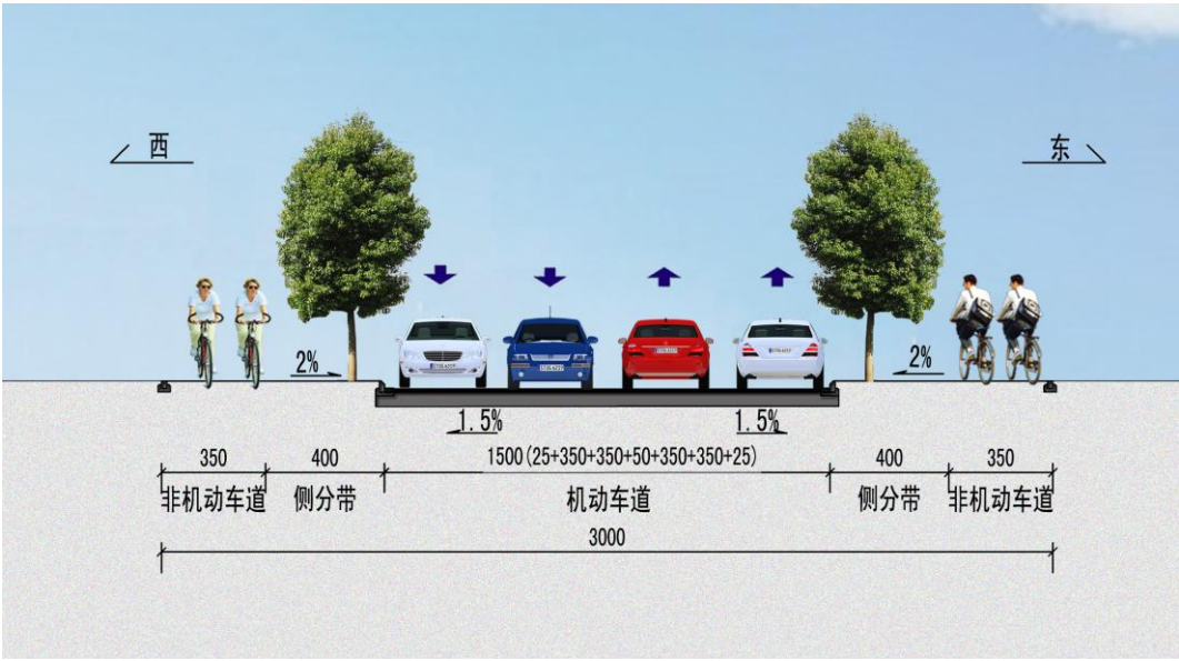
图 3.2-2 十二号路工程横断面图
