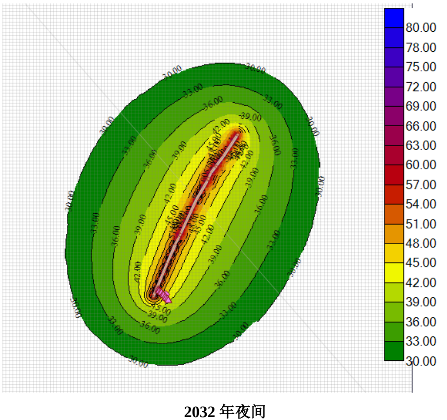
图 6.4-7 十二号路等声级线图
