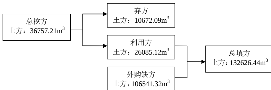
图 3.2-7 拟建项目路基工程土石方平衡图
