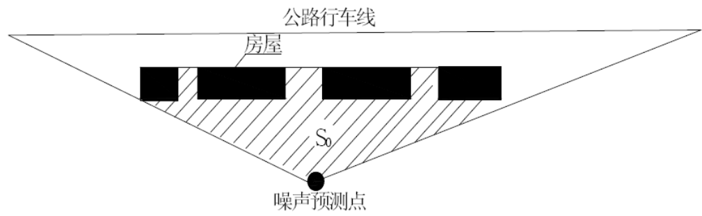
图 6.4-5 房屋降噪量估算示意图
