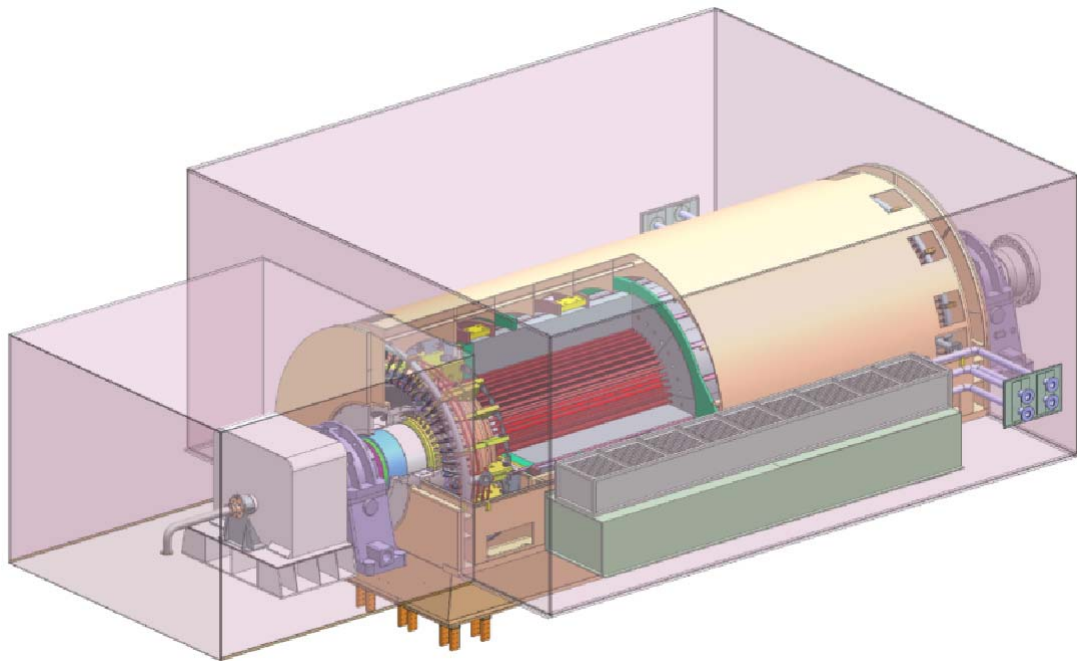
图 3.5-1 带有隔声罩的调相机
