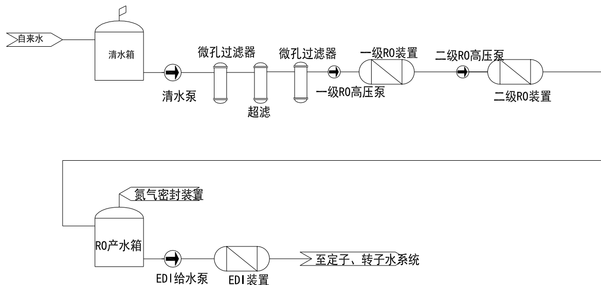
图 3.1-2 除盐水处理工艺
