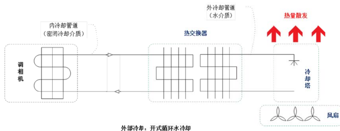
图 3.1-1 调相机冷却系统原理及流程
