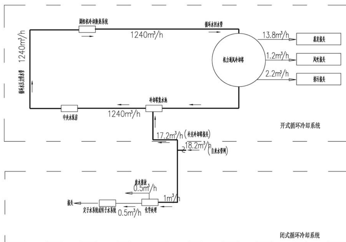
图 3.1-3 水量平衡图(夏季工况下)
