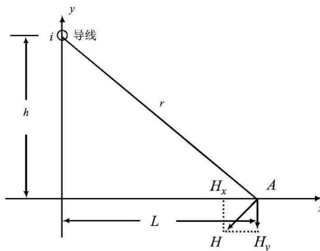
图 6.1-7 磁场向量图
