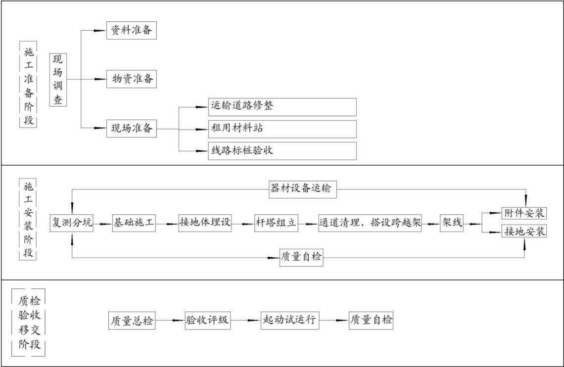
图 3.1-3 新建架空线路施工工艺流程图
