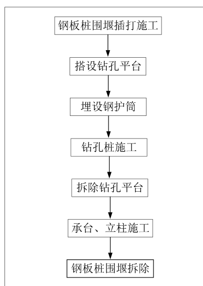
图 3.1-4 围堰法施工工艺流程图
