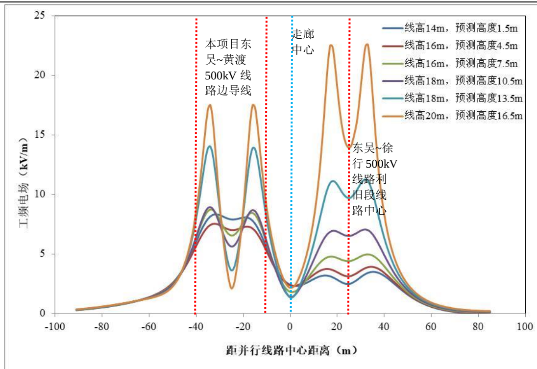
图 6.1-13 情形 1 不同计算高度工频电场强度预测结果
