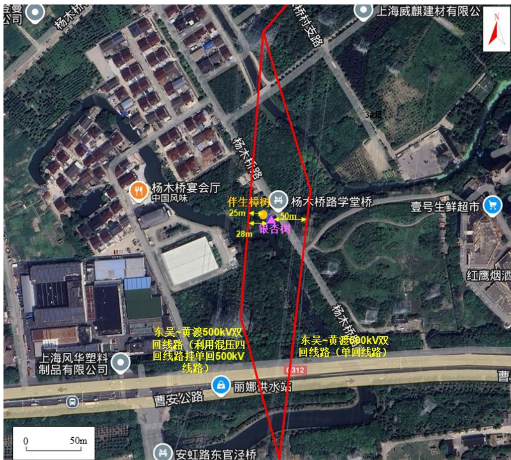
图 4.5-4 本项目与古树名木相对位置示意图
