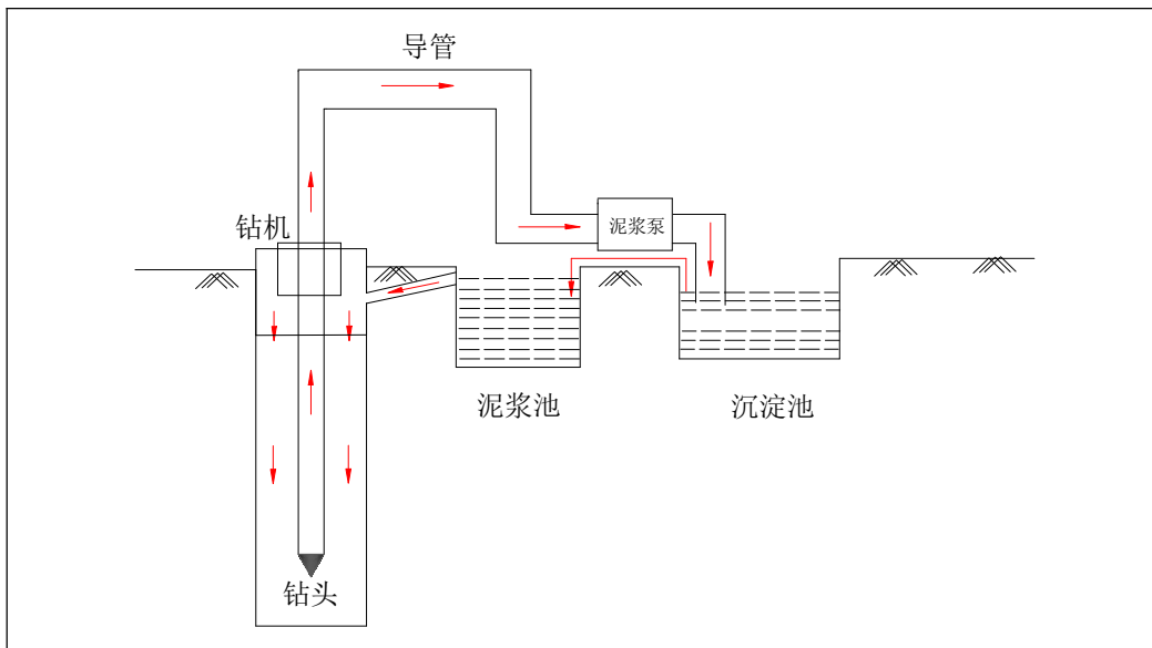
图 3.1-5 采用泥浆护壁钻机正循环法钻进施工工艺
