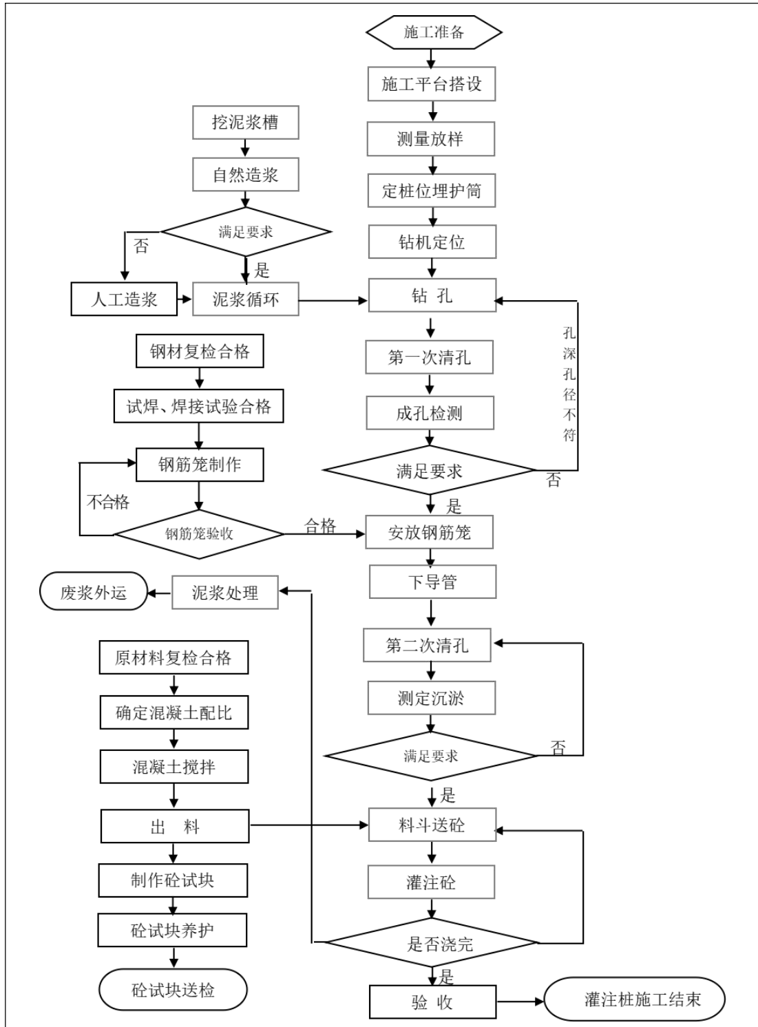
图 3.1-4 钻孔灌注桩的施工流程图
