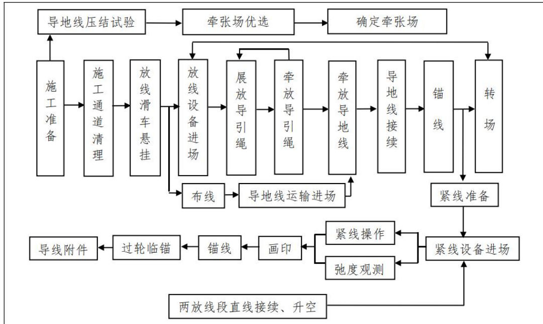
图 3.1-8 架线施工流程图
