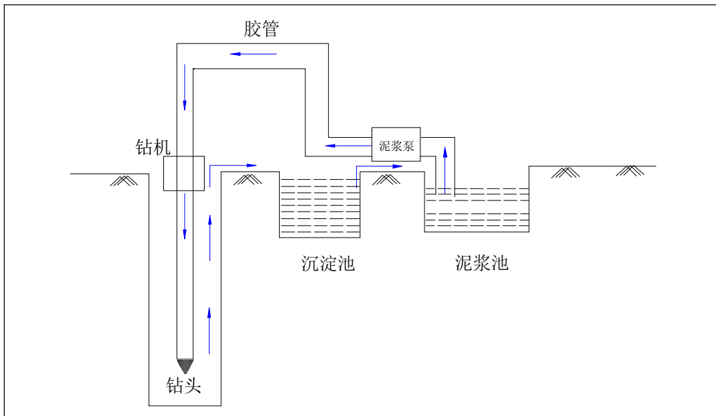
图 3.1-6 采用泥浆护壁钻机反循环法钻进施工工艺
