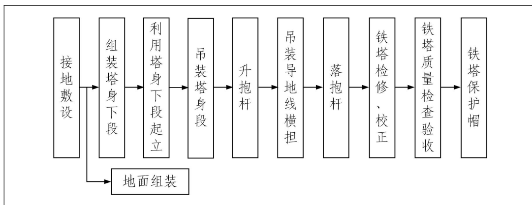
图 3.1-7 杆塔组立及接地工程施工流程图
