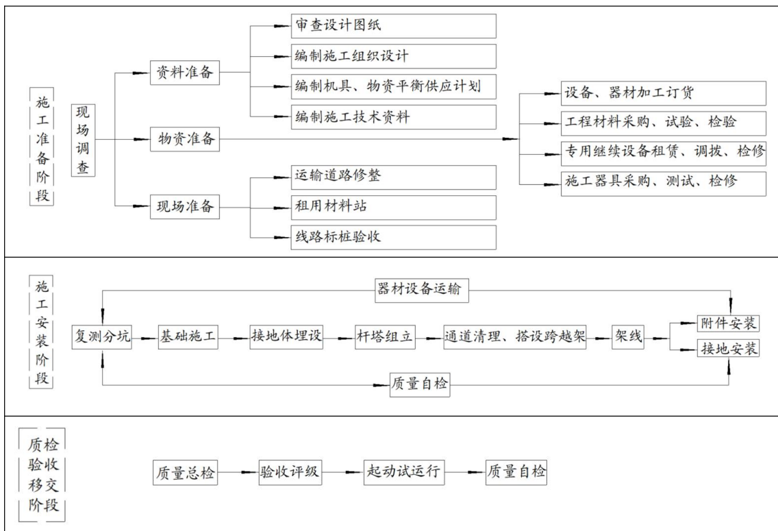
图 3.1-3 新建架空线路施工工艺流程图
