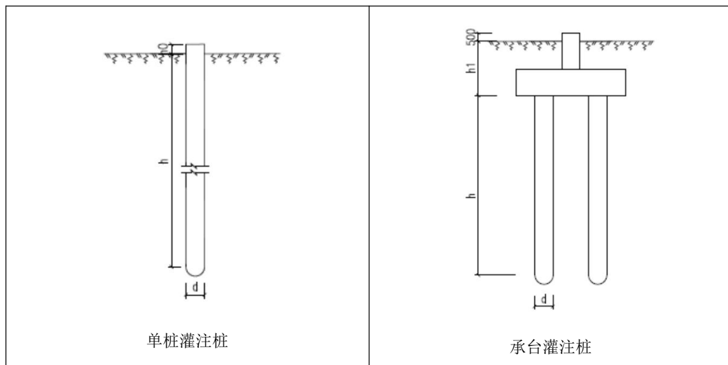
图 3.1-2 本项目塔基基础一览图
