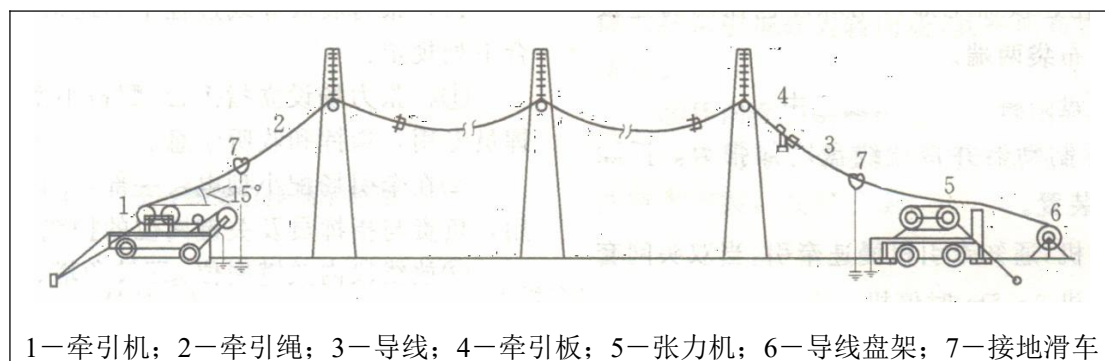
图 3.1-9 牵、张系统构成示意图
