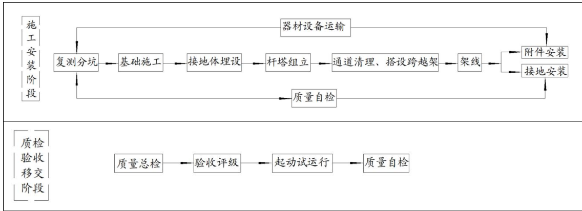
图 3.1-3 新建架空线路施工工艺流程图
