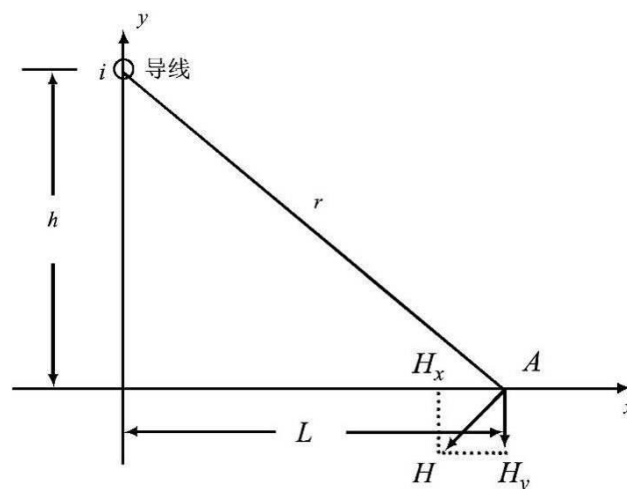
图 6.1-7 磁场向量图
