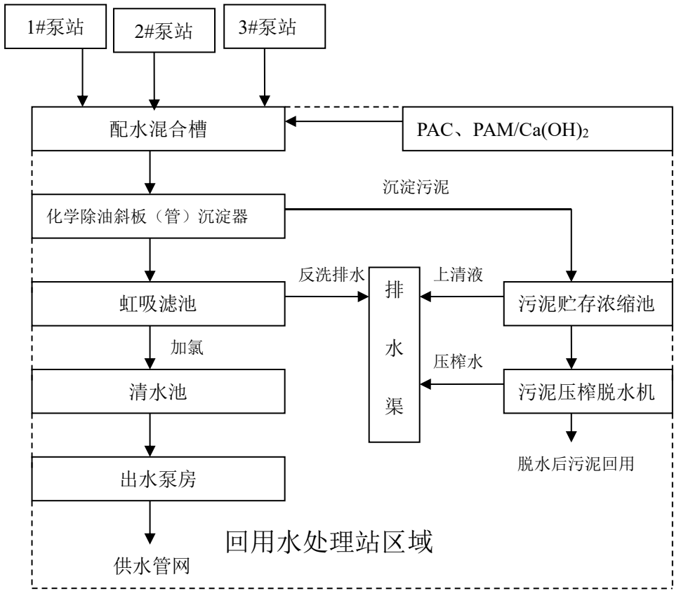
图 7.2-1 三回水处理系统工艺流程图
