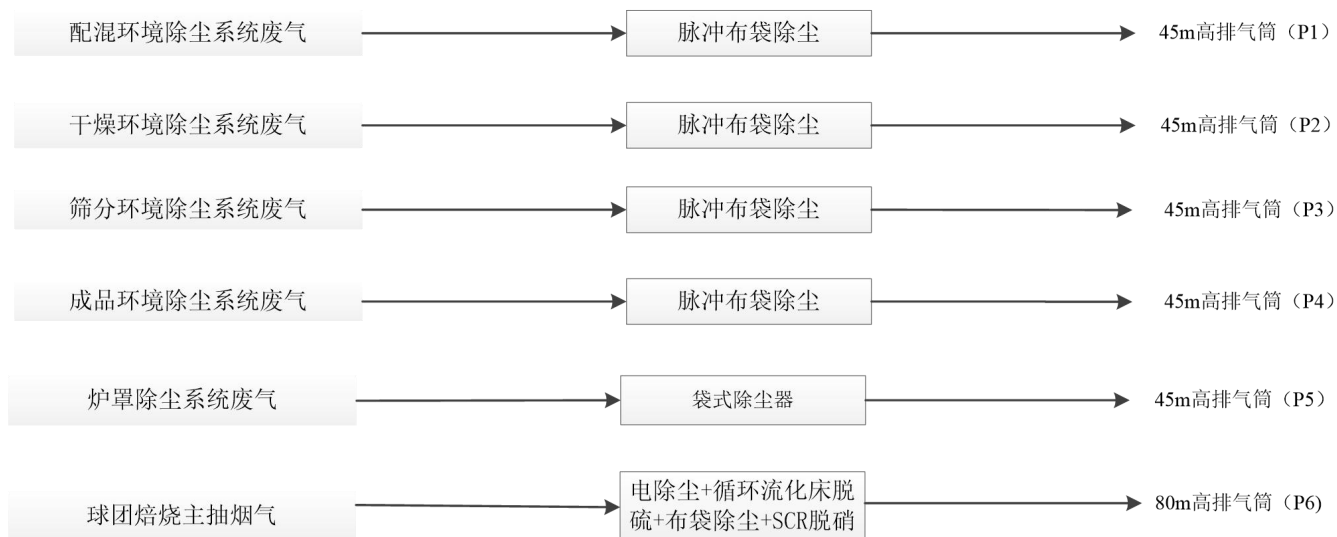
图 7.1.1-1 生产过程废气收集、处置示意图
