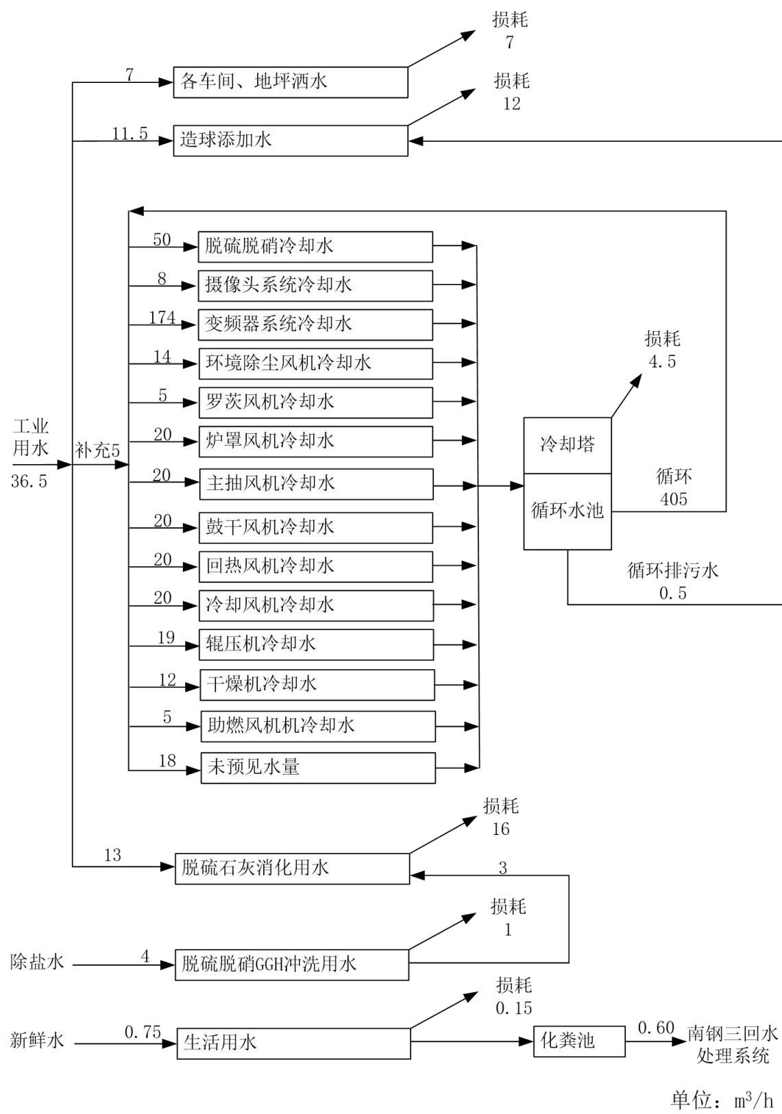
图 4.2.5-1 本项目水平衡图 (单位: m³/h)
