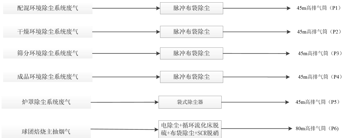
图 4.2.1-2 生产过程废气收集、处置示意图
