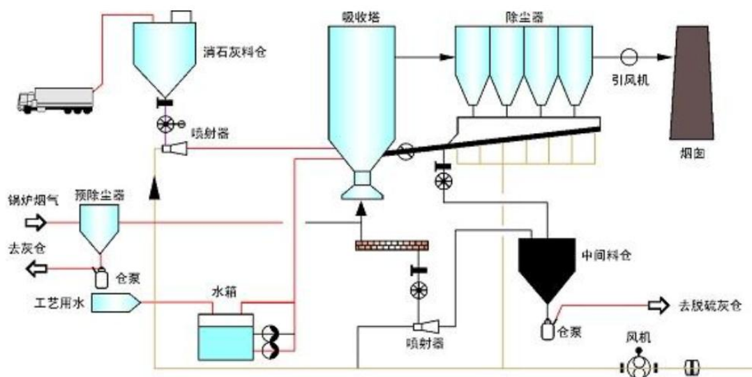
图 7.1.1-2 典型的循环流化床+布袋除尘脱硫除尘工艺流程图
