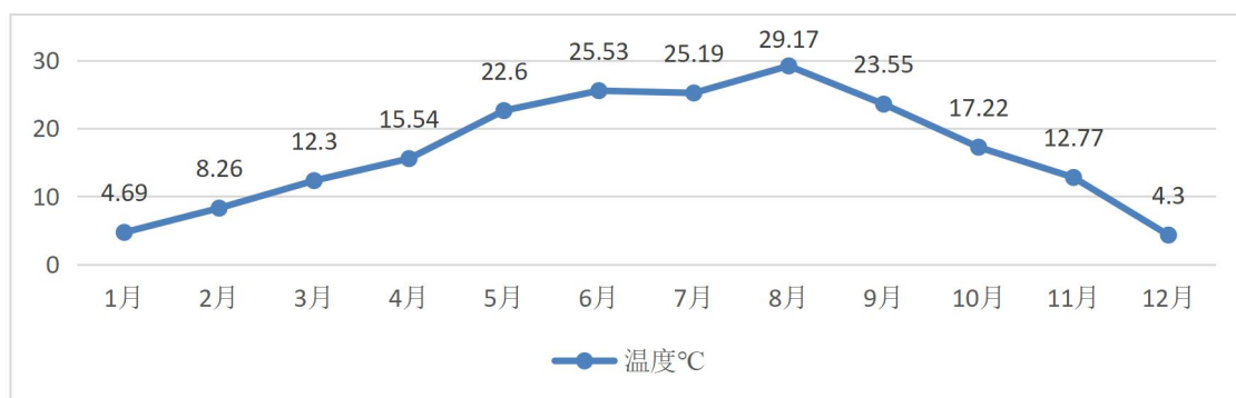
图 6.2.1-1 浦口 2020 年年平均温度的月变化图
