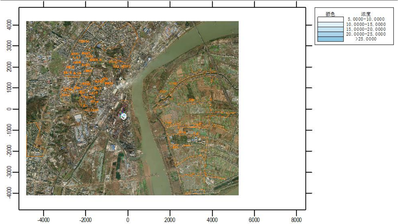
图 6.2.5-1 最常见条件下一氧化碳泄漏风险敏感目标时间-浓度图
