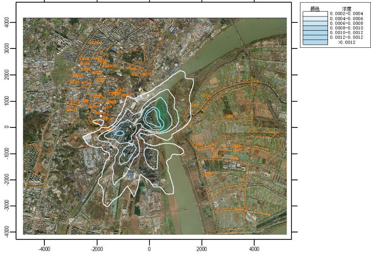
图 6.2.1-17 叠加后 SO 2 日均浓度贡献值分布图
