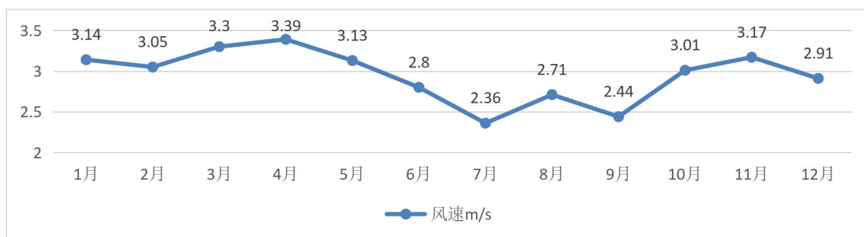
图 6.2.1-2 浦口 2020 年平均风速月变化
