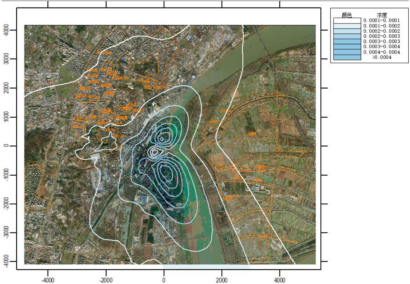
图 6.2.1-22 叠加后 PM 10 年均浓度贡献值分布图
