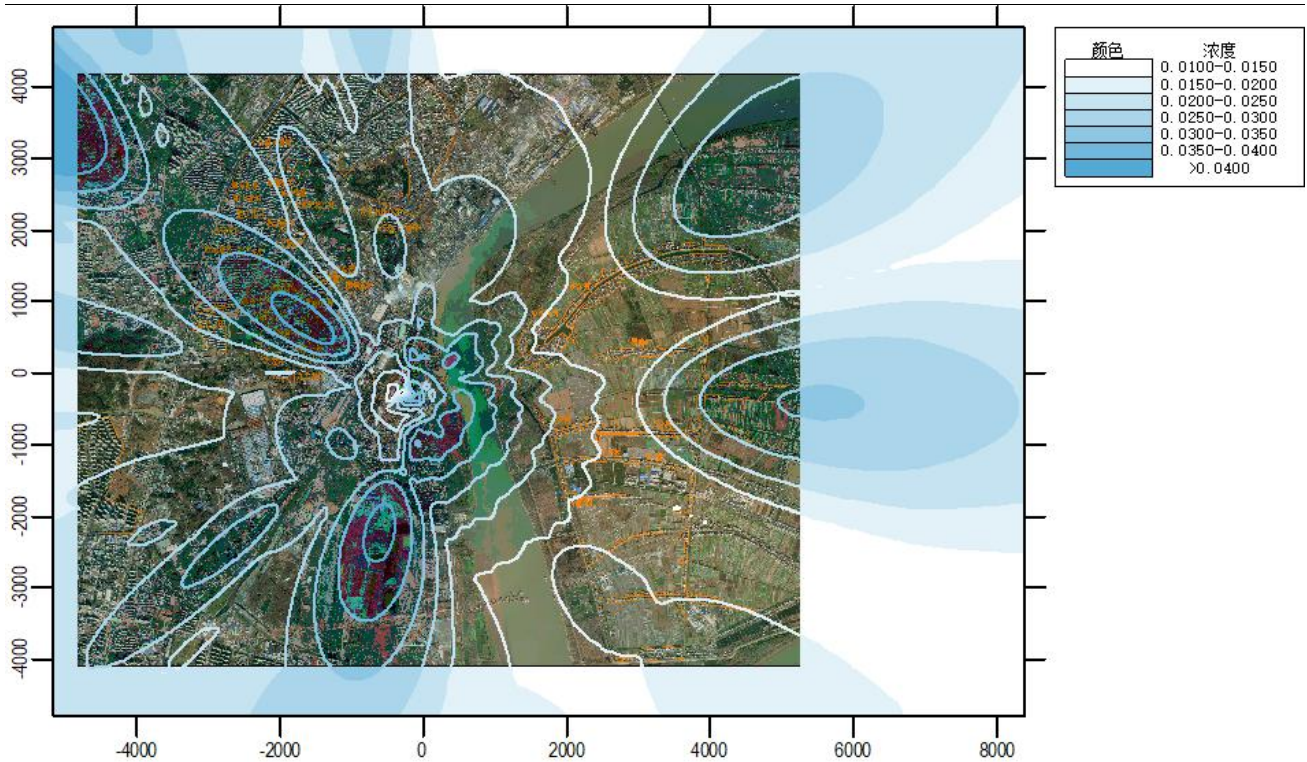
图 6.2.1-25 非正常工况下二氧化氮最大浓度分布图
