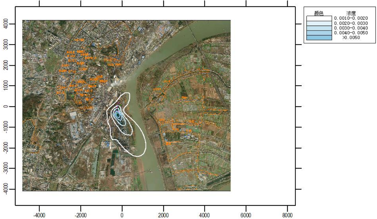
图 6.2.1-14 PM_{10} 年均浓度贡献值分布图
