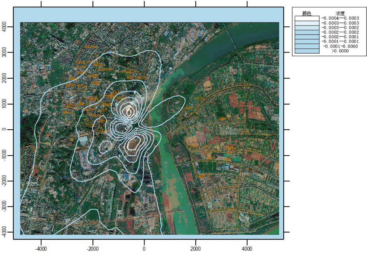
图 6.2.1-19 叠加后 NO 2 日均浓度贡献值分布图
