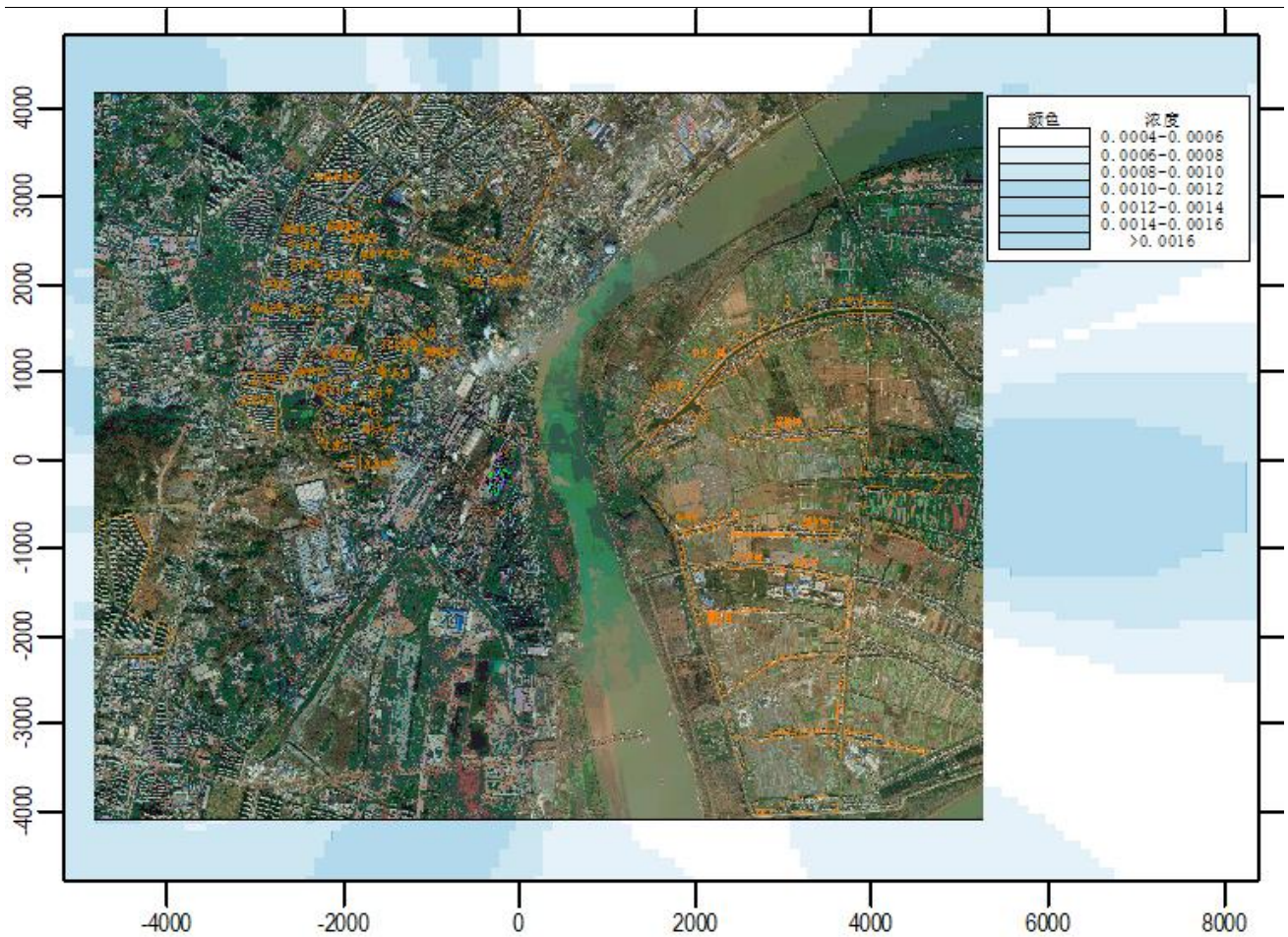
图 6.2.1-24 非正常工况下氟化物最大浓度分布图
