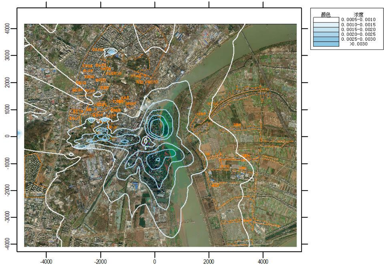
图 6.2.1-21 叠加后 PM 10 日均浓度贡献值分布图
