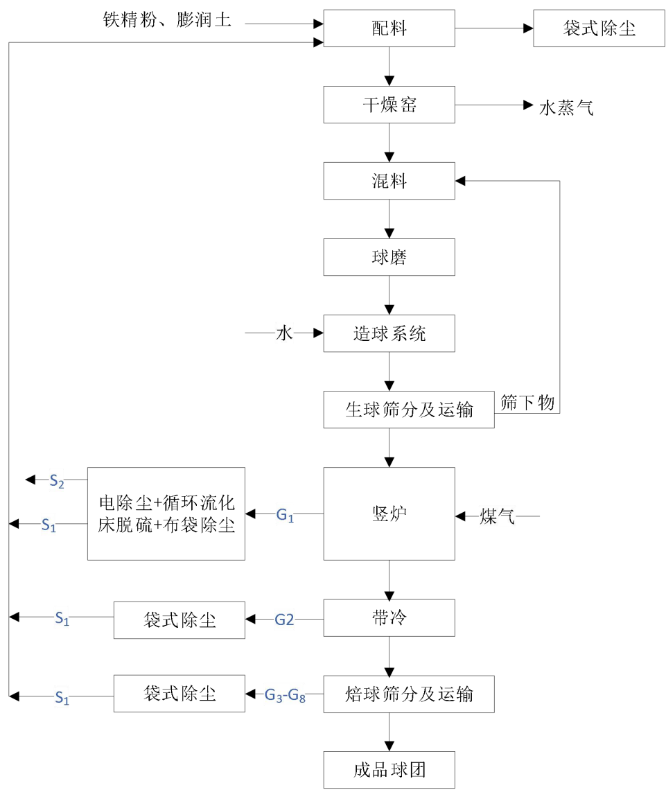
图3.2-1 现有球团工序生产工艺流程
