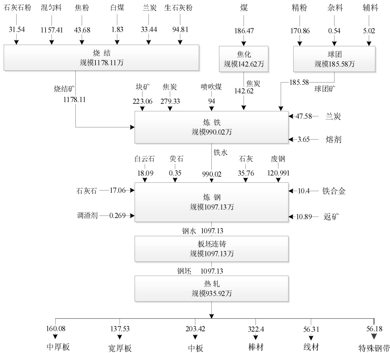
图 3.1.7-1 南钢公司现有生产工艺流程示意图
