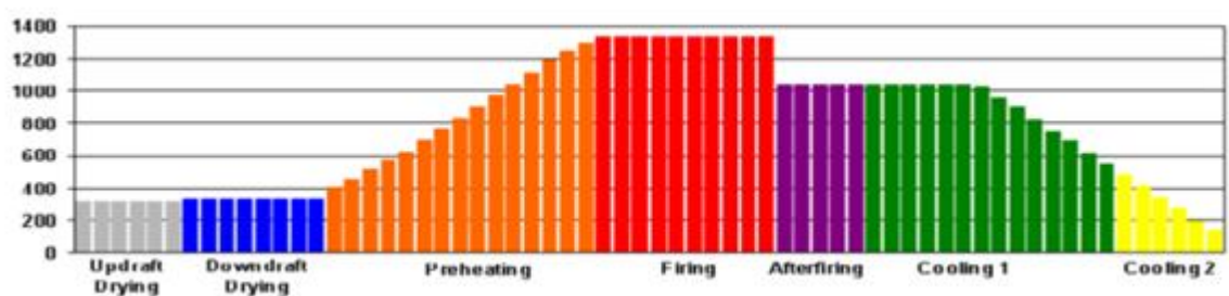
图 2.1-2 温度分布及风系统图
