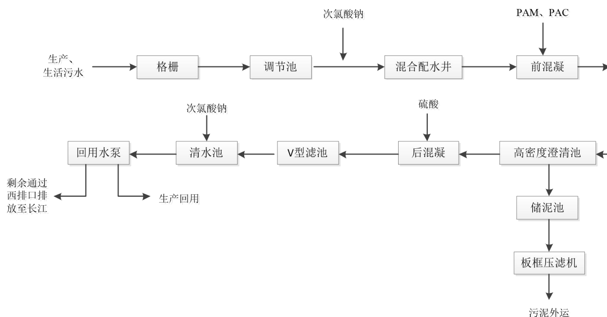
图 3.1.7-1 回用水厂处理工艺流程图
