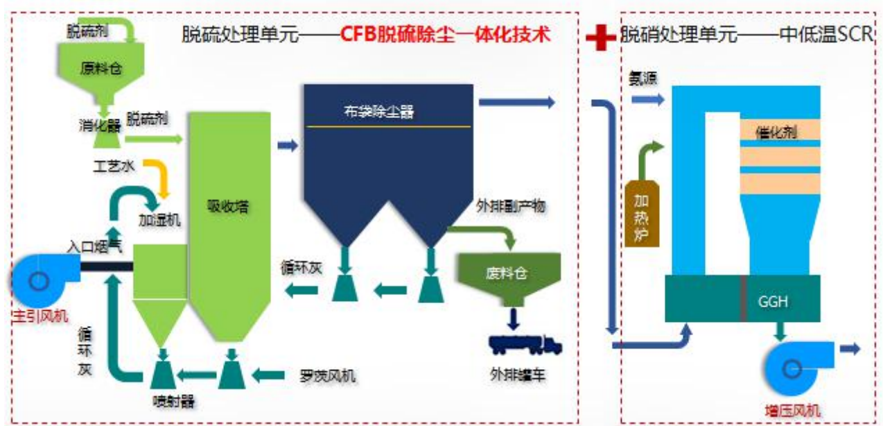
图 1 脱硫脱硝工艺流程图
