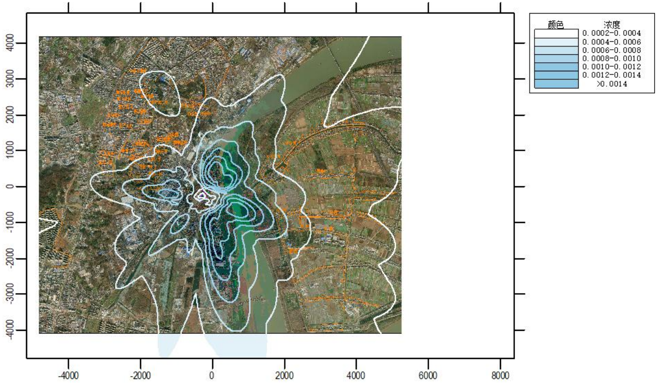
图 6.2.1-7 SO 2 小时浓度贡献值分布图
