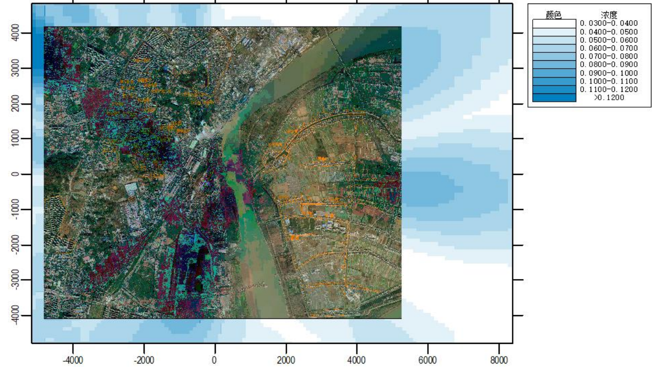
图 6.2.1-24 非正常工况下二氧化硫最大浓度分布图
