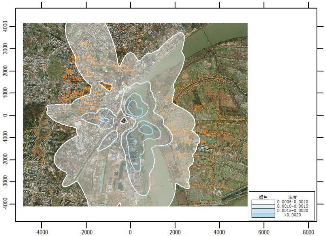
图 6.2.1-10 NO 2 小时浓度贡献值分布图
