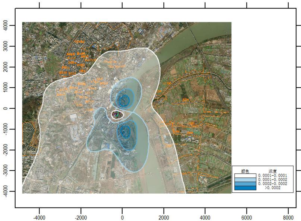
图 6.2.1-12 NO 2 年均浓度贡献值分布图
