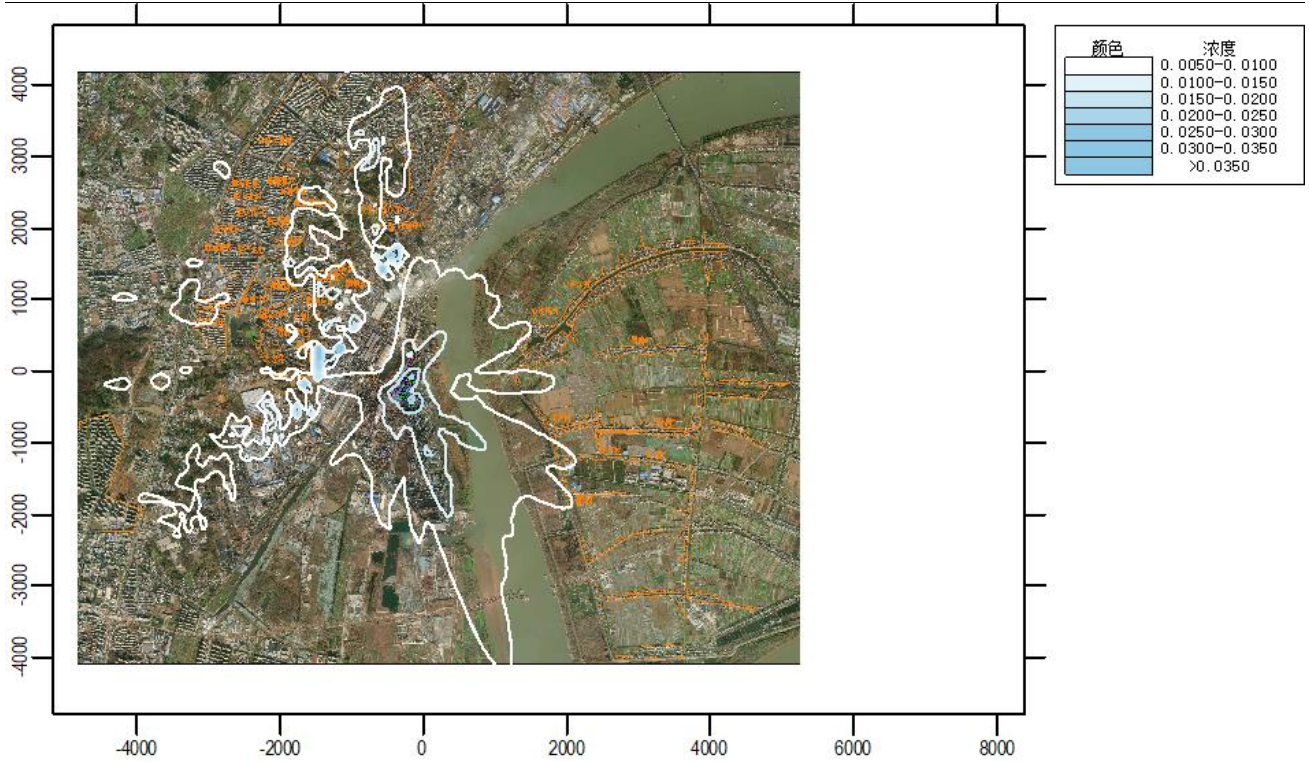
图 6.2.1-13 PM_{10} 日均浓度贡献值分布图
