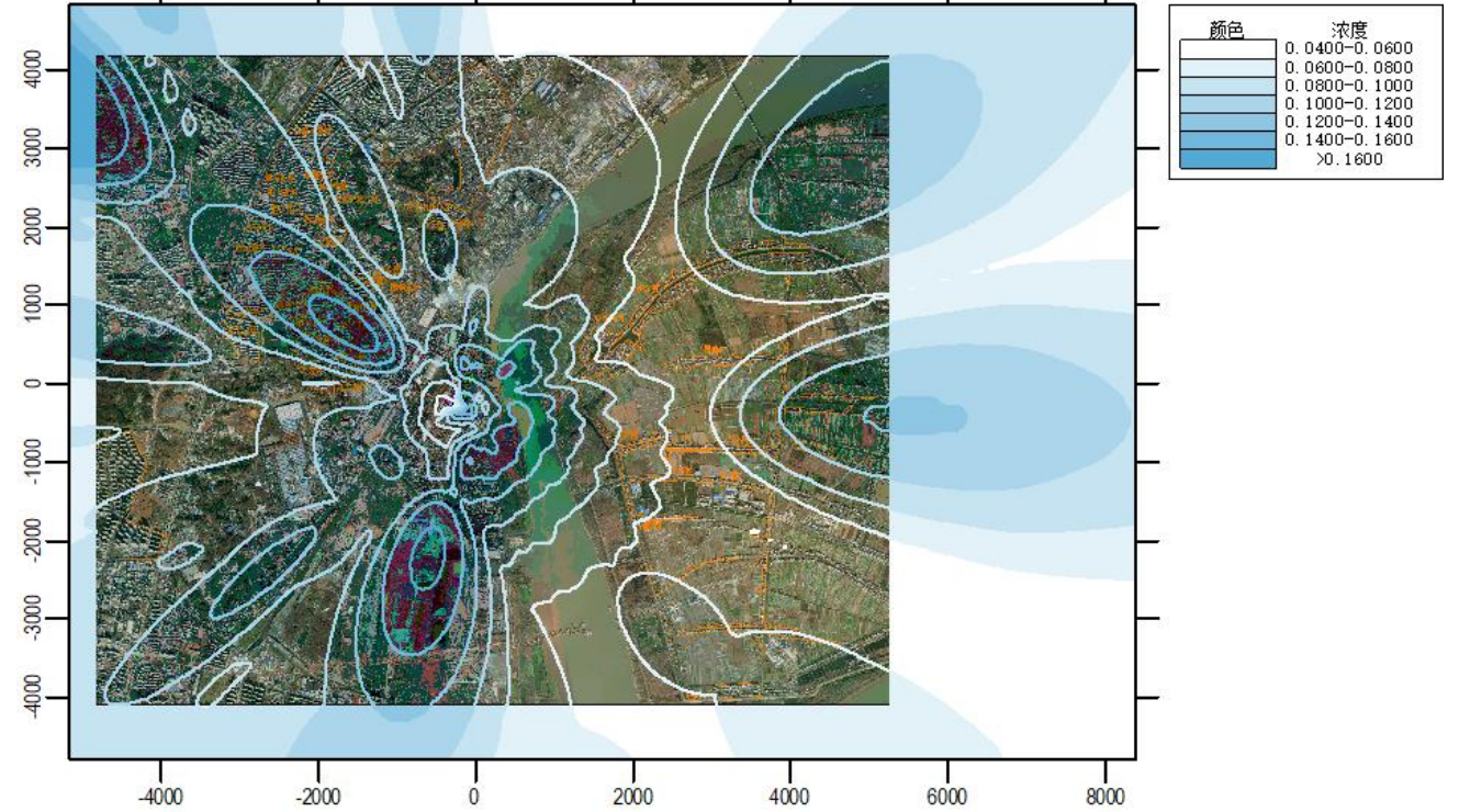
图 6.2.1-24 非正常工况下 PM 2.5 最大浓度分布图
