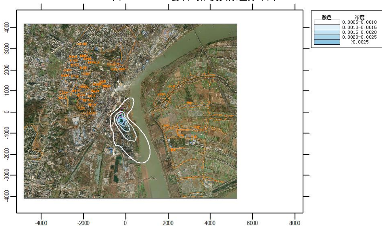
图 6.2.1-16 PM 2.5 年均浓度贡献值分布图
