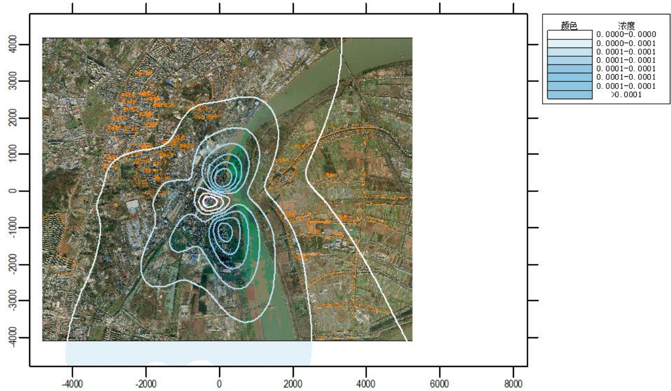
图 6.2.1-9 SO 2 年均浓度贡献值分布图
