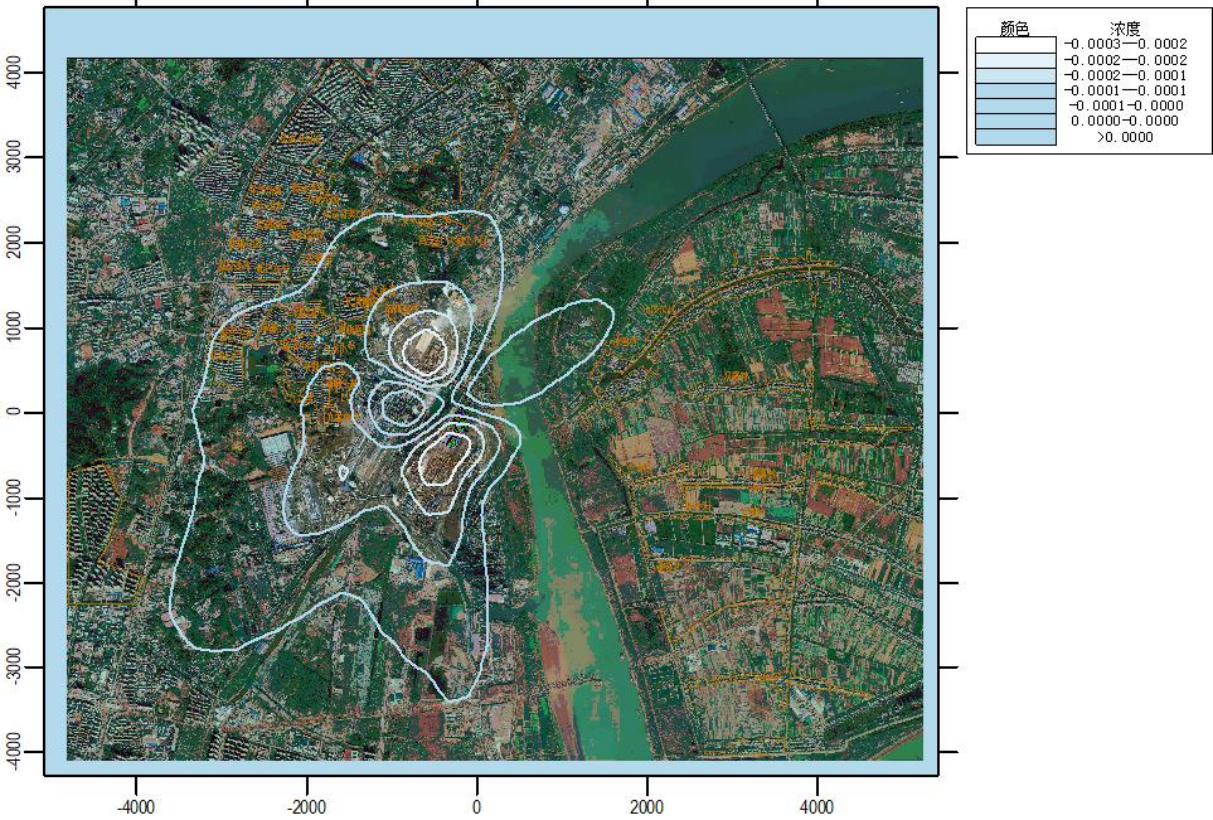
图 6.2.1-18 叠加后 SO 2 年均浓度贡献值分布图
