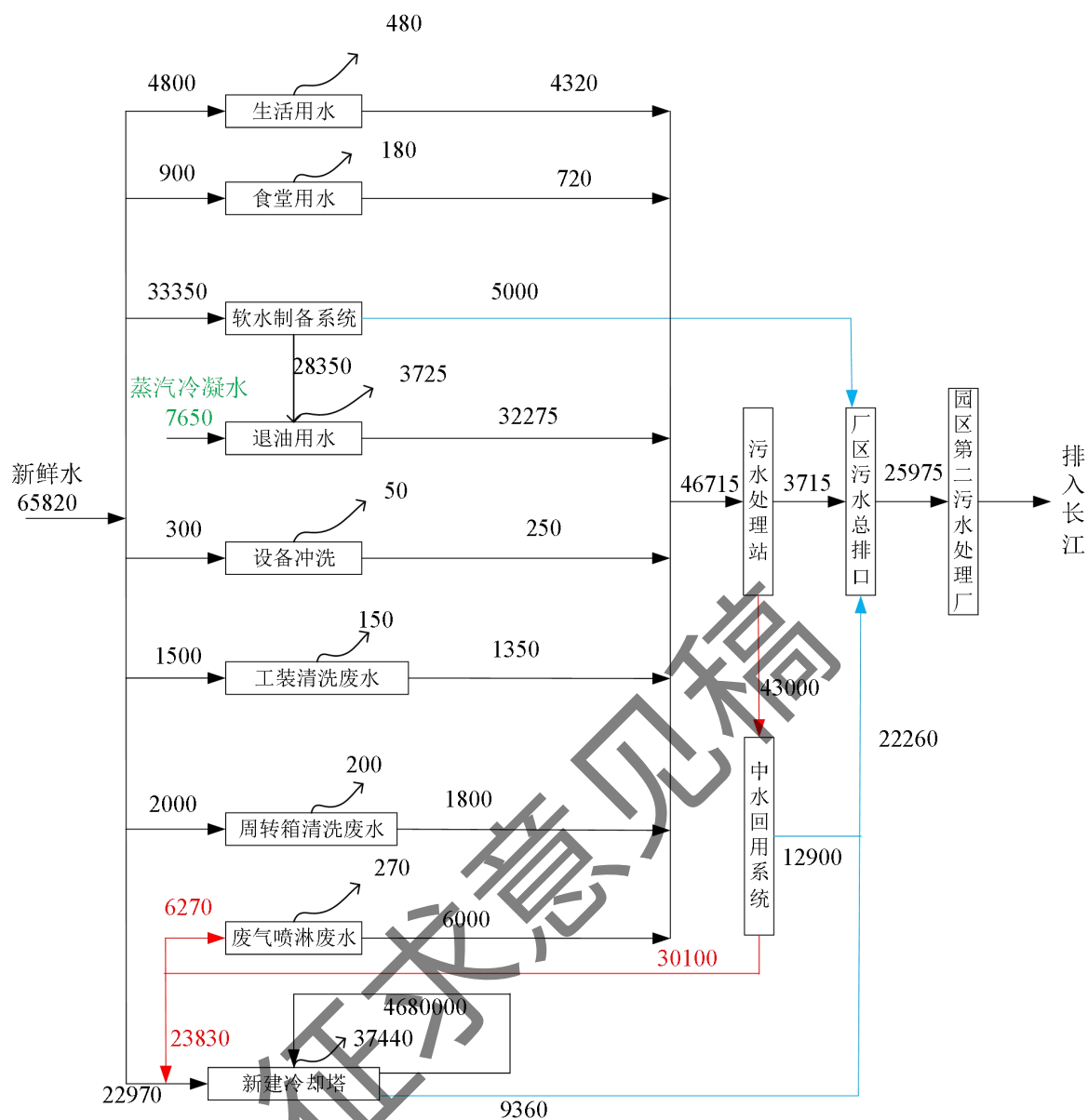
图 4.3-1 改扩建项目水量平衡图 ( \text{m}^3/\text{a} )
