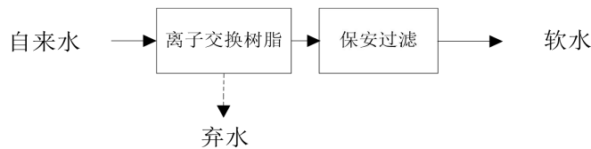
图 4.3-3 软水制备系统工艺流程图
