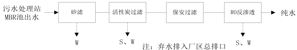
图 3.1-3 纯水制备系统工艺流程图
