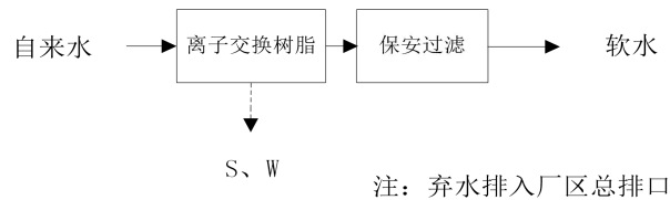
图 3.1-2 软水制备系统工艺流程图
