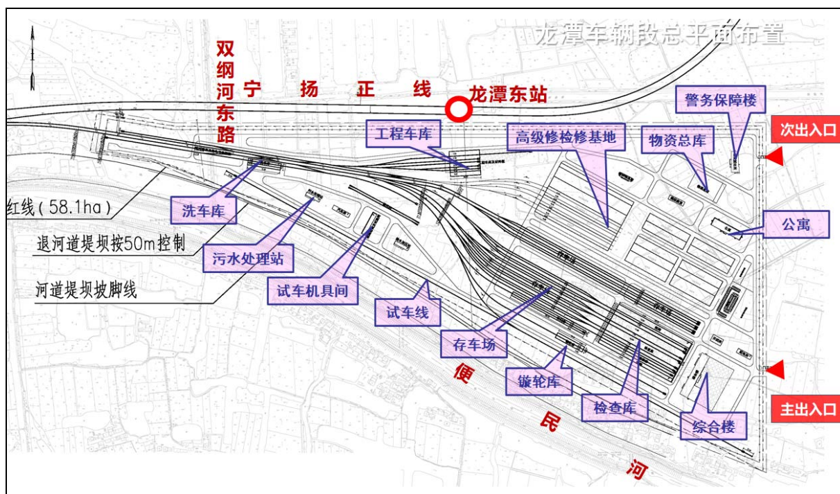
图 2.1-21 龙潭车辆段总平面布置图
