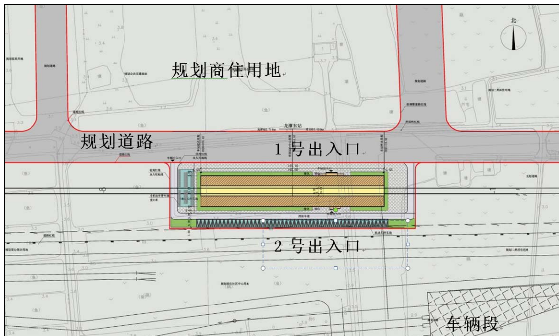
图 2.1-7 龙潭东站总平面布置图
