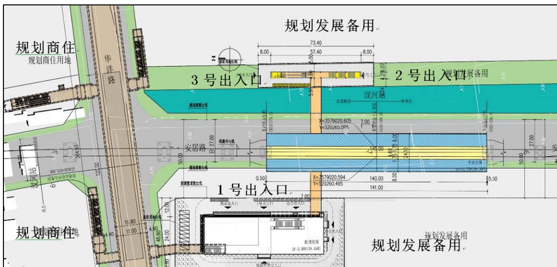
图 2.1-14 汉河站总平面布置图
