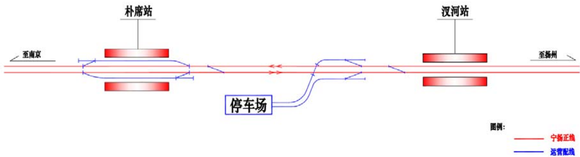
图 2.1-26 扬州停车场接轨示意图
