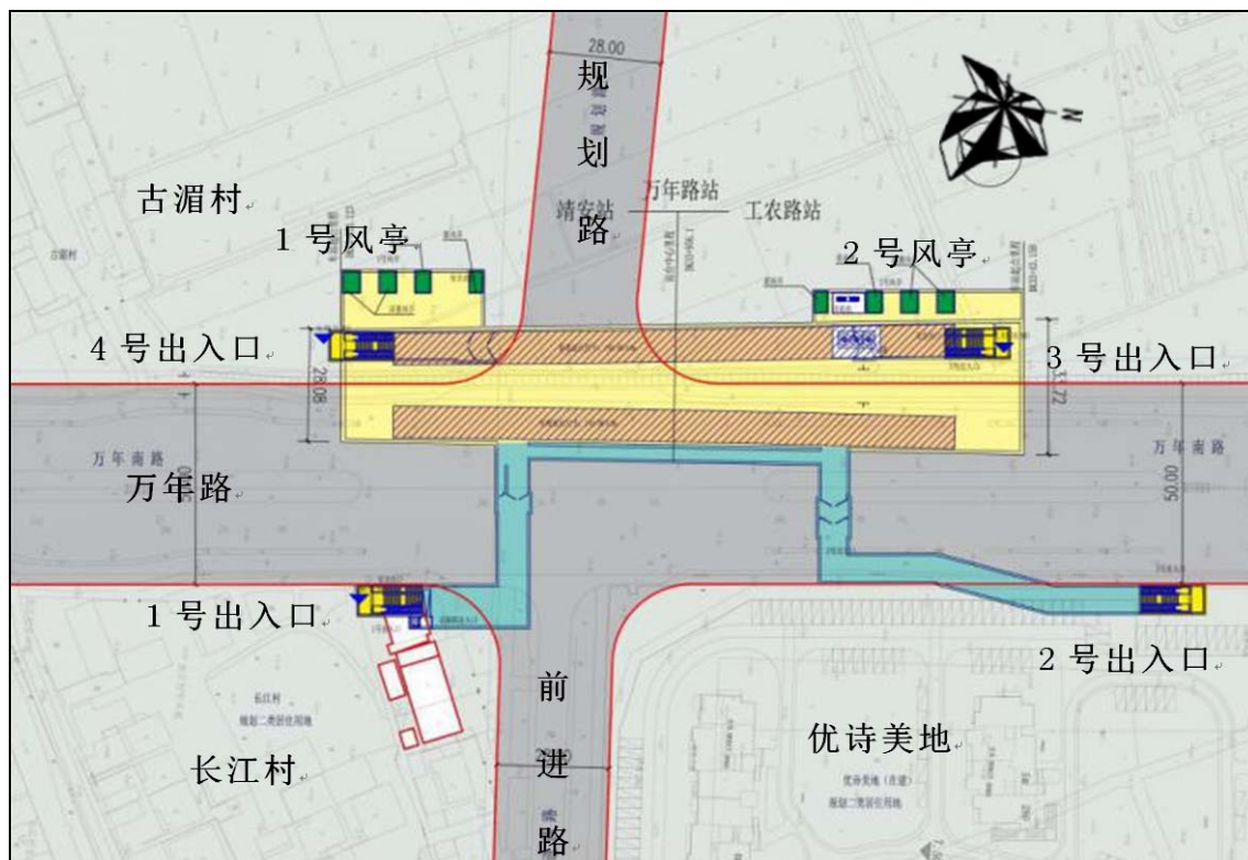
图 2.1-9 万年路站总平面布置图
