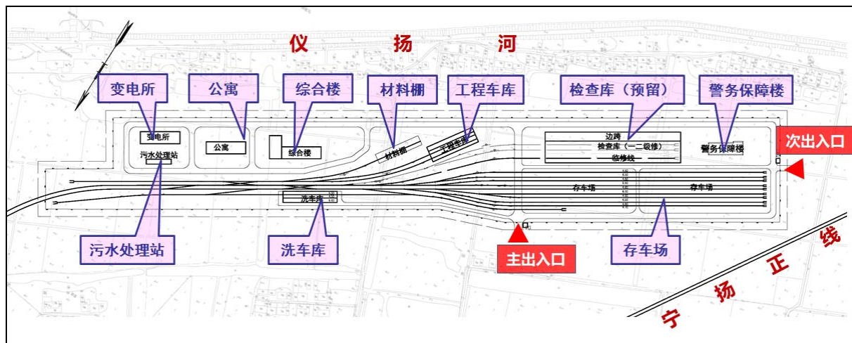
图 2.1-25 扬州停车场总平面布置图
