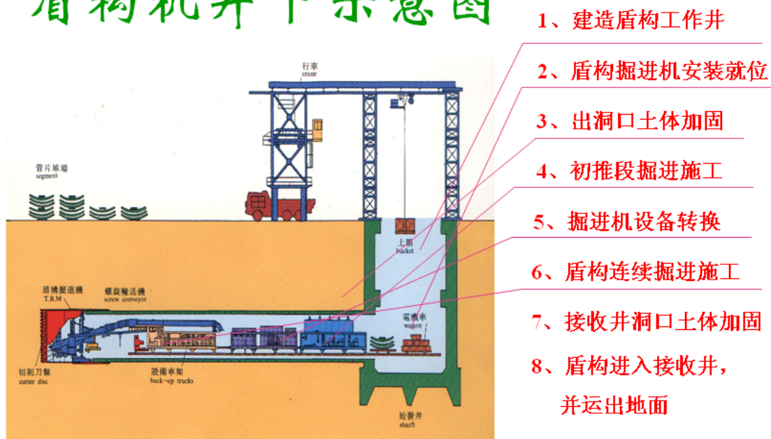
图 4.4-2 盾构法施工流程示意图
