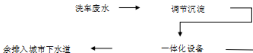
图 4.4-4 扬州停车场生产废水处理工艺图
