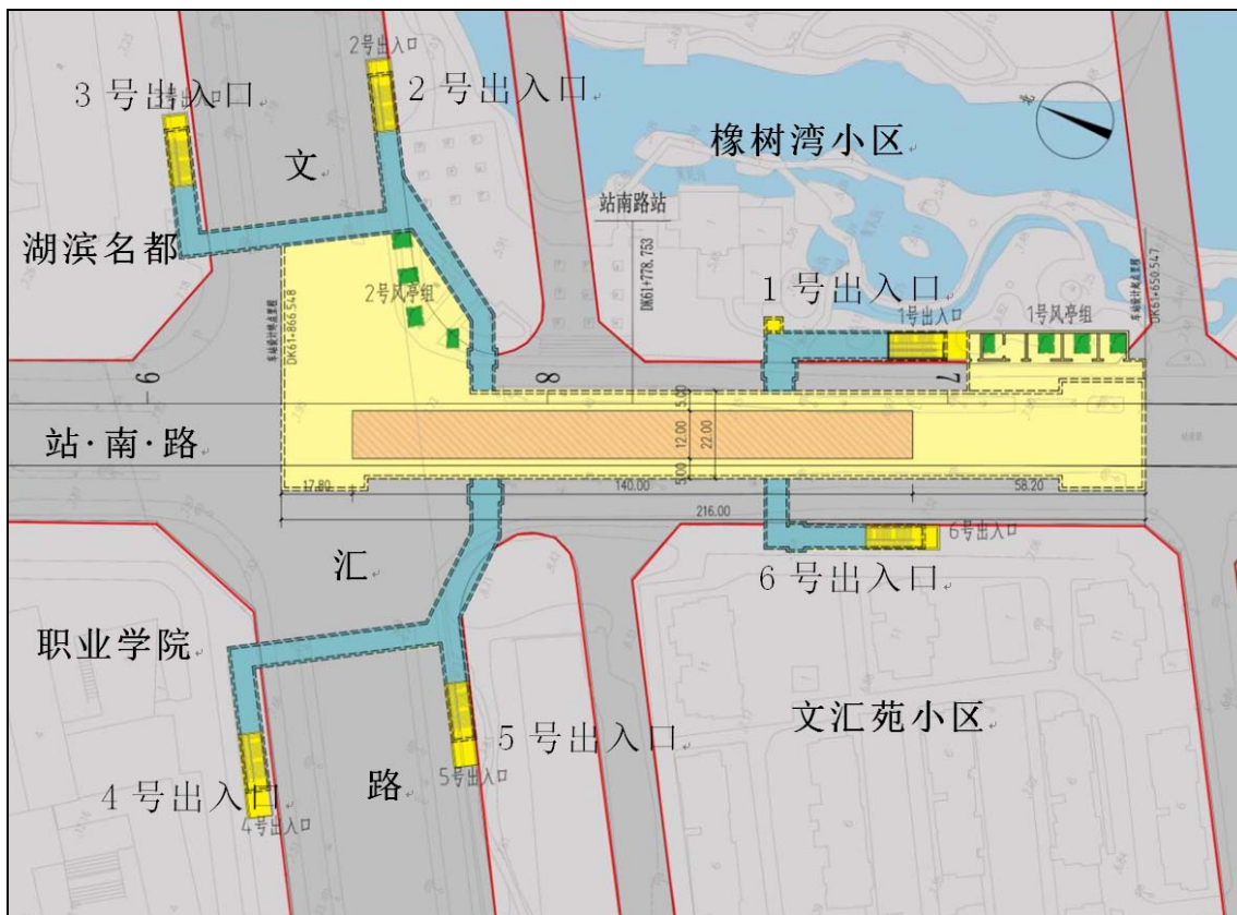
图 2.1-15 站南路站总平面布置图
