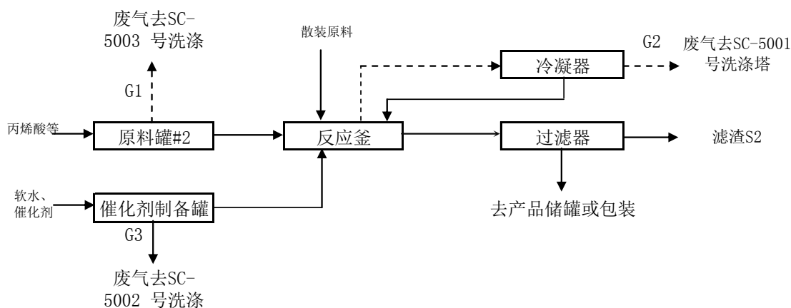
图 3.2-3 作为 C 线时的工艺流程及产污环节图
