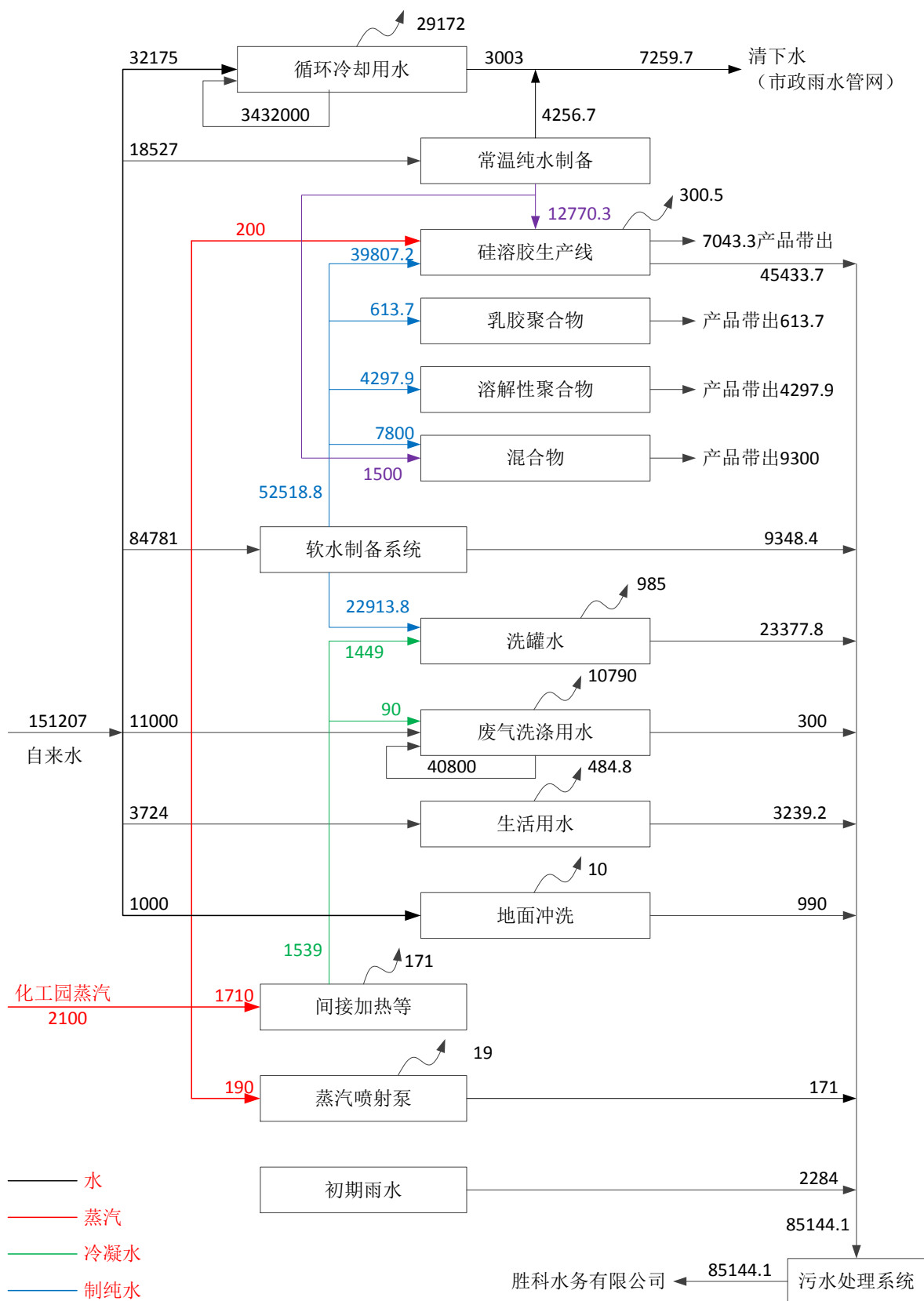
图 3.2-10 现有项目全厂水平衡图
