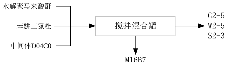
图 4.2-13 M16B7 生产工艺流程方框图
