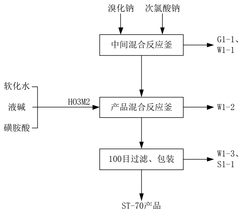
图 4.2-1 ST-70 生产工艺流程方框图
