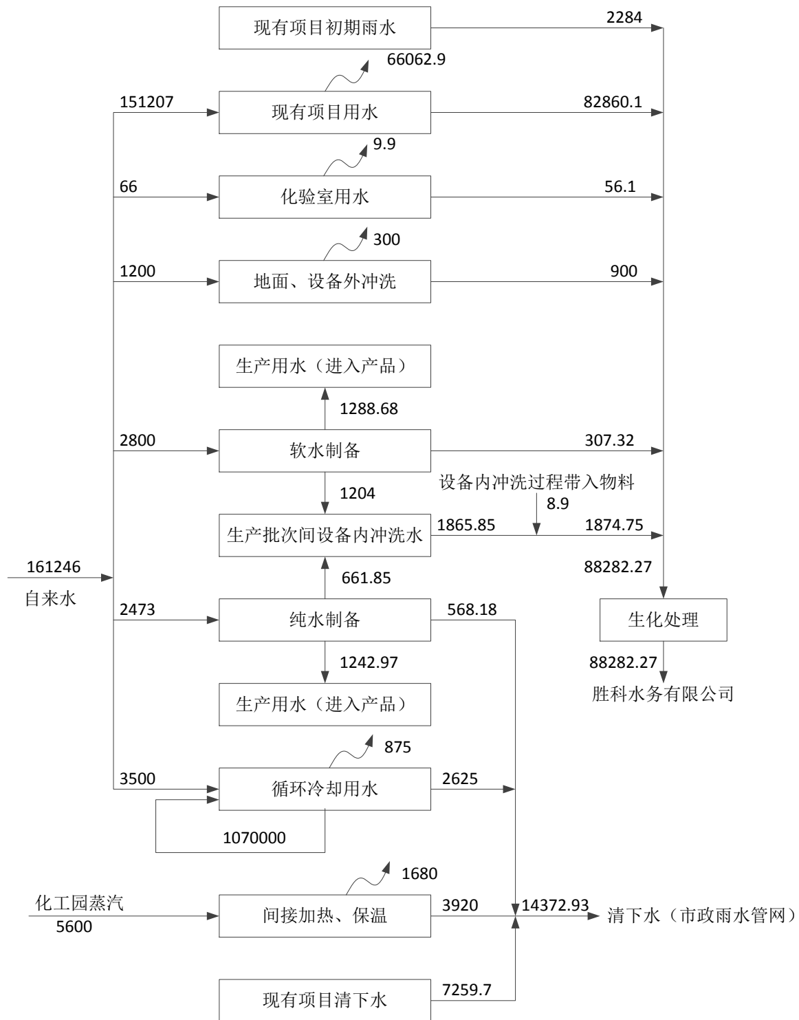
图 4.2-11 项目建成后全厂水平衡图 (t/a)
