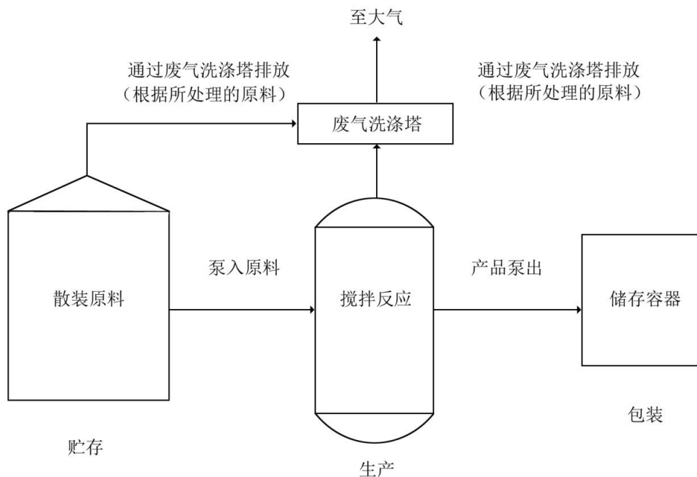
图 3.2-1 生产工艺流程及产污环节示意图
