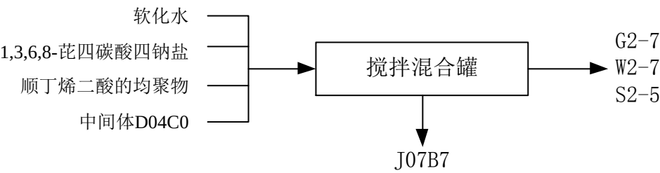
图 4.2-15 J07B7 生产工艺流程方框图
