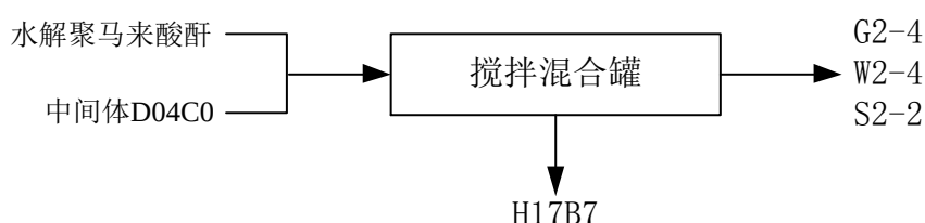
图 4.2-12 H17B7 生产工艺流程方框图
