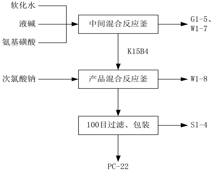
图 4.2-5 PC-22 生产工艺流程方框图
