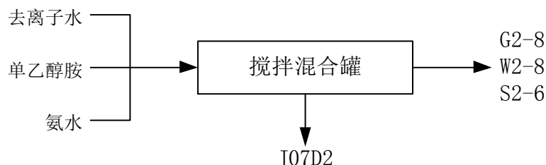
图 4.2-16 J07D2 生产工艺流程方框图
