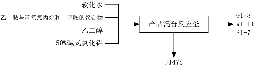
图 4.2-8 J14Y8 生产工艺流程方框图
