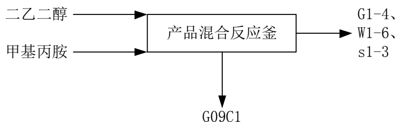
图 4.2-4 G09C1 生产工艺流程方框图
