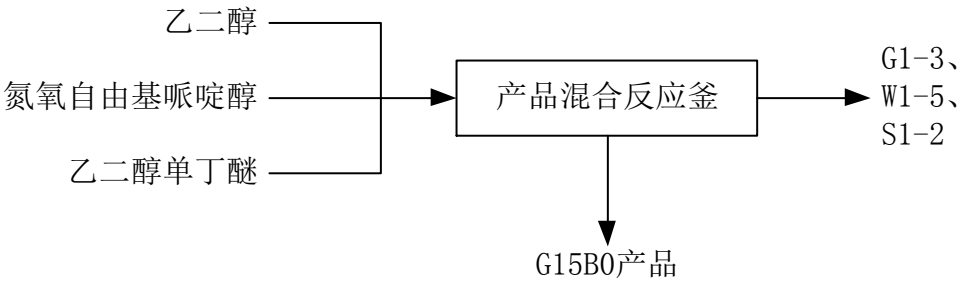
图 4.2-3 G15B0 生产工艺流程方框图
