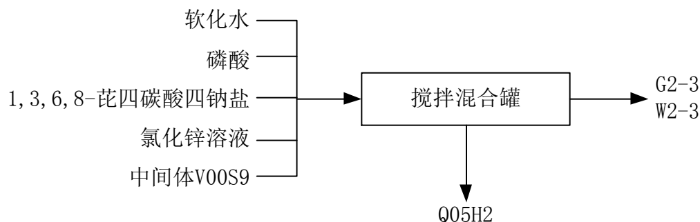
图 4.2-11 Q05H2 生产工艺流程方框图
