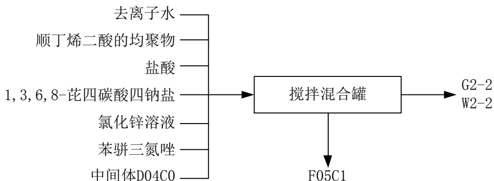
图 4.2-10 R19S4 生产工艺流程方框图
