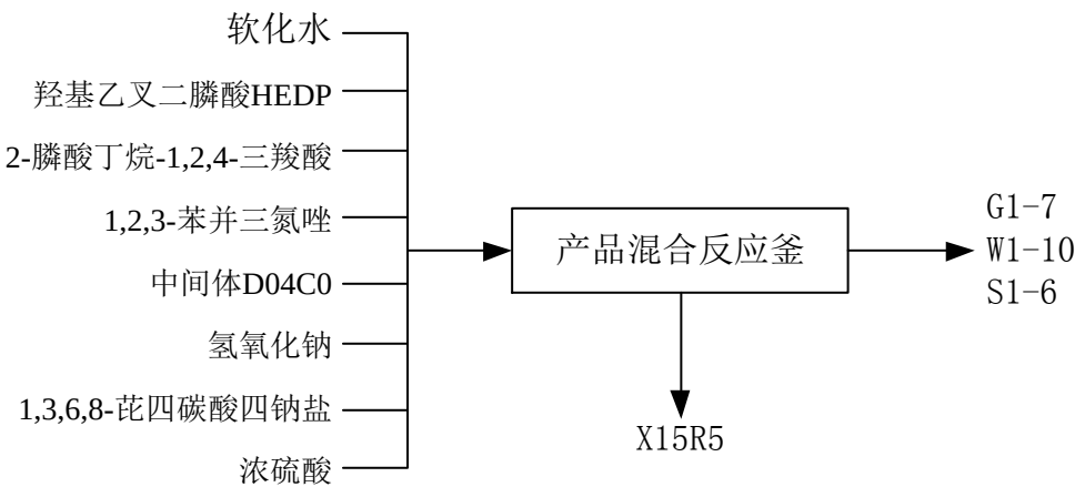
图 4.2-7 X15R5 生产工艺流程方框图
