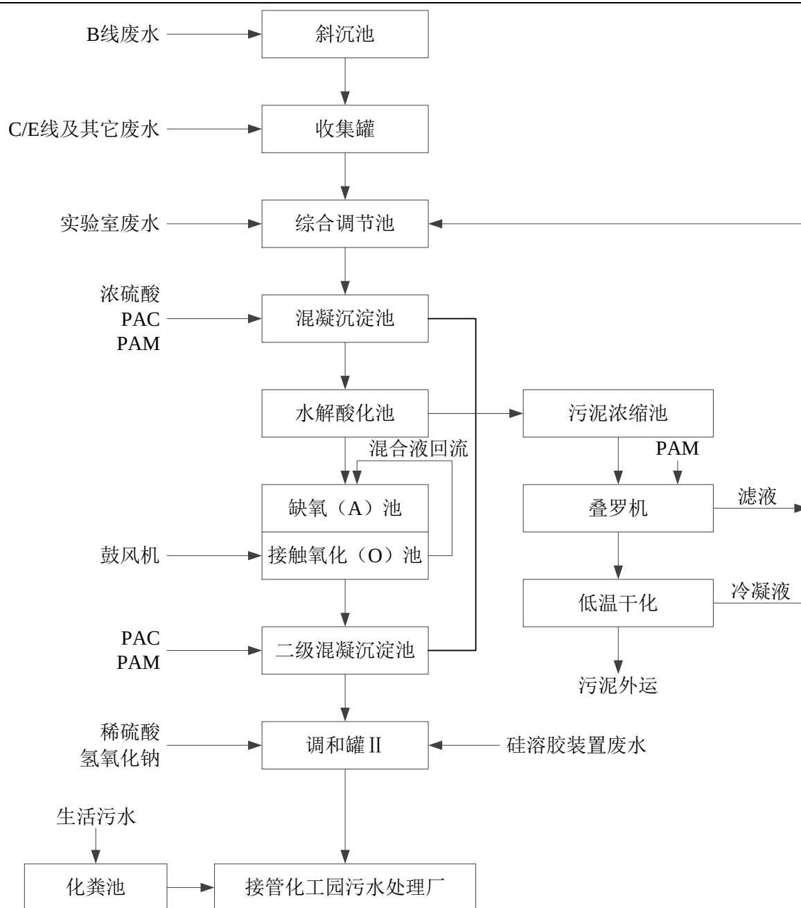
图 3.3-3 现有污水处理系统实际建设工艺流程图
