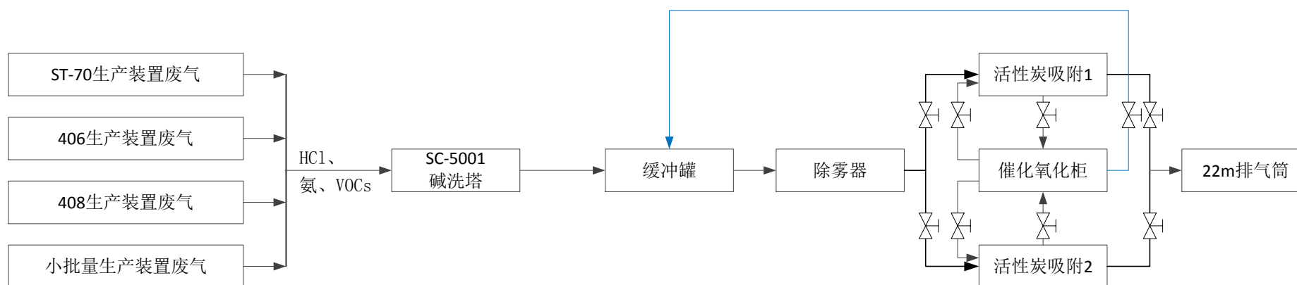
图 7.1-1 本项目生产工艺废气收集系统示意图
