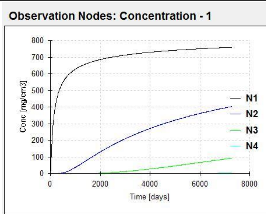
图 6.7-1 不同预测点 COD 浓度随时间变化曲线图
