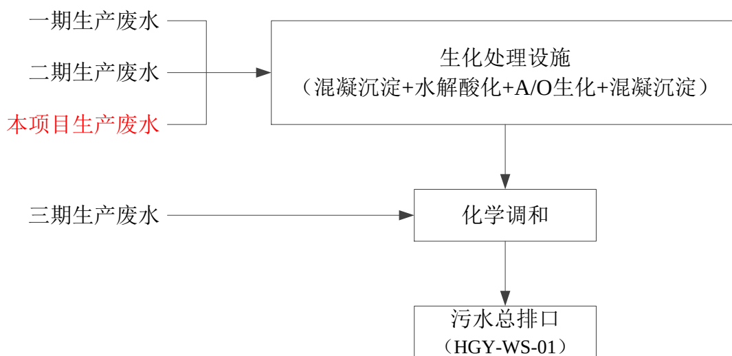
图 7.2-1 本项目废水收集走向示意图
