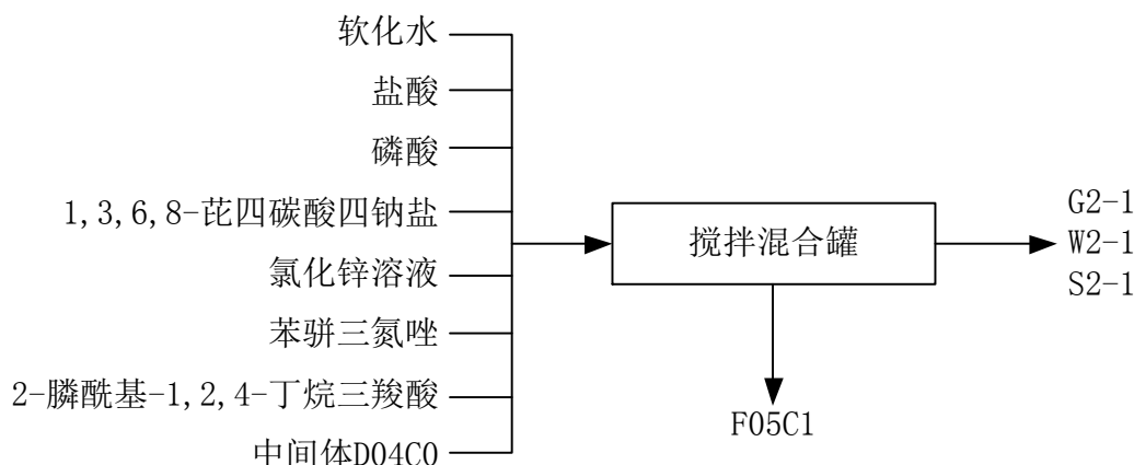
图 4.2-9 F05C1 生产工艺流程图方框图
