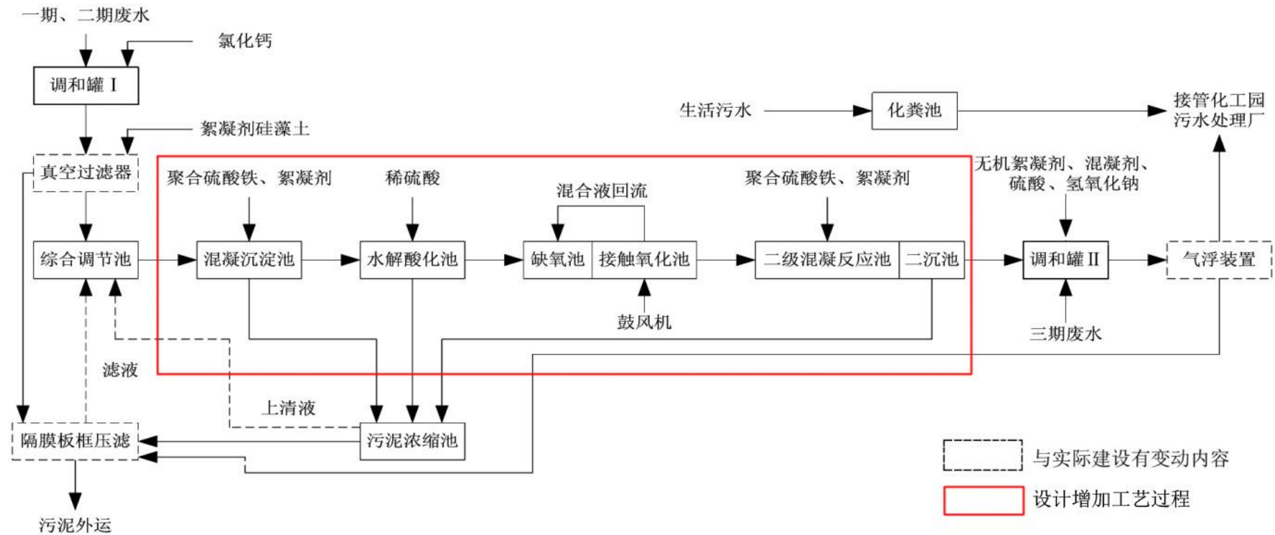
图 3.3-2 现有污水处理系统改造环评设计工艺流程图
