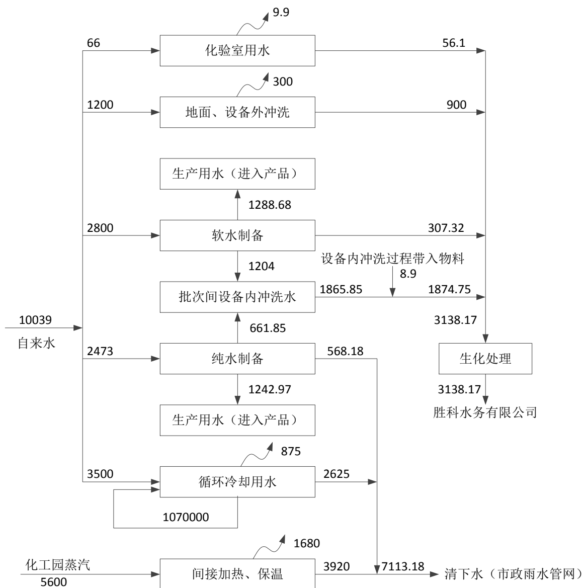
图 4.2-10 本项目水平衡图 (t/a)
