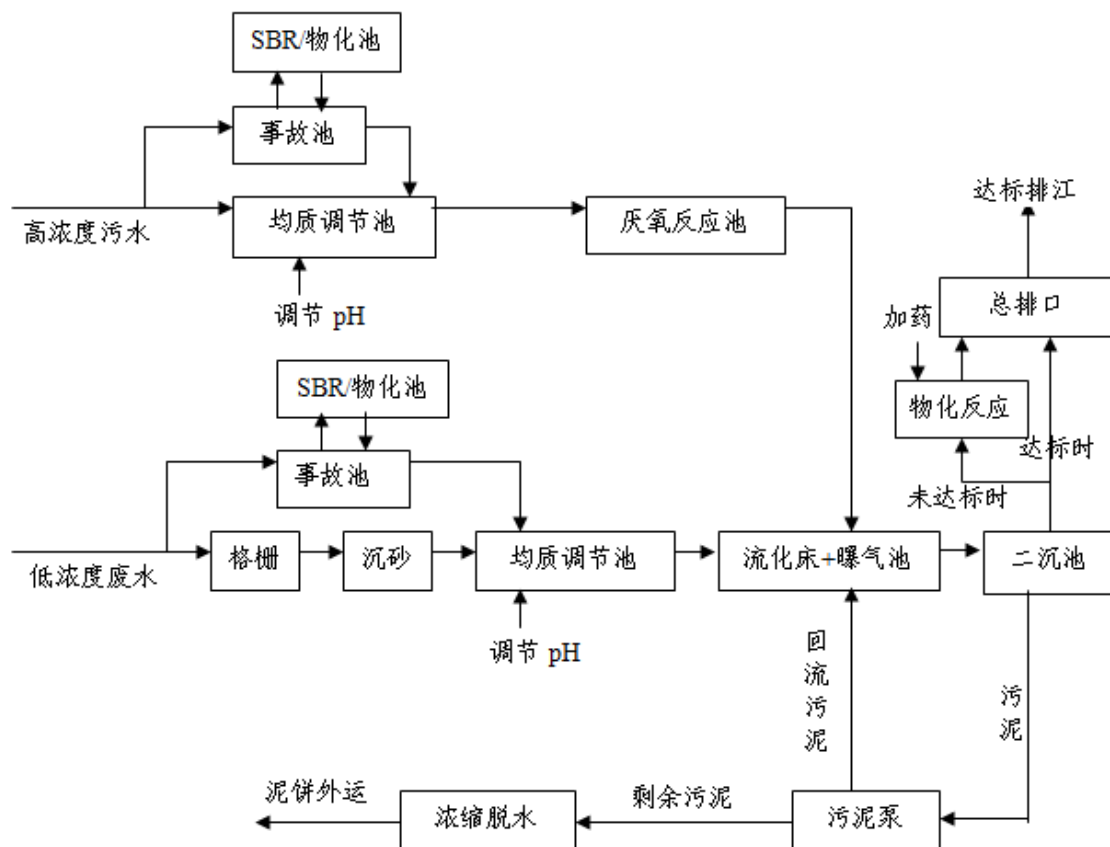
图 7.2-1 南京化学工业园污水处理厂一期工艺流程图
