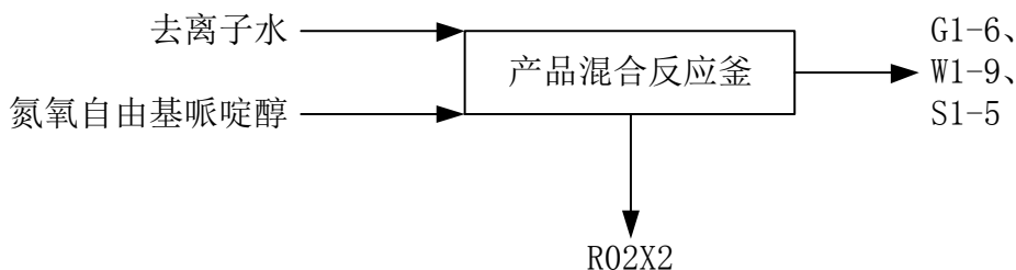
图 4.2-6 R02X2 生产工艺流程方框图
