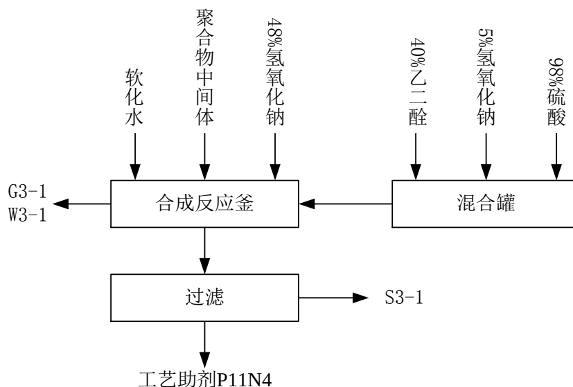
图 4.2-17 工艺助剂 P11N4 生产工艺流程方框图
