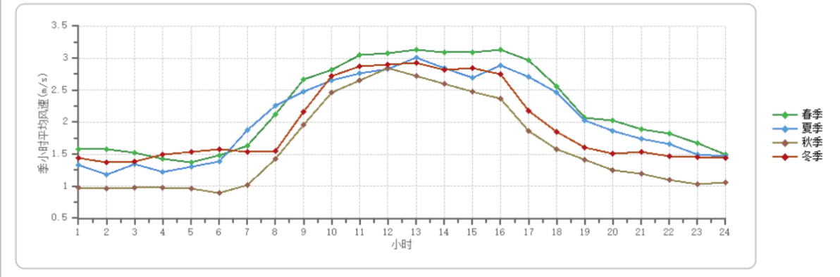
图 6.1-3 季小时平均风速的日变化曲线
