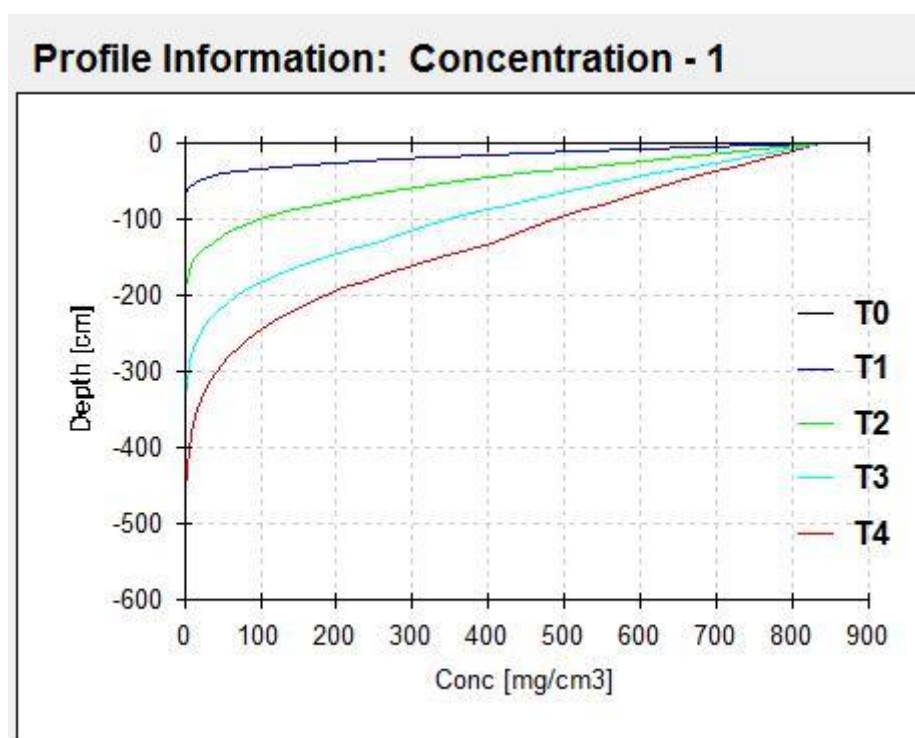
图 6.7-2 不同预测时间 COD 浓度随深度变化曲线图
