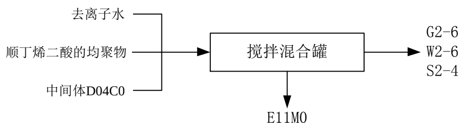
图 4.2-14 E11M0 生产工艺流程方框图
