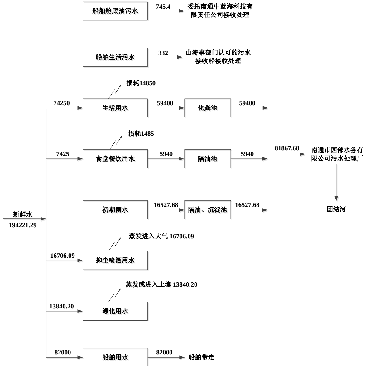
图 3.4-7 建设项目水平衡图 (t/a)
