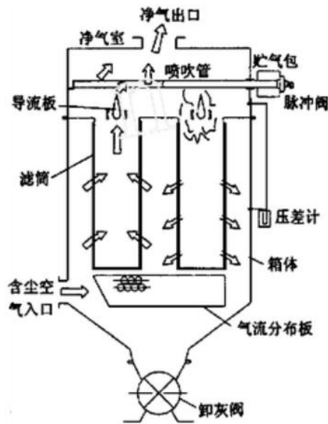
图 6.1-3 滤筒式除尘器构造示意图
