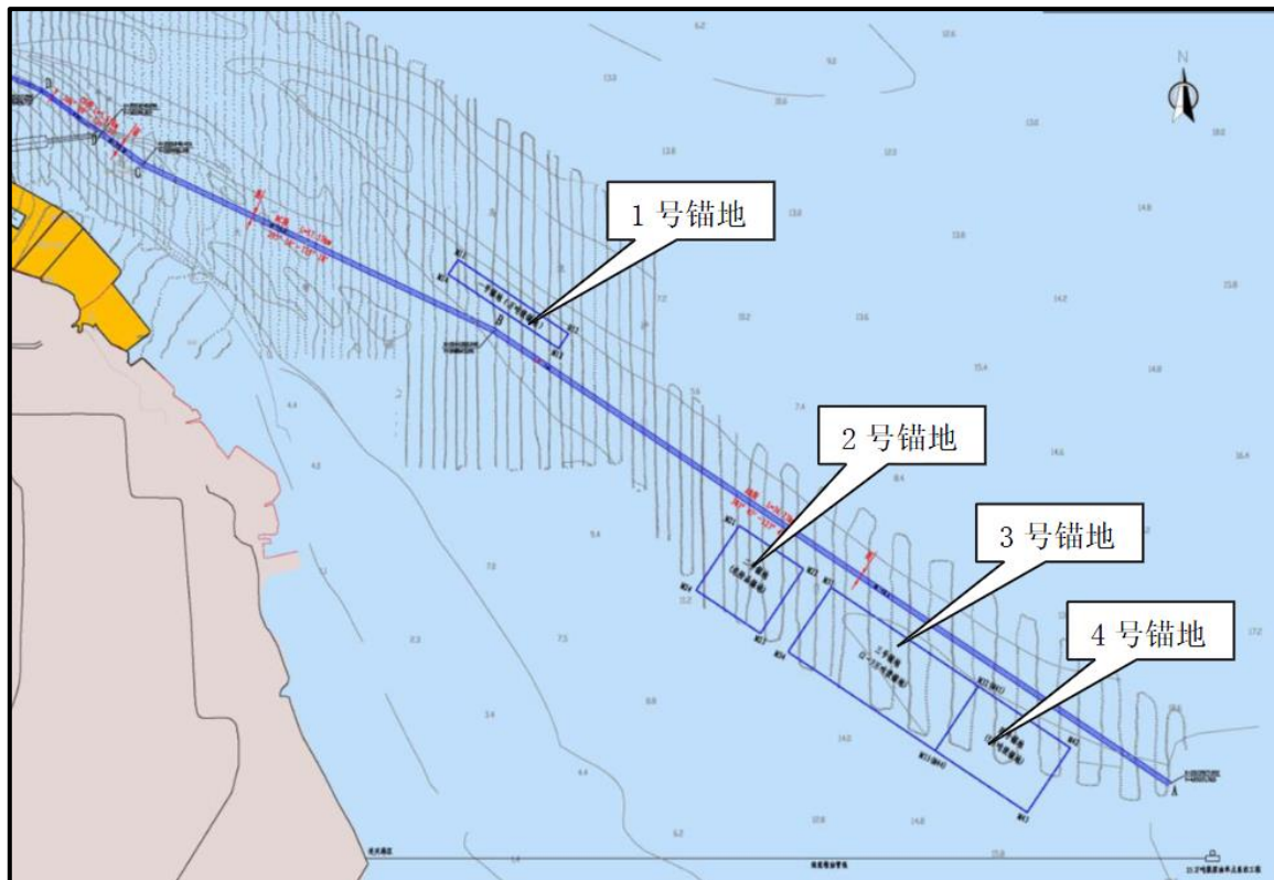
图 3.1-10 锚地布置示意图
