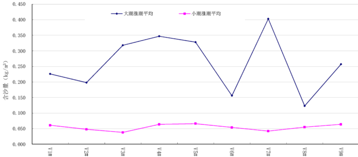
图 4.4-7 (2) 各垂线涨潮期潮平均含沙量分布图
