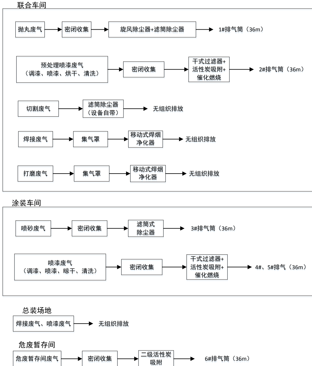
图 6.1-1 本项目废气收集、治理流向图
