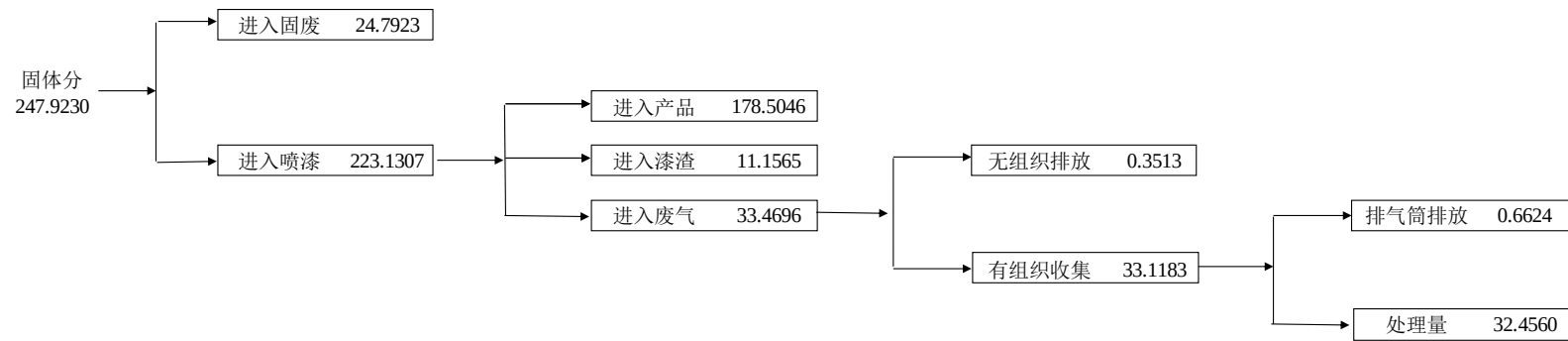
图 3.4-6 固体份平衡图
