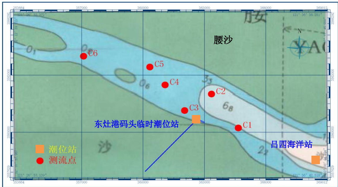
图 5.7-10 (b) 潮位站及水文泥沙测点位置示意图 (2014 年 9 月)
