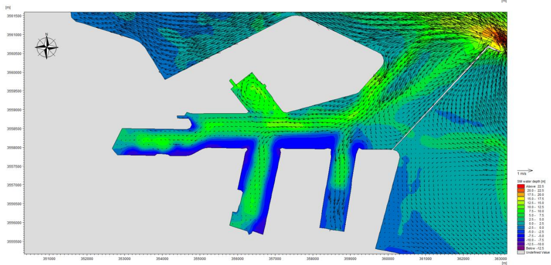
图 5.7-16 项目后海域大潮涨急流场图
