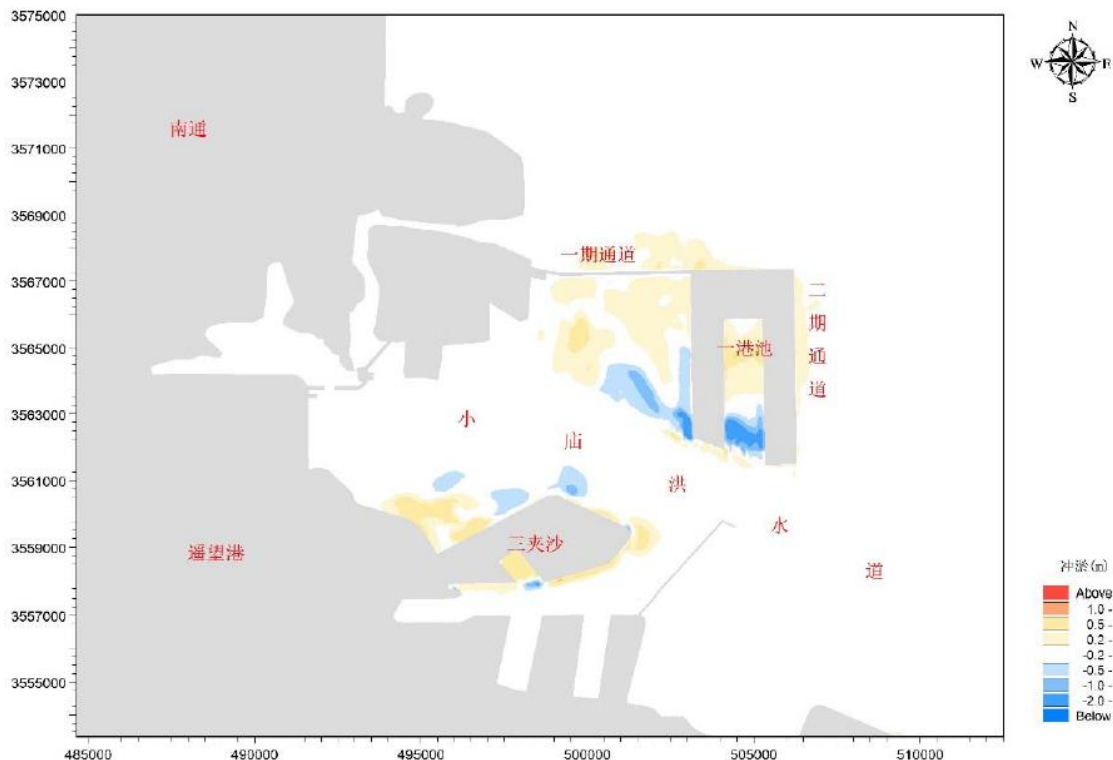
图 5.8-2 围填海工程实施后周边水域泥沙年冲淤强度分布图 (m/a) (模拟)
