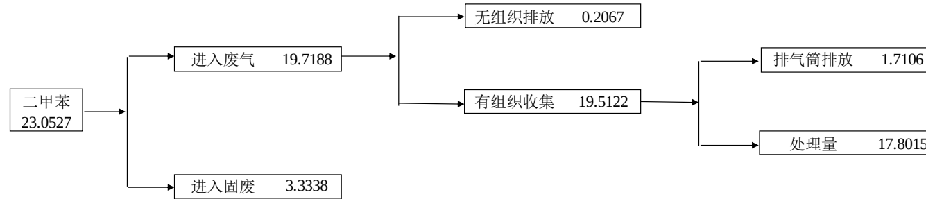
图 3.4-4 二甲苯物料平衡图
