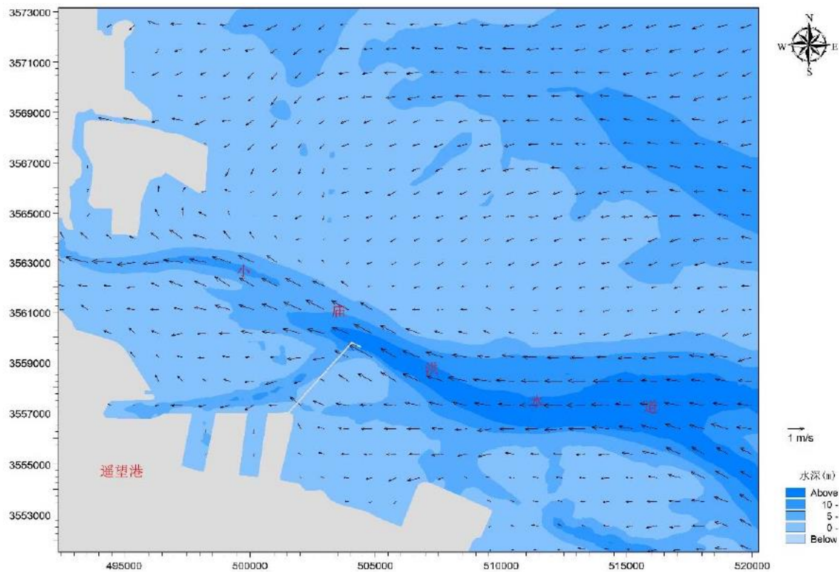
图 5.7-1 围填海工程前大潮涨急流场图
