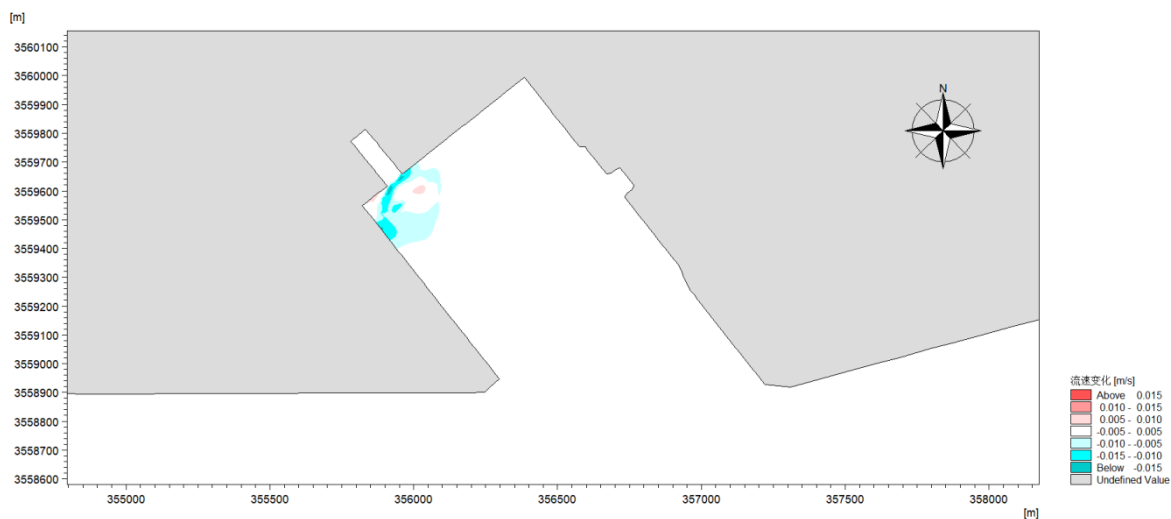
图 5.7-19 项目后大潮落急流速变化图
