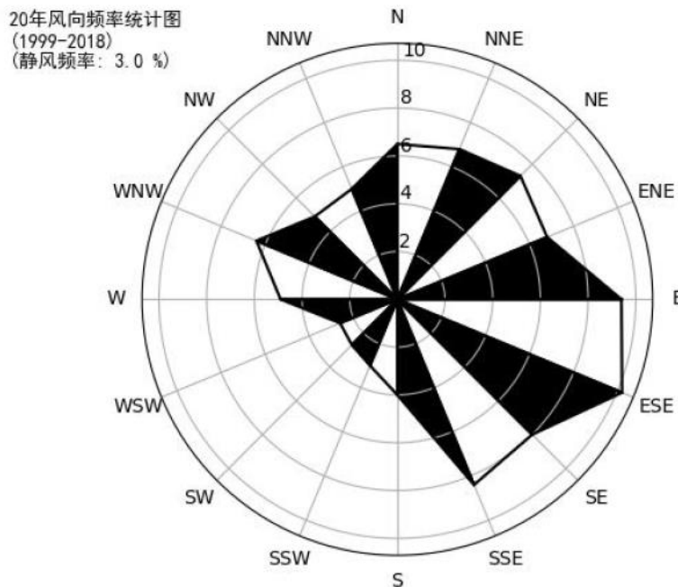
图 4.1-1 吕泗风向玫瑰图 (静风频率 3.0%)
