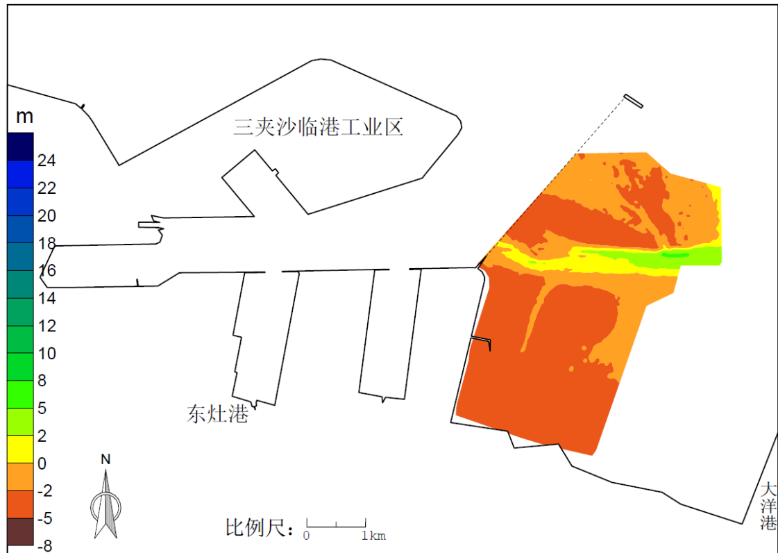
图 4.5-15 2018 年水下地形图
