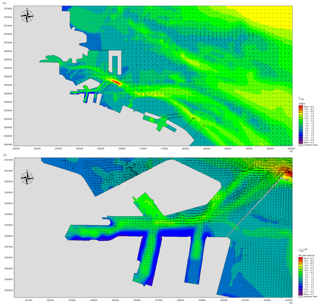
图 5.7-17 项目后海域大潮落急流场图
