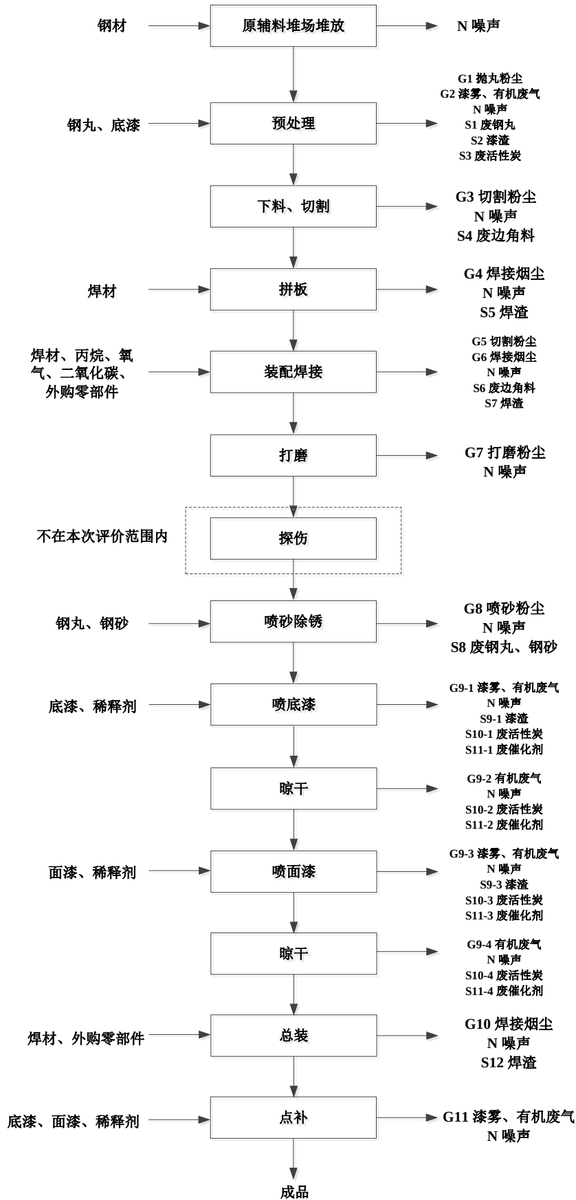
图 3.2-1 本项目生产工艺流程图（风电设备、海工智能模块、特种钢结构）
