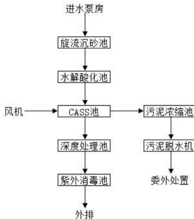
图 6.1-5 南通市西部水务有限公司污水处理工艺流程图
