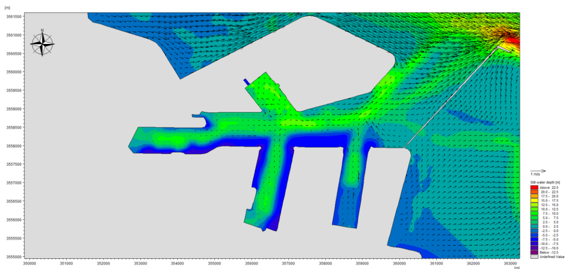
图 5.7-15 项目前海域大潮落急流场图
