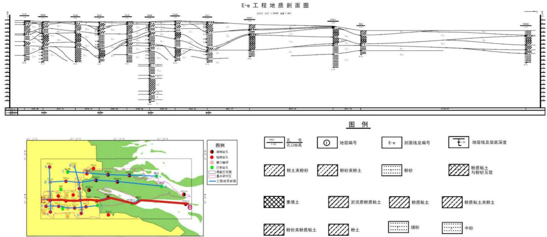
图 4.1-5 工程地质剖面图 (Ee)
