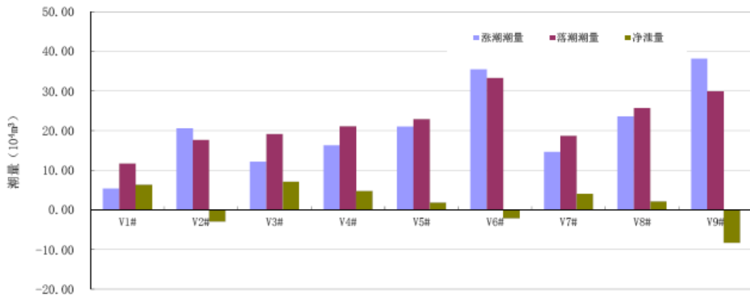
图 4.4-6 (2) 各垂线小潮单宽涨、落潮潮量柱状图
