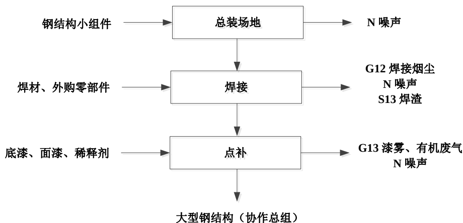
图 3.2-2 本项目生产工艺流程图（大型钢结构（协作总组））
