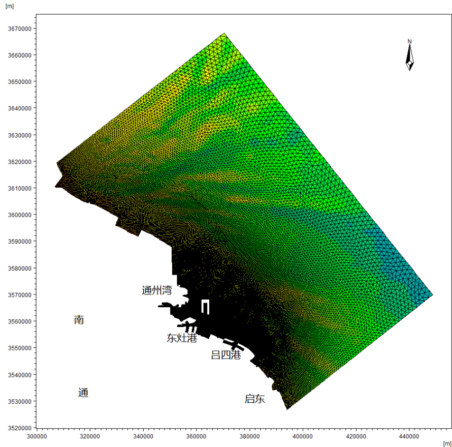
图 5.7-9 模型计算网格
