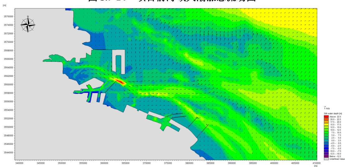
图 5.7-14 项目前海域大潮涨急流场图
