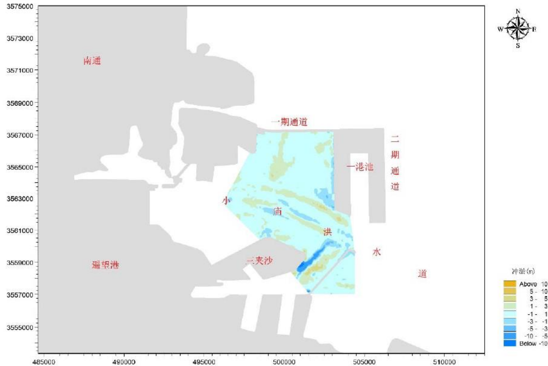
图 5.8-1 2014 年至 2018 年间海床冲淤图（实测）
