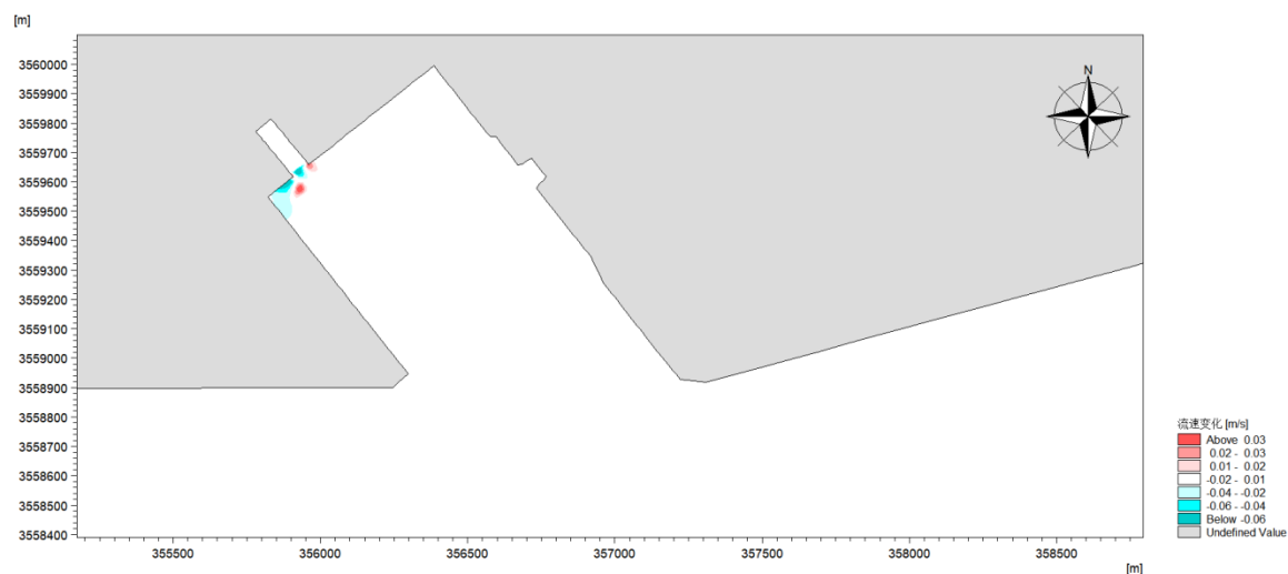
图 5.7-18 项目后大潮涨急流速变化图
