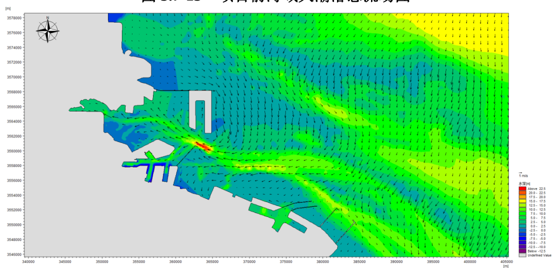
图 5.7-15 项目前海域大潮落急流场图
