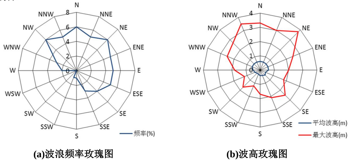
图 4.1-4 吕四海洋站波浪玫瑰图（1969 年～2001 年）
