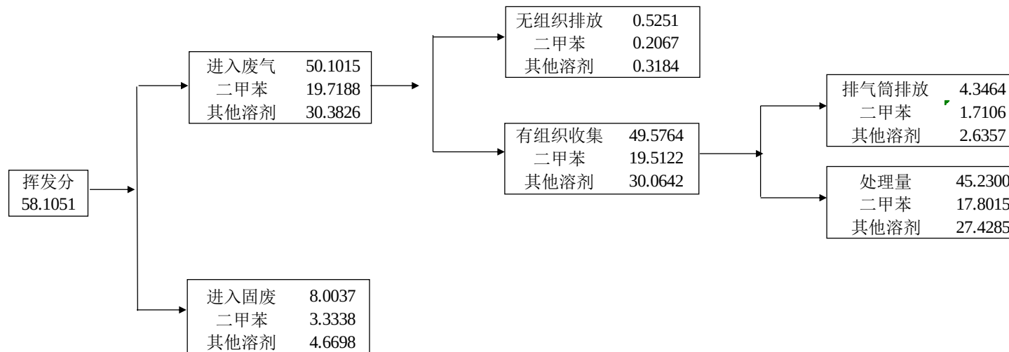
图 3.4-5 VOCs 平衡图
