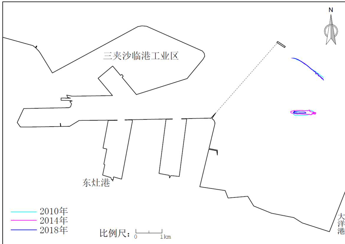
图 4.5-18 2010 年、2014 年、2018 年 5 米等深线变化图
