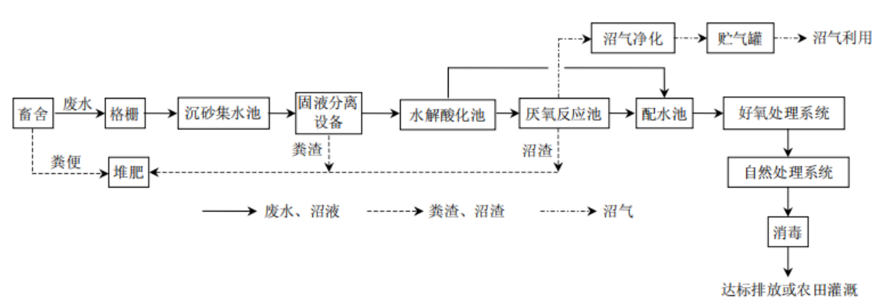
图 6.2-4 模式III工艺基本流程图
