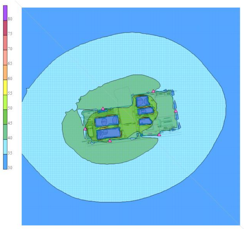
图 5.2-2 噪声贡献值等声值线图（单位：dB(A)）
