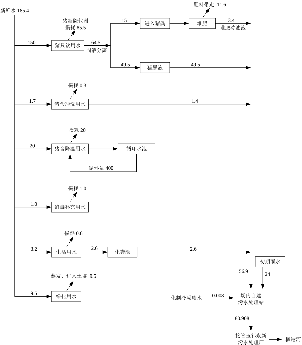
图 3.4-2 夏季水量平衡图 (单位: m³/d)
