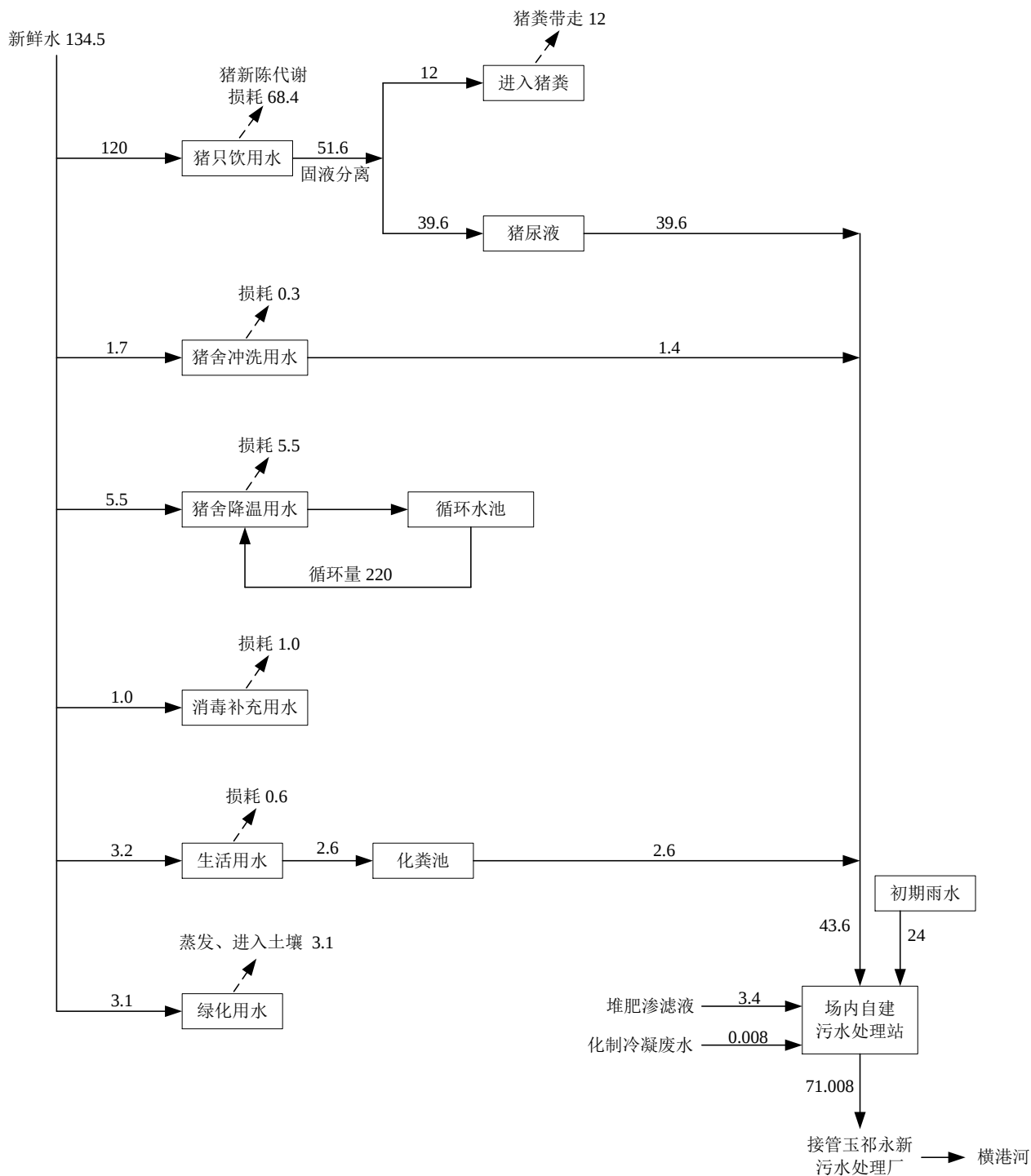
图 3.4-1 全年平均（春秋季节）水量平衡图（单位： \text{m}^3/\text{d} ）
