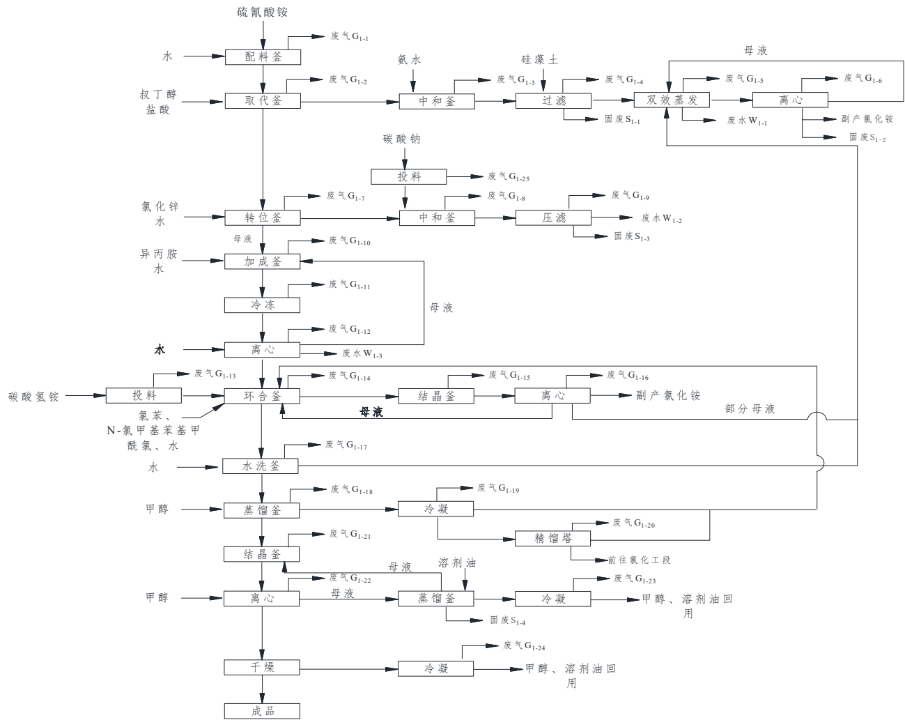
图 2.1-1 扑虱灵生产工艺流程及产污环节图
